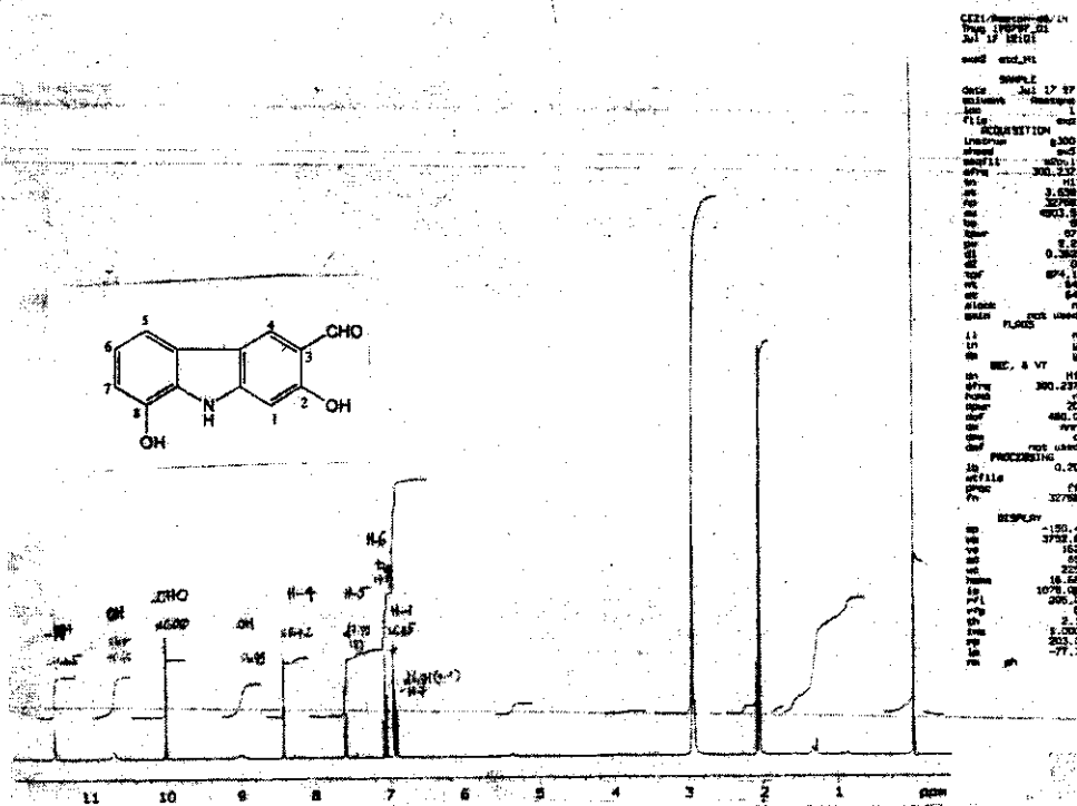
Hình 1. Phổ ^1\text{H} -NMR của clauszolin-M (300 MHz, acetone- \text{d}_6 )
