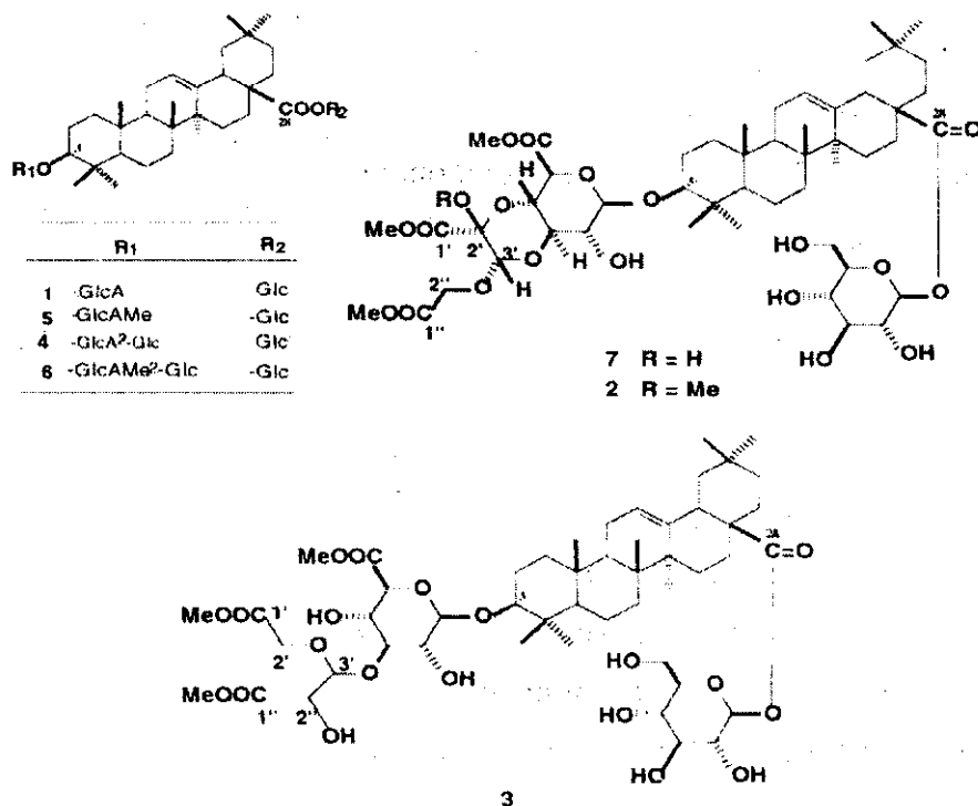
Hình 1. Cấu trúc các saponin G (1), H (2), I (3) và J (4) và các saponin liên hệ phân lập từ rễ cỏ xước.
