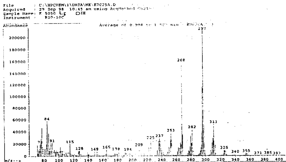
Hình 2. Phổ khối lượng của L 5
