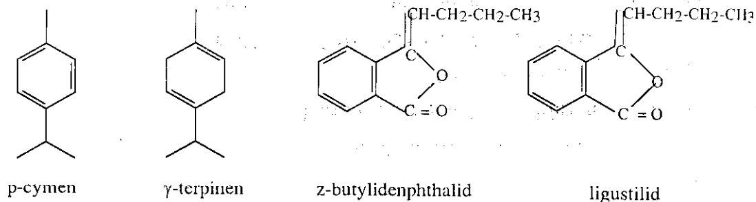
Hình 1: Cấu trúc hoá học của một số thành phần chính của tinh dầu lá đương quy Nhật Bản trồng tại Thái Nguyên. [1, 2, 6]
