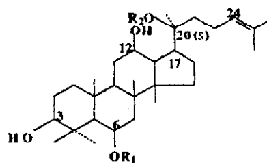
Saponin nhóm protopanaxatriol
