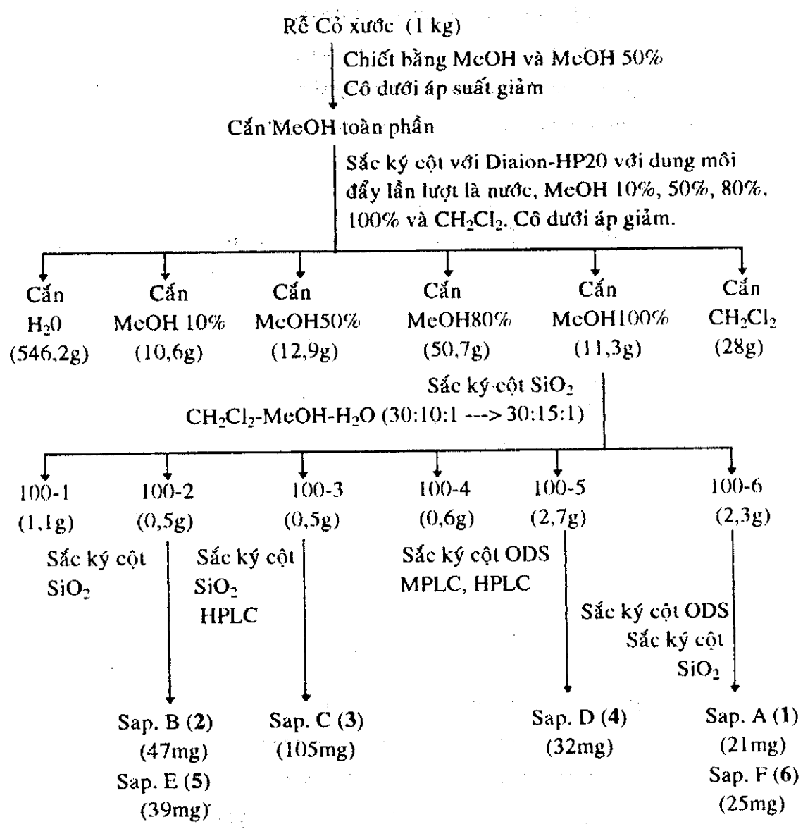
Hình 2. Sơ đồ chiết xuất và phân lập các saponin A-F từ rễ cỏ xước
