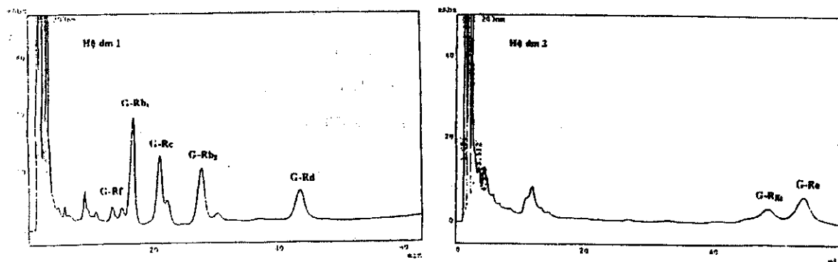
Hình 5: Sắc đồ HPLC của mẫu "BHT" ( Panax ginseng C.A. Meyer).
