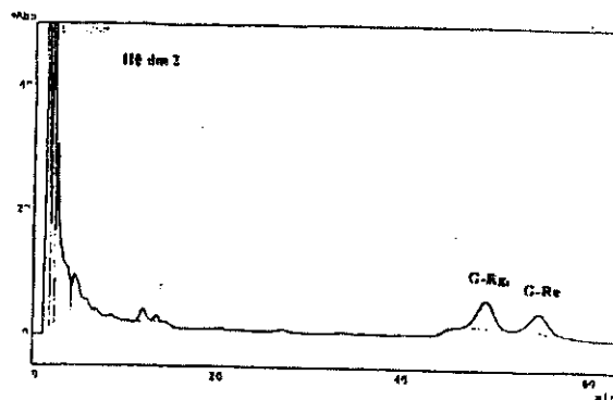
Hình 3: Sắc đồ HPLC của mẫu "HS2" ( Panax ginseng C.A. Meyer).
