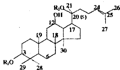
Saponin nhóm protopanaxadiol
