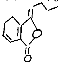
Ligustilid (theo Zhang Shi-Yu và Cheng Kuo Chang, 1989).
