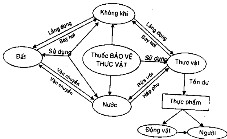
Hình 2: Sơ đồ chuyển hóa thuốc BVTV trong môi trường
