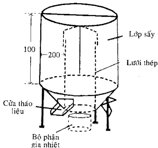
Hình 3.4: Thiết bị sấy thủ công SH-200 (Viện công nghệ sau thu hoạch)
