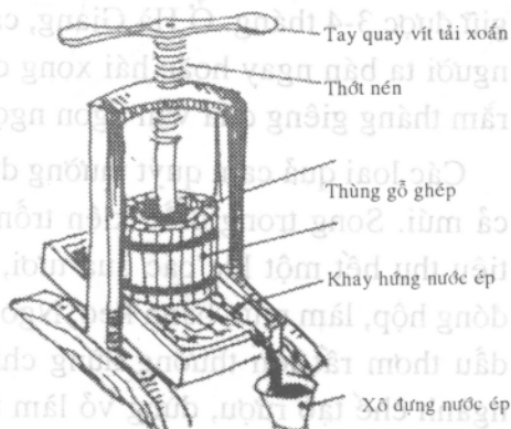
Hình 4.3: Máy ép thủ công
