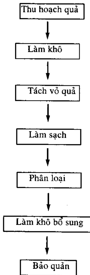
Hình 3.3: Quy trình công nghệ xử lý đậu, đỗ, lạc sau thu hoạch
