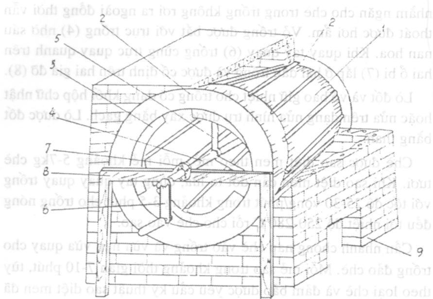
Hình 1.2: Trống sạ chè quay tay
