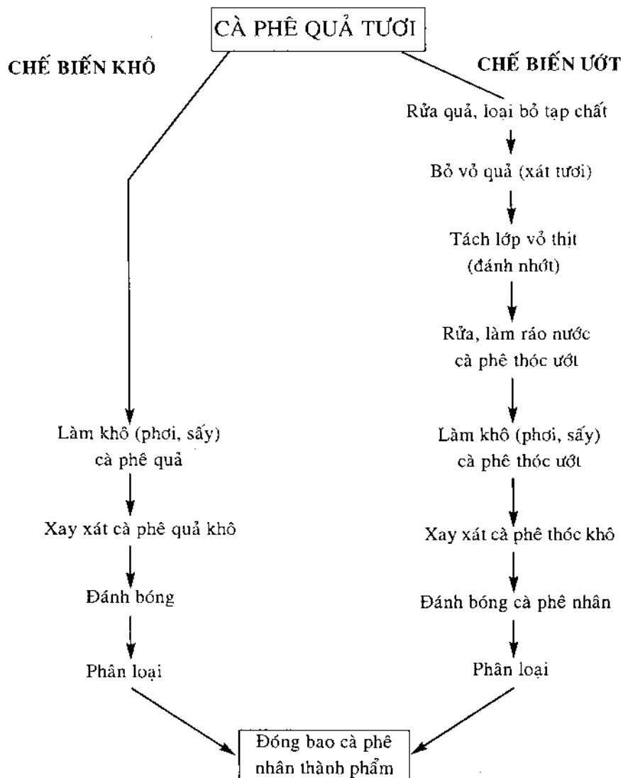
Hình 2.1: Sơ đồ công nghệ chế biến cà phê
