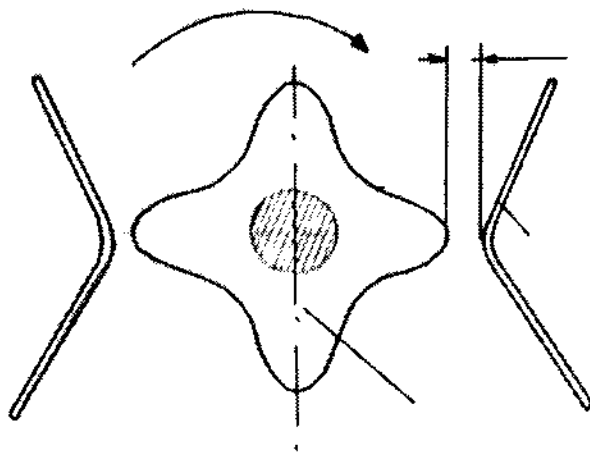
Hình 2.4: Điều chỉnh độ rộng hẹp khe hở giữa trục phân phối và tấm giăng.
