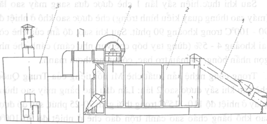
Hình 1.1: Máy sấy chè S-300
