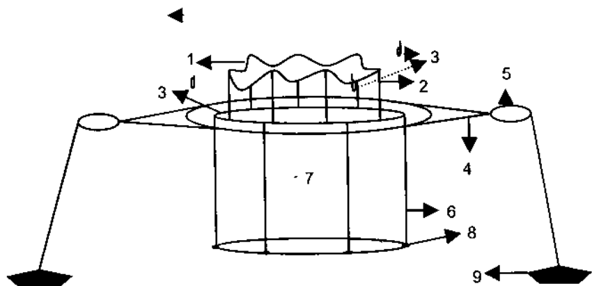
Lồng nuôi cá hình tròn (kiểu Naui)
