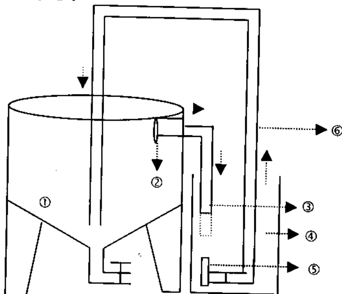
Hệ thống bể ương tuần hoàn
