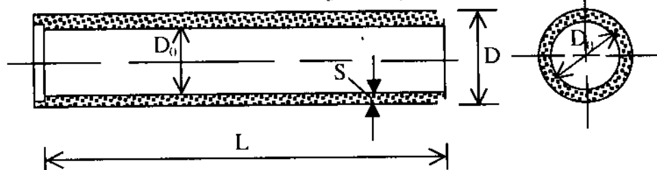
Hình 2.7: Ống bê tông
