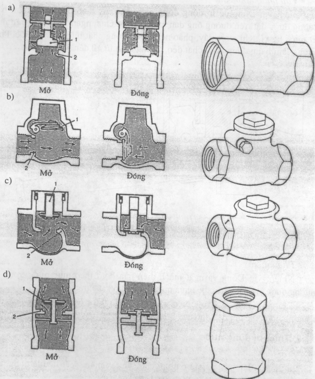
Hình 5.11: Van 1 chiều
