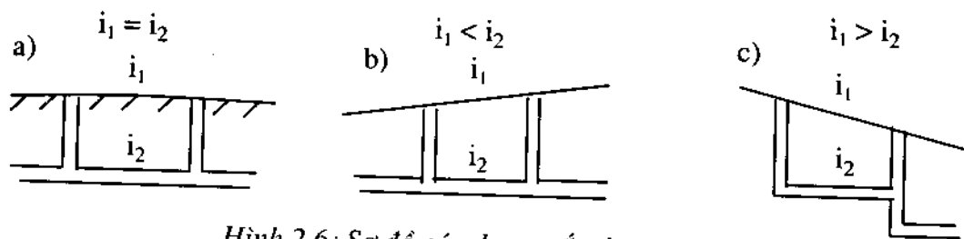
Hình 2.6: Sơ đồ các dạng trắc dọc mạng lưới i_1 - Độ dốc mặt đất; i_2 - Độ dốc đáy cống.
