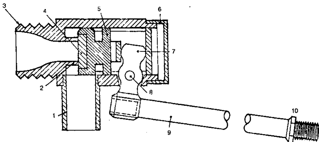
Hình 5.12: Van phao
