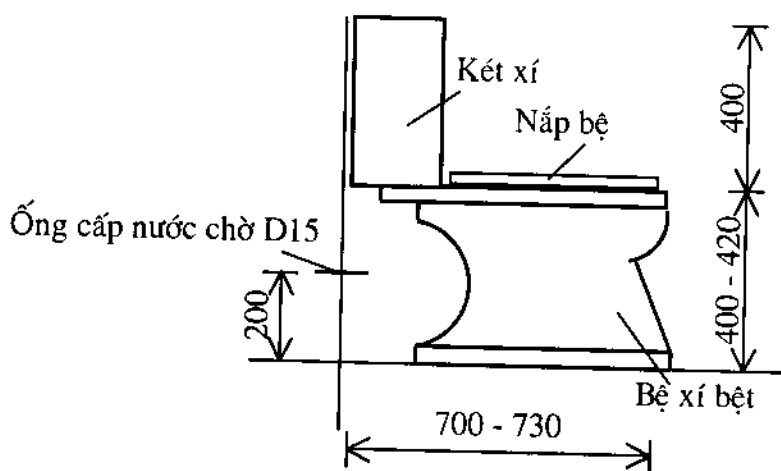
Hình 4.1: Bệ xí ngồi bệt
