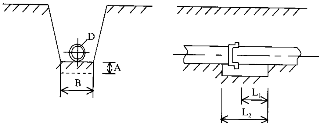
Hình 2.3: Kích thước mương và hố xấp
