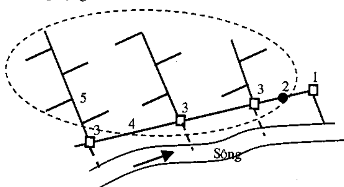
Hình 1.1: Sơ đồ hệ thống thoát nước chung
