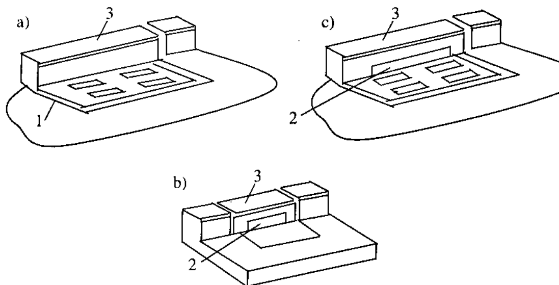
Hình 2.12: Các kiểu cửa thu nước mưa
