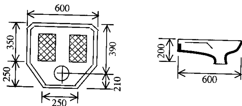
Hình 4.2: Bệ xí ngồi xổm
