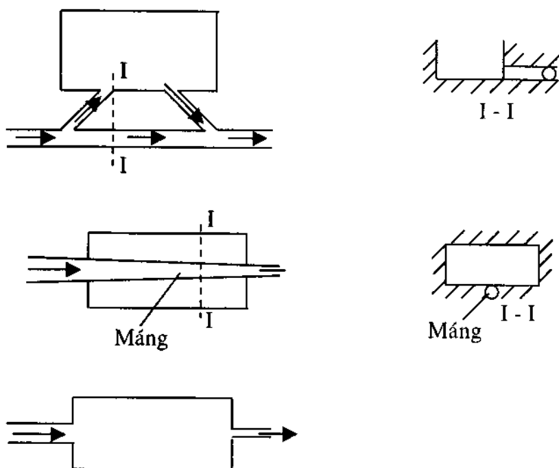
Hình 2.13: Sơ đồ khái quát của hồ điều hoà
