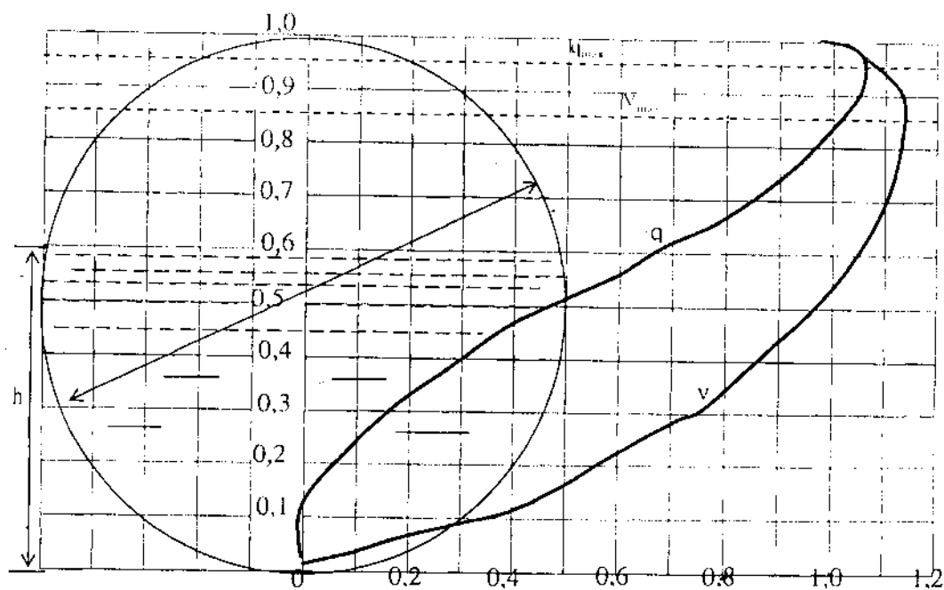
Hình 4.7: Biểu đồ h/D
