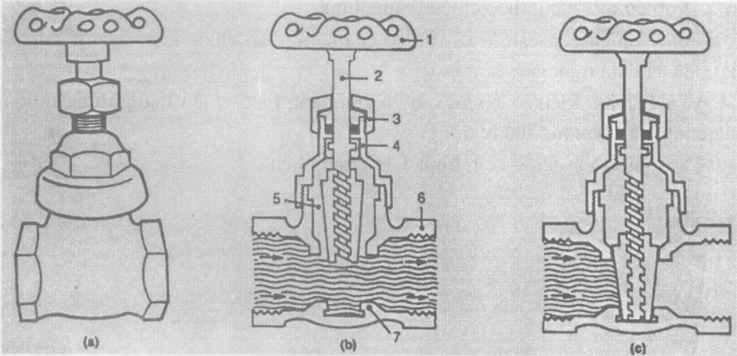
Hình 5.10: Van trực chìm
