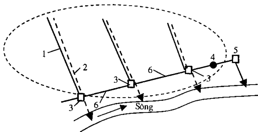
Hình 1.3: Sơ đồ hệ thống thoát nước nửa riêng
