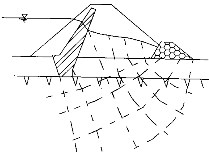
Hình 1- 25. Biểu đồ mặt cắt dòng thấm
