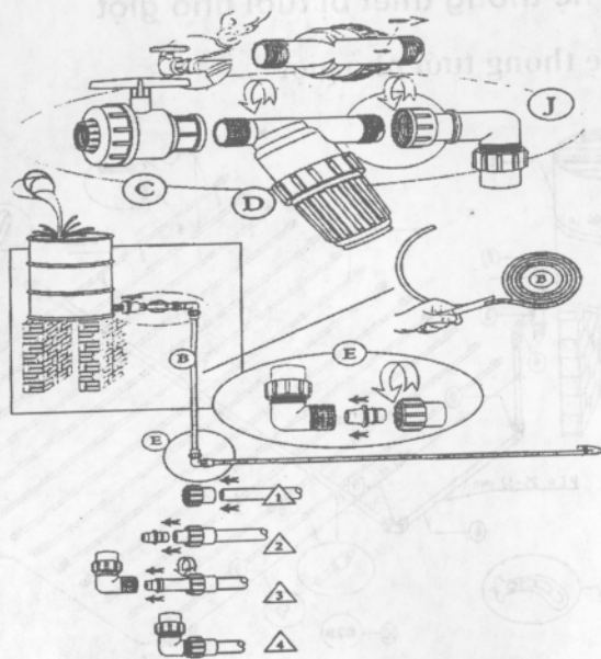
Hình 2-7. Các phụ kiện
