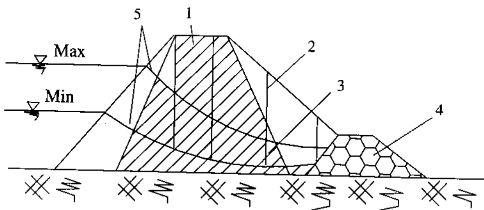
Hình 1-7. Đập có tường tâm
