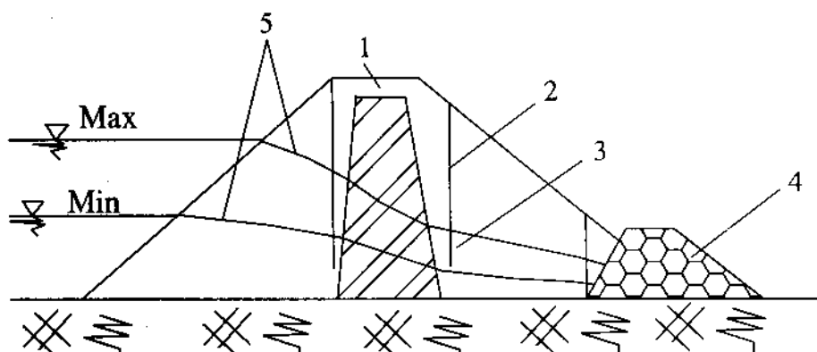
Hình 1-8. Đập có tường tâm tương đối rộng
