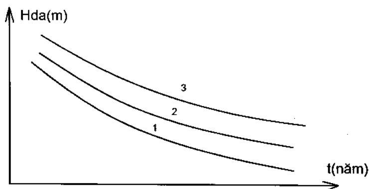
Hình 1 - 23. Đường quá trình mực nước đo áp
