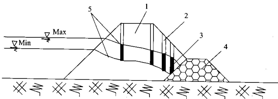
Hình 1-5. Đập đồng chất có tầng lọc ngược
