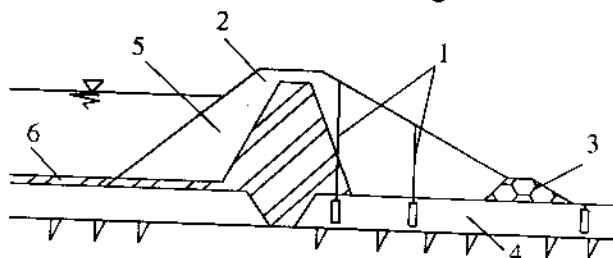
Hình 1 - 16. Sơ đồ bố trí ống đo áp của nền đá cát sỏi có tường ngăn thấm bằng đất sét
