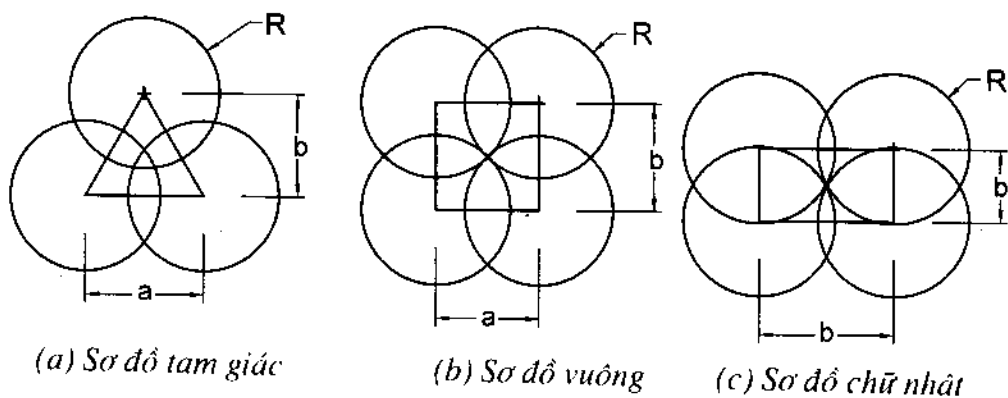
Hình 2-3. Các sơ đồ bố trí vòi phun mưa
