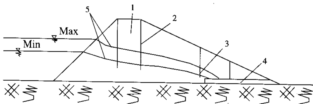
Hình 1-5. Đập đồng chất có tầng lọc ngược
