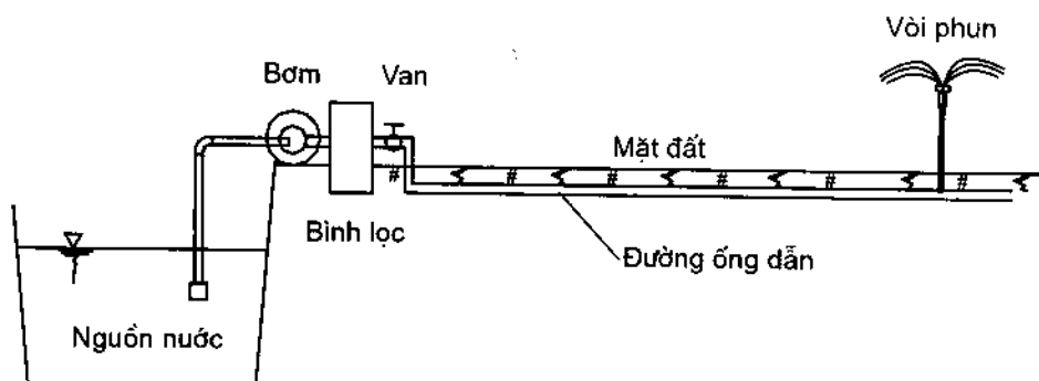
Hình 2-1. Sơ đồ đơn giản hệ thống tưới phun
