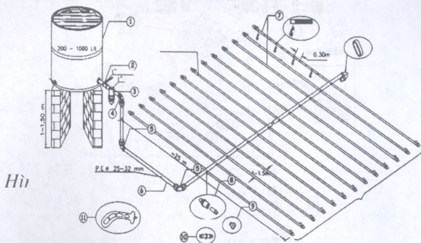
Hình 2-5. Sơ đồ đơn giản hệ thống tưới nhỏ giọt cỡ nhỏ dùng bình chứa có áp
