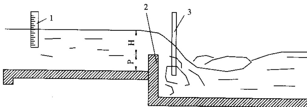
Hình 1 - 13. Sơ đồ kết cấu máng đo nước hình chữ nhật có thu hẹp bên
