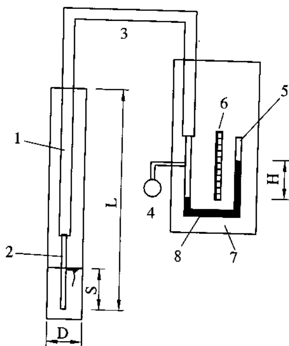
Hình 1 - 12. Cấu tạo ống đo áp kiểu áp khí hình chữ U
