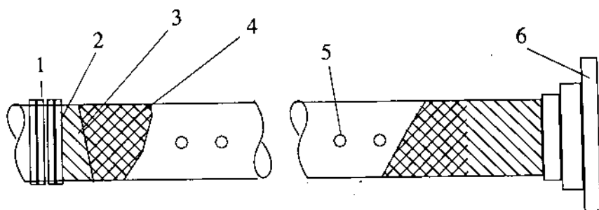
Hình 1-11. Đoạn ngấm nước tầng lọc
