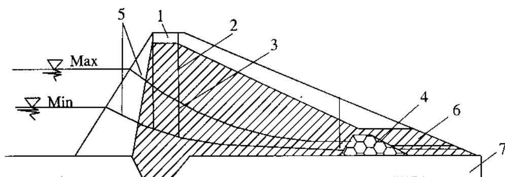
Hình 1-8. Đập có tường tâm tương đối rộng
