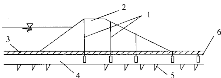
Hình 1-19. Sơ đồ bố trí ống đo áp nền đập thấm nước kết cấu 2 lớp.
