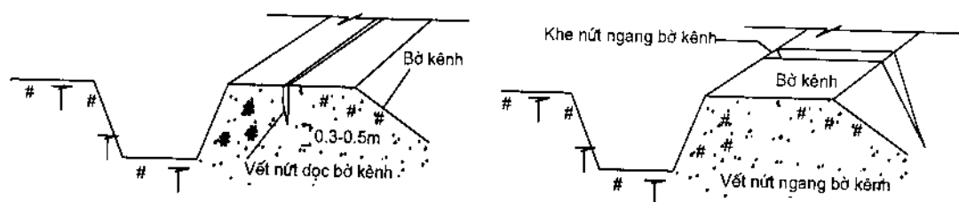
Hình 1-2. Xử lý khe nứt ở bờ kênh
