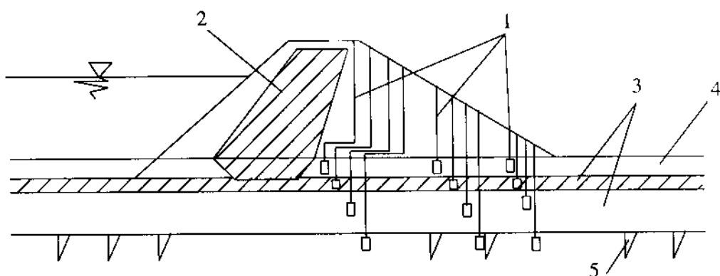
Hình 1-20. Sơ đồ bố trí ống đo áp nền đập thấm nước kết cấu nhiều tầng
