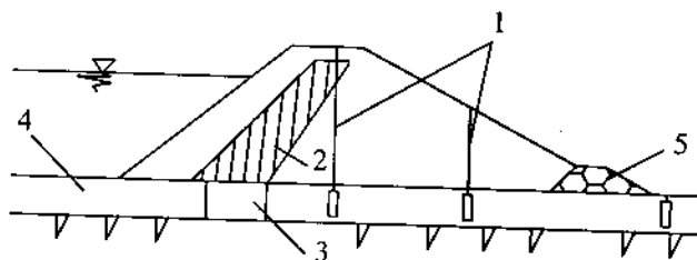
Hình 1 - 17. Sơ đồ bố trí ống đo áp của nền đá cát sỏi của đập có tường nghiêng chống thấm bằng bê tông hoặc bằng đất sét.
