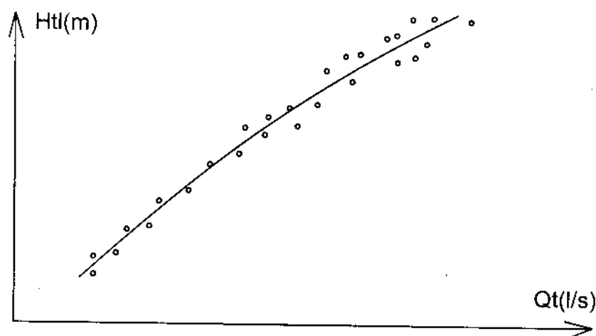
Hình 1-22. Quan hệ giữa lưu lượng thấm và mực nước thượng lưu
