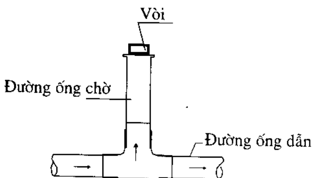
Hình 2-2. Chi tiết vị trí vòi phun
