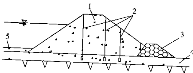
Hình 1-15. Sơ đồ bố trí ống đo áp của nền đá cát sỏi phòng thấm nằm ngang (1) Thân đập; (2) Ống đo áp; (3) Thiết bị thoát nước; (4) Tầng đá cát, sỏi; (5) Lớp phủ.
