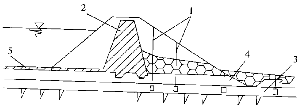
Hình 1-21. Sơ đồ bố trí ống đo áp của nền đập đất có phủ trọng lực
