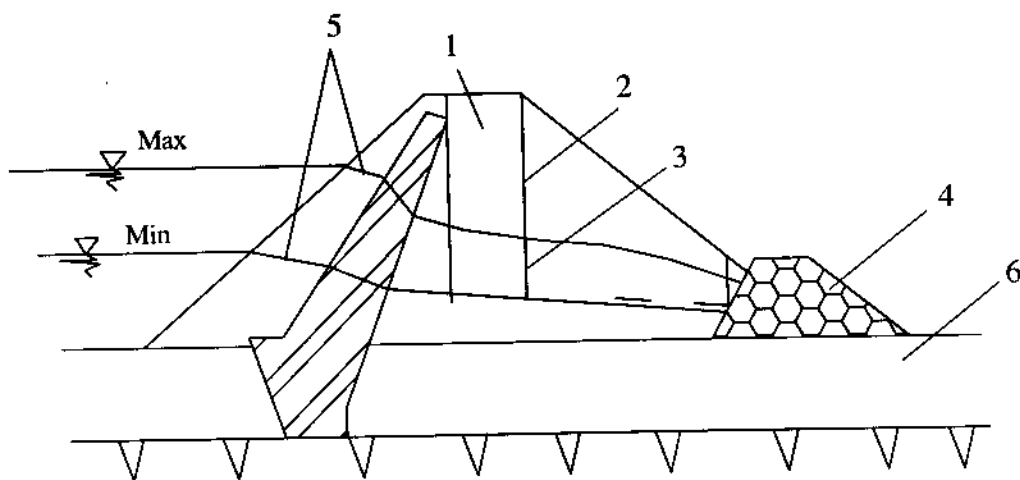
Hình 1-10. Đập có tường nghiêng mềm
