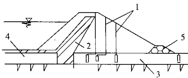
Hình 1-18. Sơ đồ bố trí ống đo áp của nền đá cát sỏi của đập có tường nghiêng chân khay chống thấm
