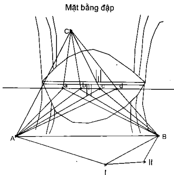
Hình 1- 4. Phương pháp quan trắc theo lưới tam giác
