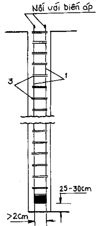
Hình 4 - 5. Điện trở trong lỗ nệm thẳng đứng
