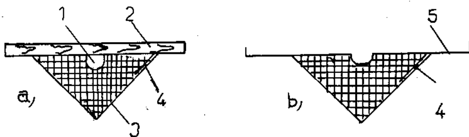
Hình 4.4 Nệm bitum đúc sẵn
