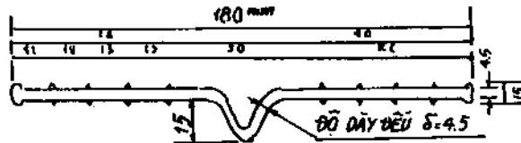
H-1 - Hình dạng và kích thước vật chắn nước PVC (chất dẻo) VCN- KN92.
