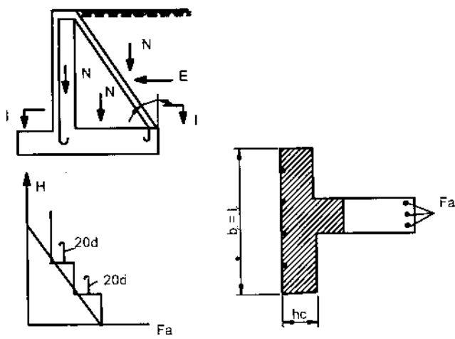
Hình 4-28 Sơ đồ tính toán sườn chống
