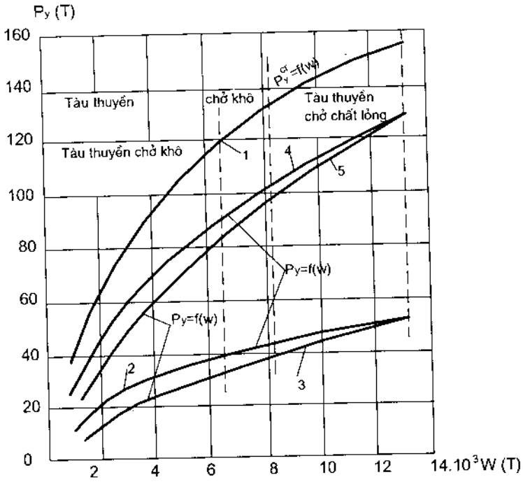
Hình 1-11 Đường quan hệ P_y = f(w) ;
