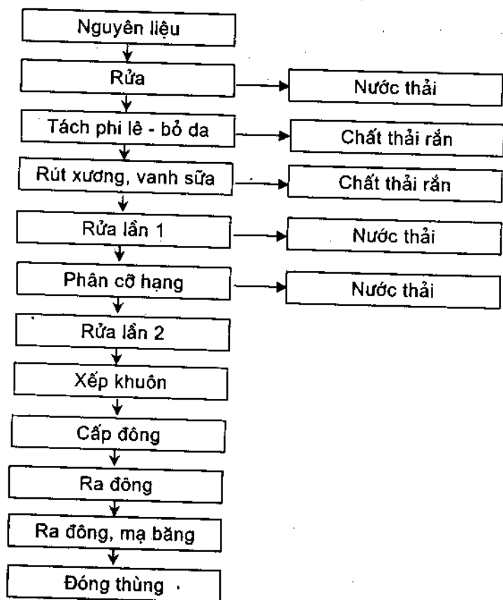
Hình 10.1. Sơ đồ quy trình sản xuất cá phi lê
