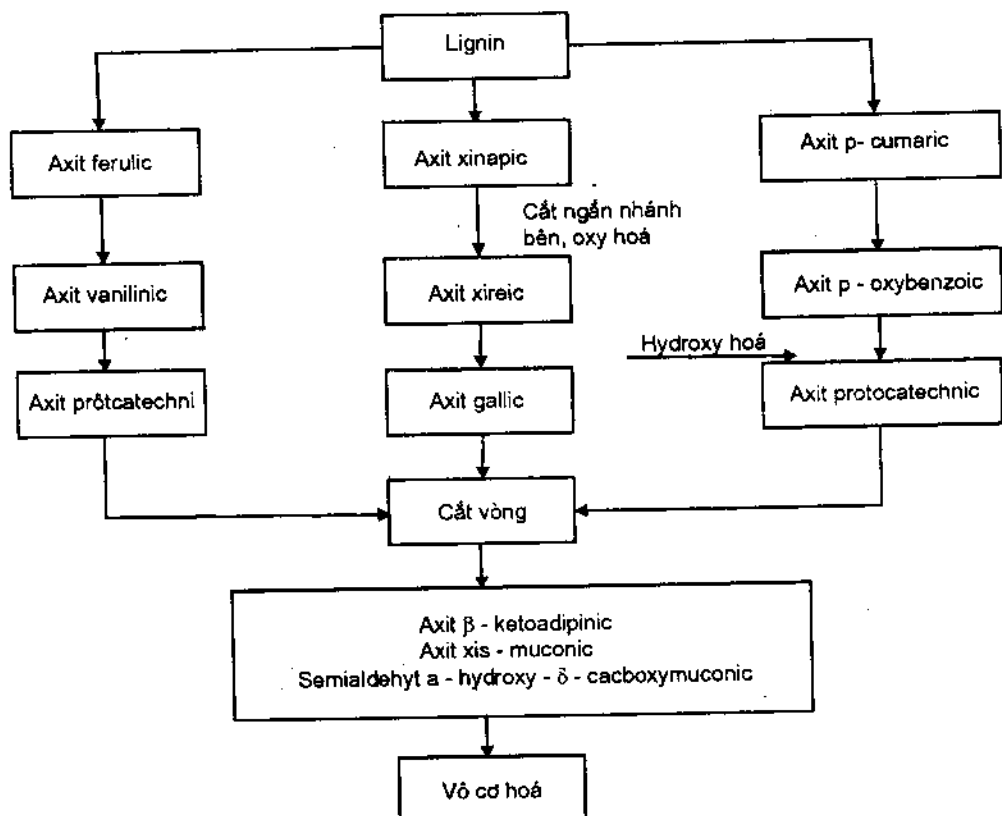
Hình 8.2. Sơ đồ cơ chế phân giải lignin
