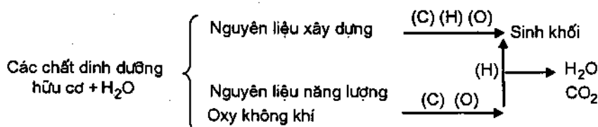
Hình 4.1. Sơ đồ dị dưỡng cacbon trong điều kiện hảo khí
