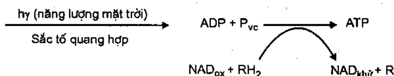
Hình 4.3. Sơ đồ tự dưỡng cacbon
