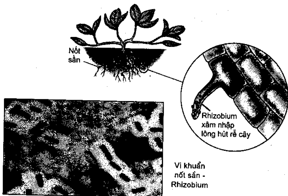
Hình 8.6. Cơ chế của quá trình cố định nitơ phân tử ở cây họ Đậu
