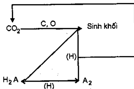
Hình 4.4. Sơ đồ tổng quát tự dưỡng quang năng
