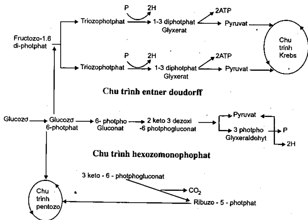
Hình 4.5. Sơ đồ các chu trình lên men
