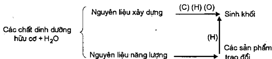
Hình 4.2. Sơ đồ dị dưỡng cacbon trong điều kiện yếm khí
