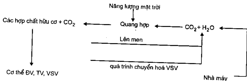
Hình 8.1. Sơ đồ chu chuyển cacbon trong tự nhiên
