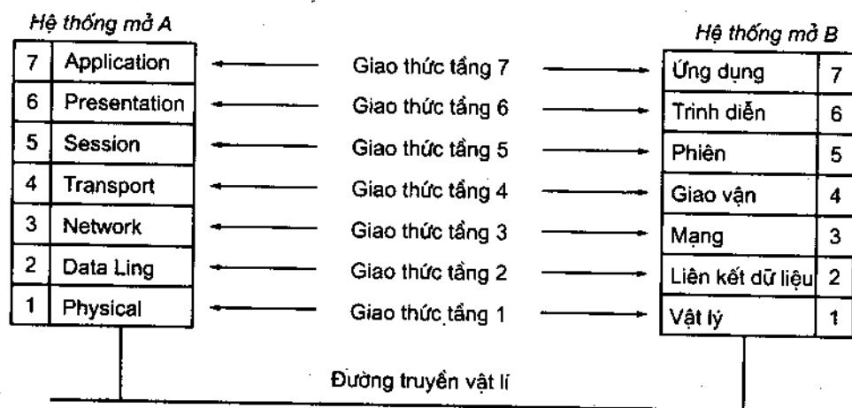
Hình 2.2. Mô hình OSI 7 tầng
