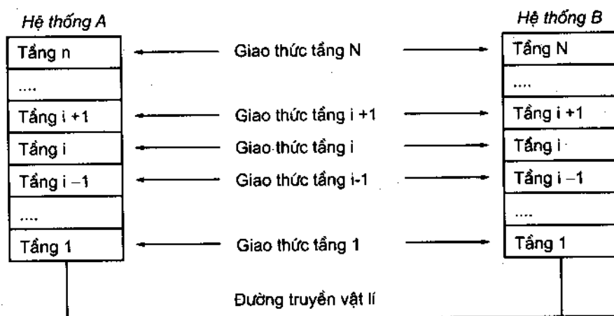
Hình 2.1. Mô hình kiến trúc mạng phân tầng
