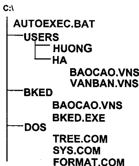
Cây thư mục hiển thị trên màn hình khi dùng lệnh TREE/f
