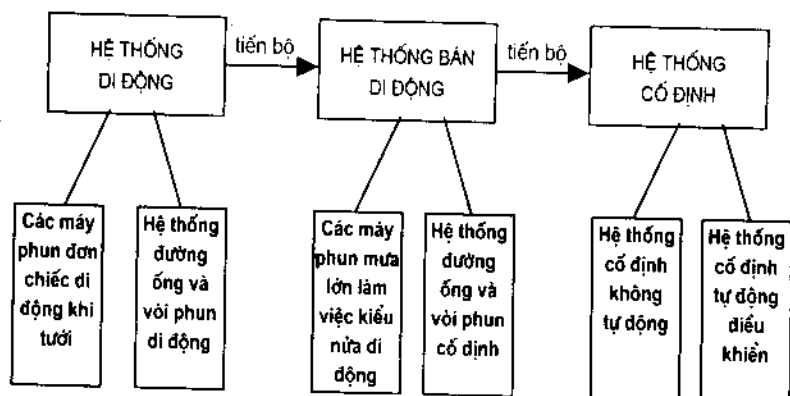
Sơ đồ hệ thống tưới phun mưa
