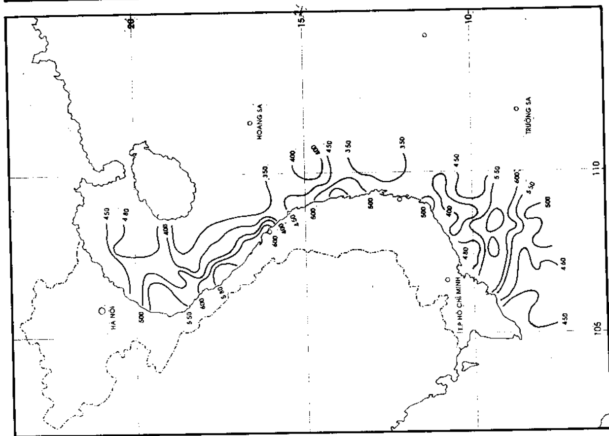
HÌNH VII.9. PHÂN BỐ MUỐI \text{SiO}_2 , TẦNG MẶT THÁNG X/1989 - 1/1990
