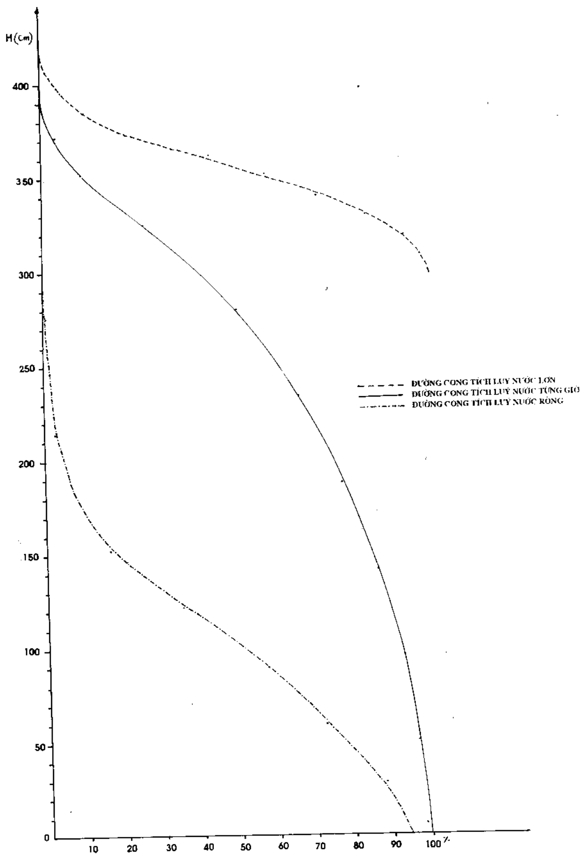
HÌNH III.4. ĐƯỜNG CỘNG TÍCH LŨY MỨC NƯỚC TÙNG GIÒ, NƯỚC LỚN, NƯỚC RÒNG TRẠM : VŨNG TÀU
