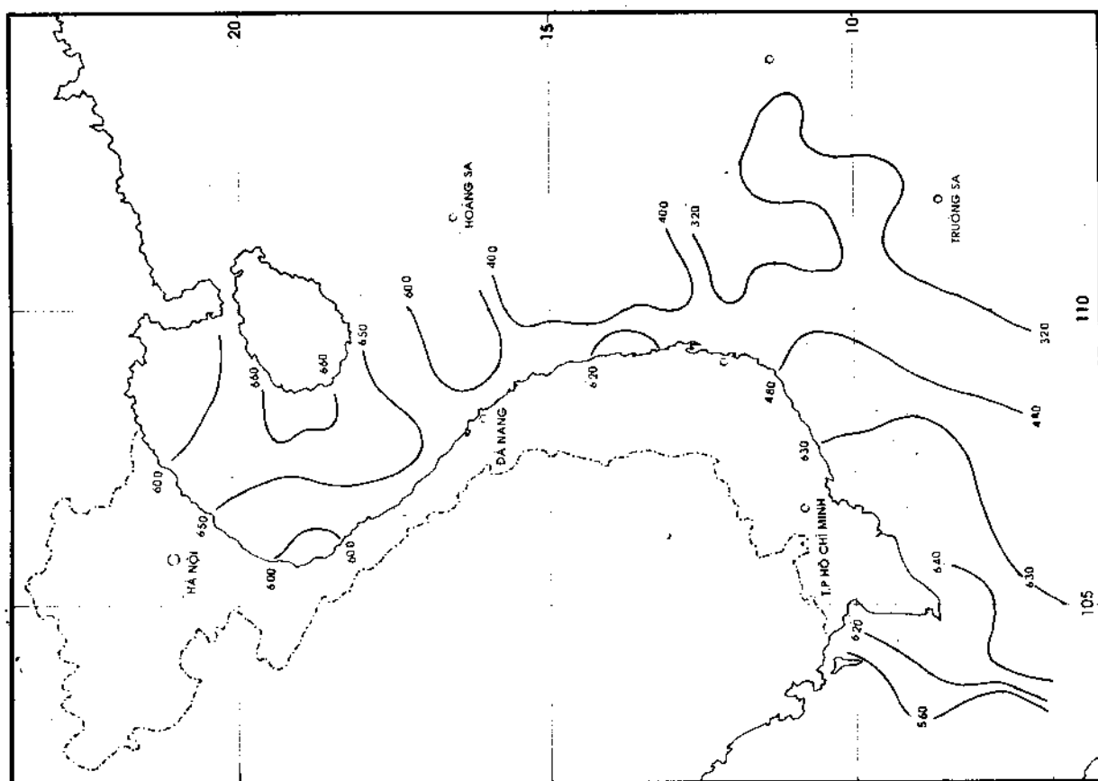
HÌNH VII.15. PHÂN BỐ OXY HÒA TÁN TẦNG ĐÁY, THÁNG V - VIII/1995
