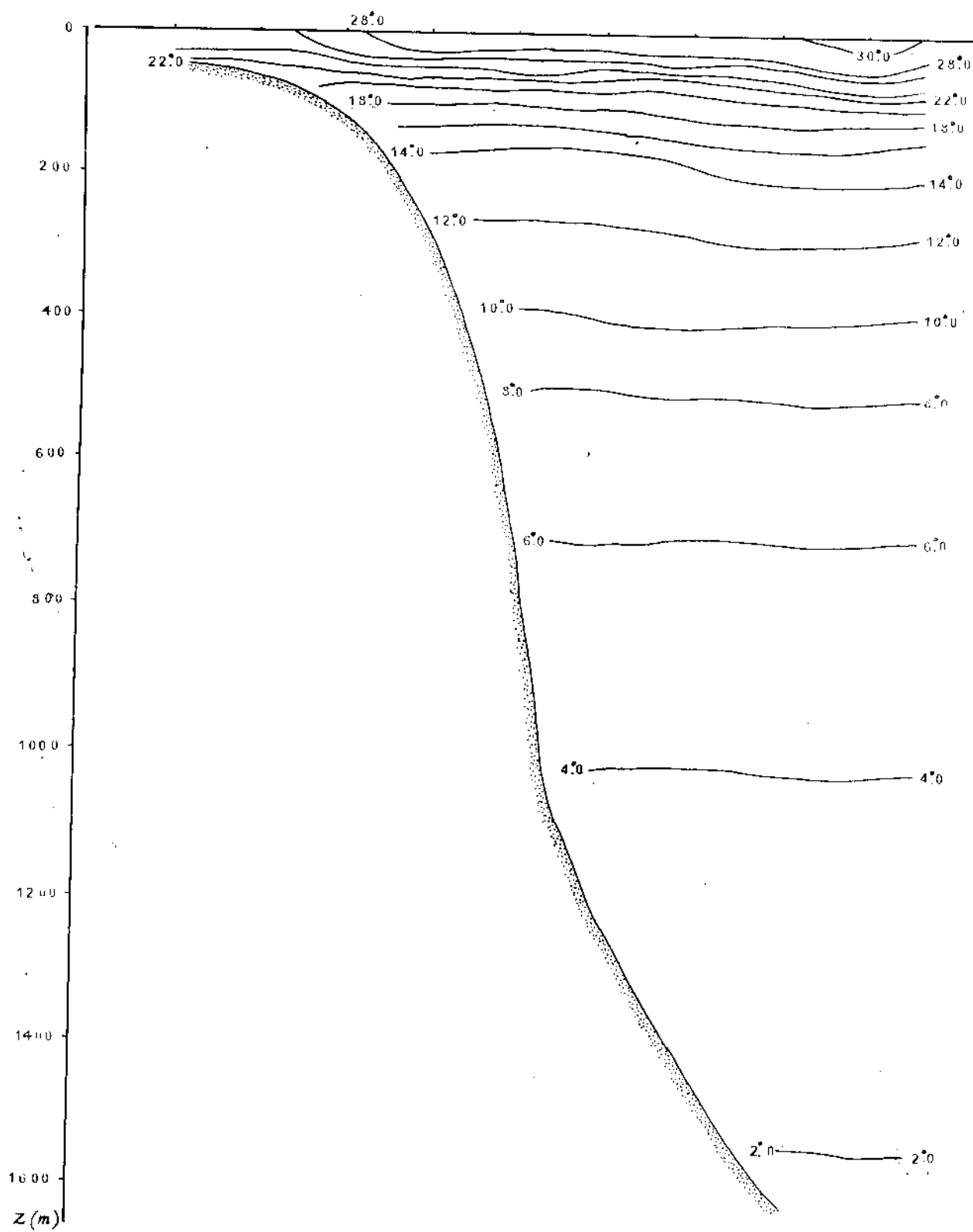
HÌNH VI.15. PHÂN BỐ NHIỆT ĐỘ ( ^{\circ}\text{C} ) NƯỚC THEO MẶT CẮT \phi = 11^{\circ} BẮC THÁNG VI/1994
