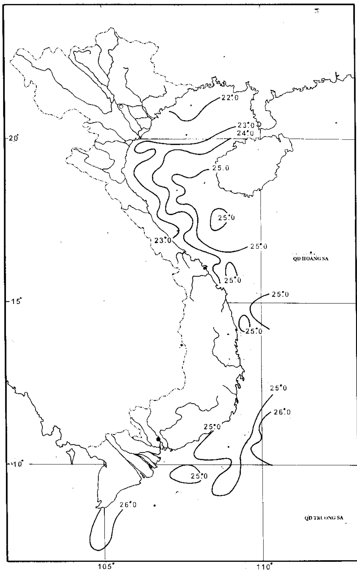
HÌNH VI.7. PHÂN BỐ NHIỆT ĐỘ (°C) NƯỚC BỀ MẶT THÁNG I/1990
