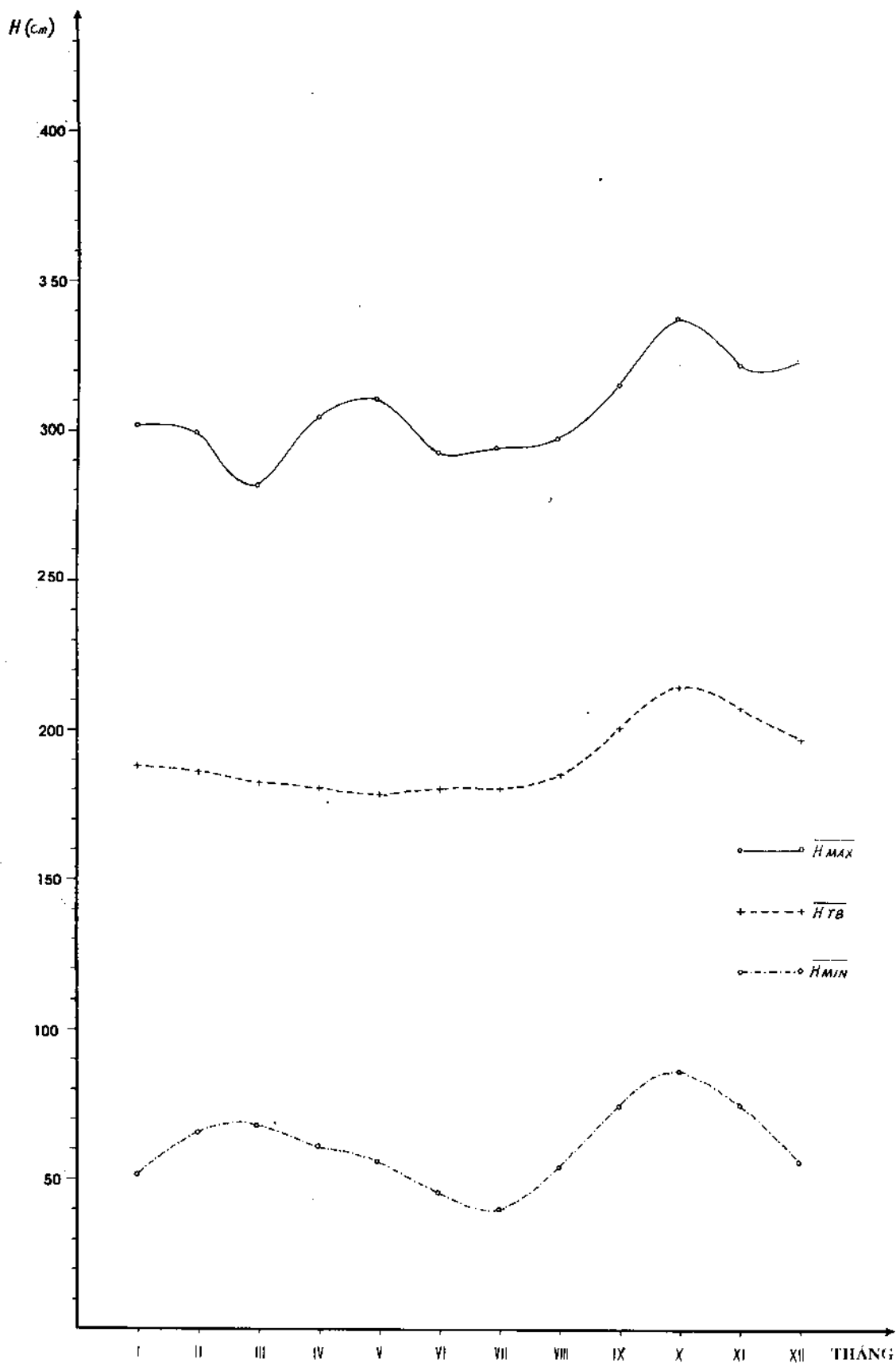
HÌNH III.3. BIẾN TRÌNH NĂM CỦA MỨC NƯỚC BIỂN CỰC ĐẠI, TRUNG BÌNH, CỰC TIỂU TRẠM : HÒN NGŨ
