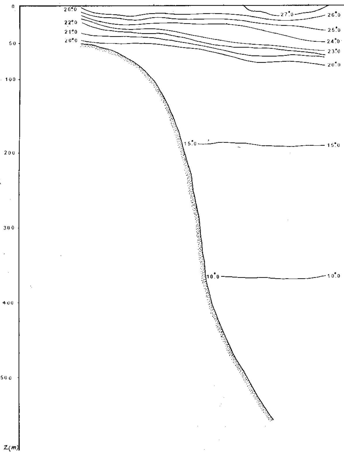
HÌNH VI.11. PHÂN BỐ NHIỆT ĐỘ ( ^{\circ}\text{C} ) NƯỚC THEO MẶT CẮT \varphi = 11^\circ BẮC THÁNG VIII/1993
