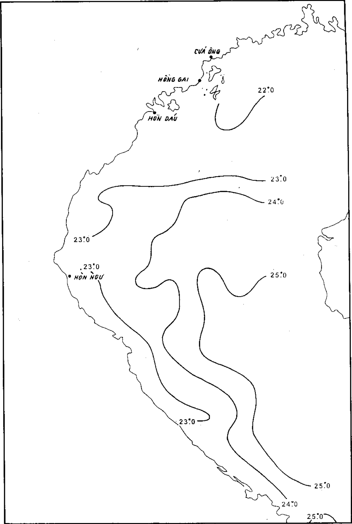
HÌNH V.1.1. PHÂN BỐ NHIỆT ĐỘ (°C) NƯỚC BỀ MẶT (VỊNH BẮC BỘ, THÁNG XII/ 1989)
