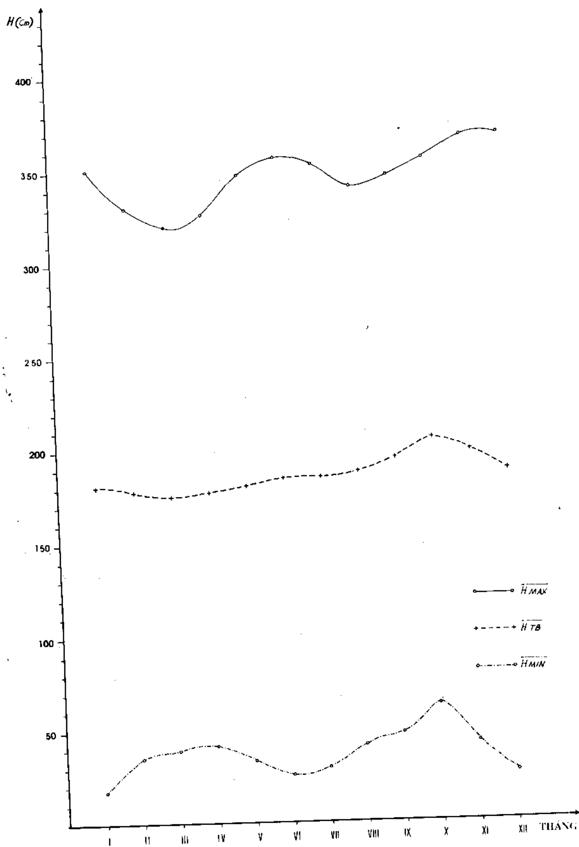
HÌNH III.3. BIẾN TRÌNH NAM CỦA MỨC NƯỚC BIỂN CỰC ĐẠI, TRUNG BÌNH, CỰC TIỂU TRẠM : HÒN DẦU
