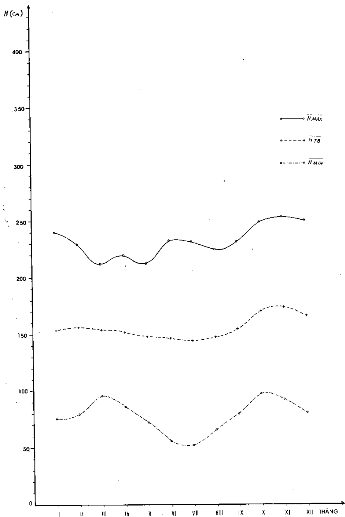
HÌNH III.3. BIẾN TRÌNH NĂM CỦA MỨC NƯỚC BIỂN CỰC ĐẠI, TRUNG BÌNH, CỰC THIỂU TRẠM: QUI NHƠN
