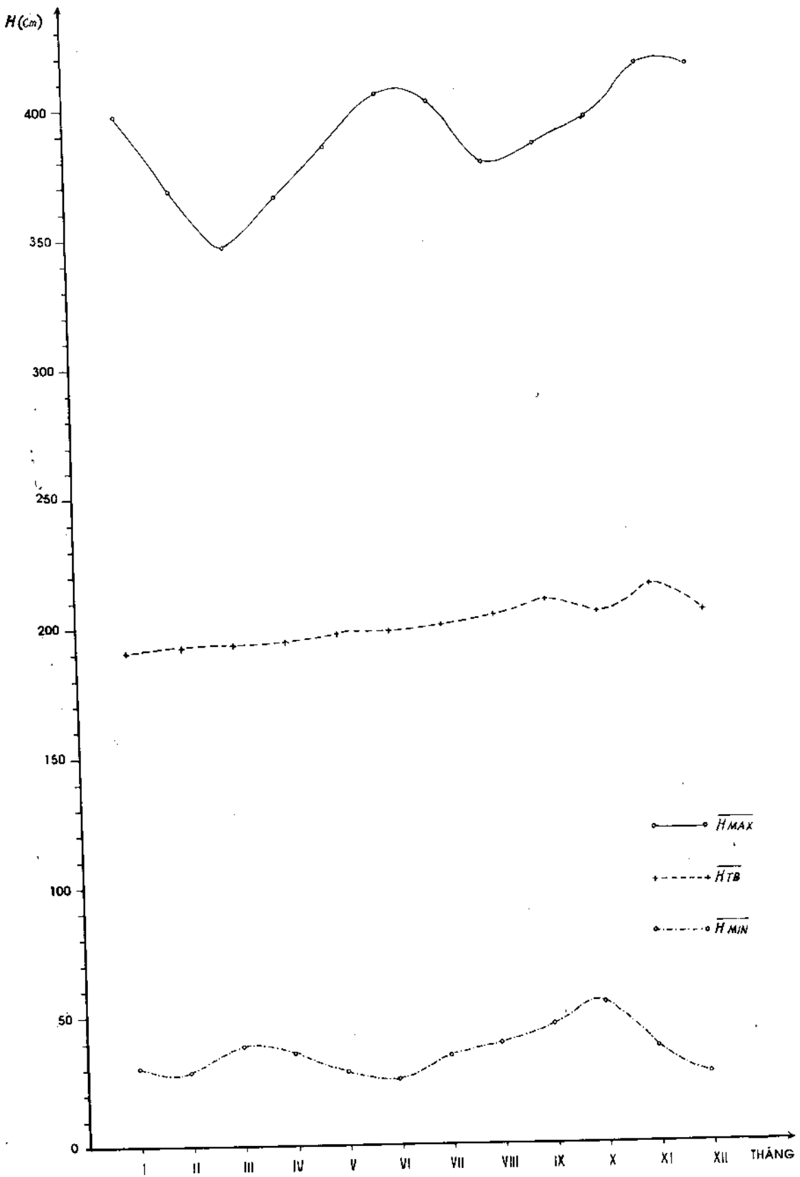
HÌNH III.3. BIẾN TRÌNH NAM CỦA MỨC NƯỚC BIỂN CỰC ĐẠI, TRUNG BÌNH, CỰC TIỂU TRẠM : CÔ TÔ
