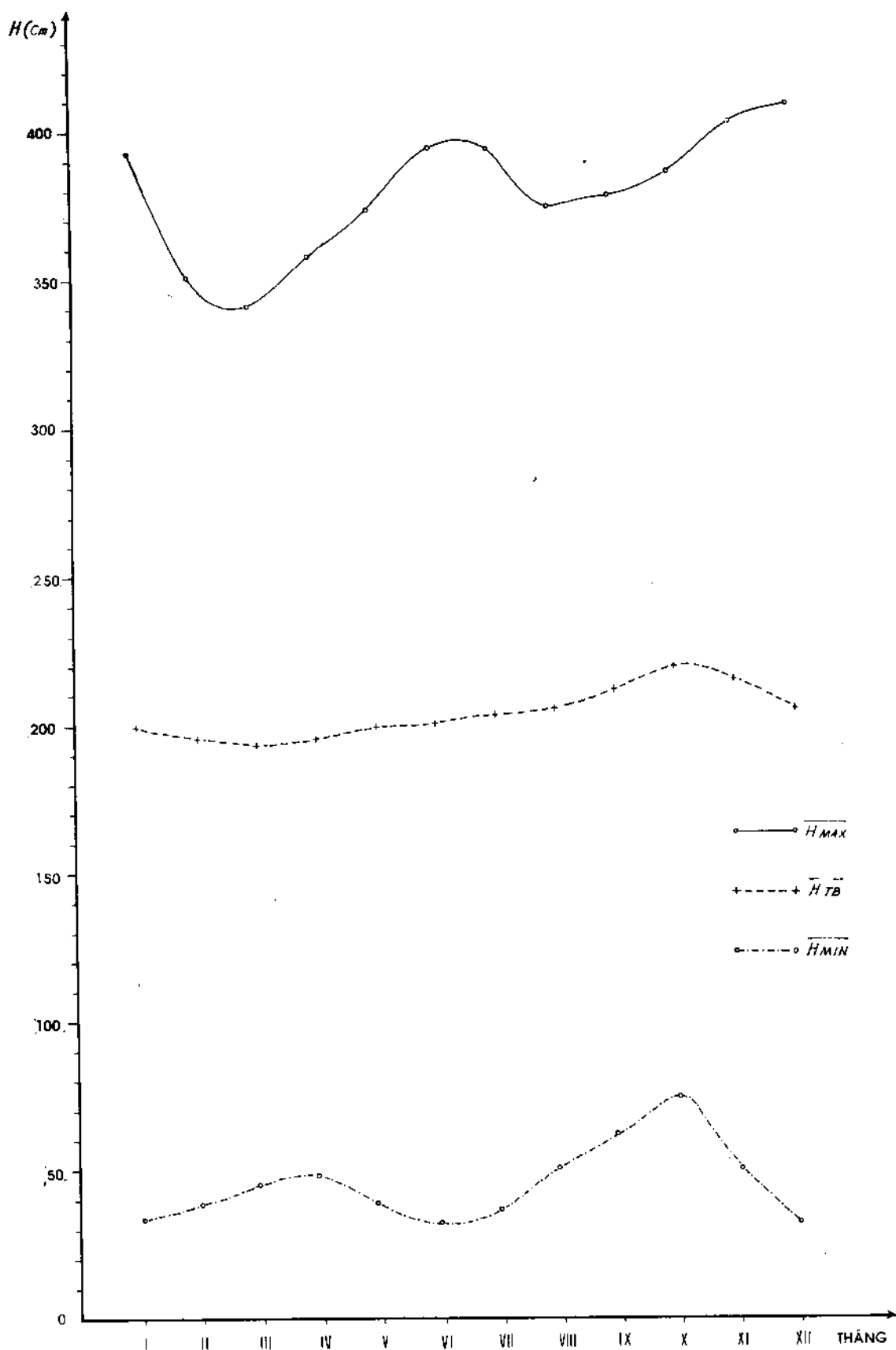
HÌNH III.3. BIẾN TRÌNH NĂM CỦA MỨC NƯỚC BIỂN CỰC ĐẠI, TRUNG BÌNH, CỰC TIỂU TRẠM : HÒN GAI
