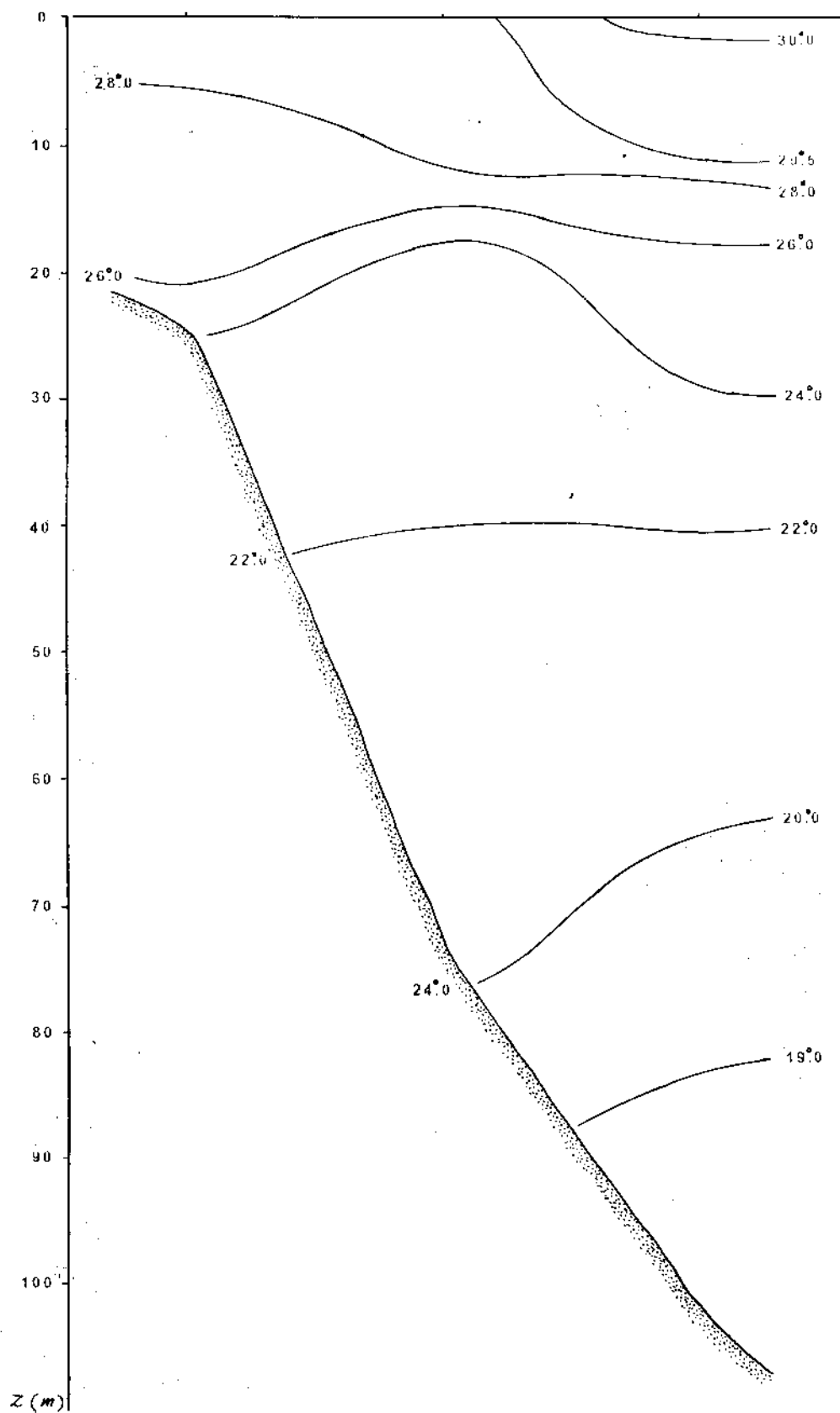
HÌNH VI.13. PHÂN BỐ NHIỆT ĐỘ ( ^\circ\text{C} ) NƯỚC THEO MẶT CẮT \varphi = 16^\circ BẮC THÁNG VI/1996
