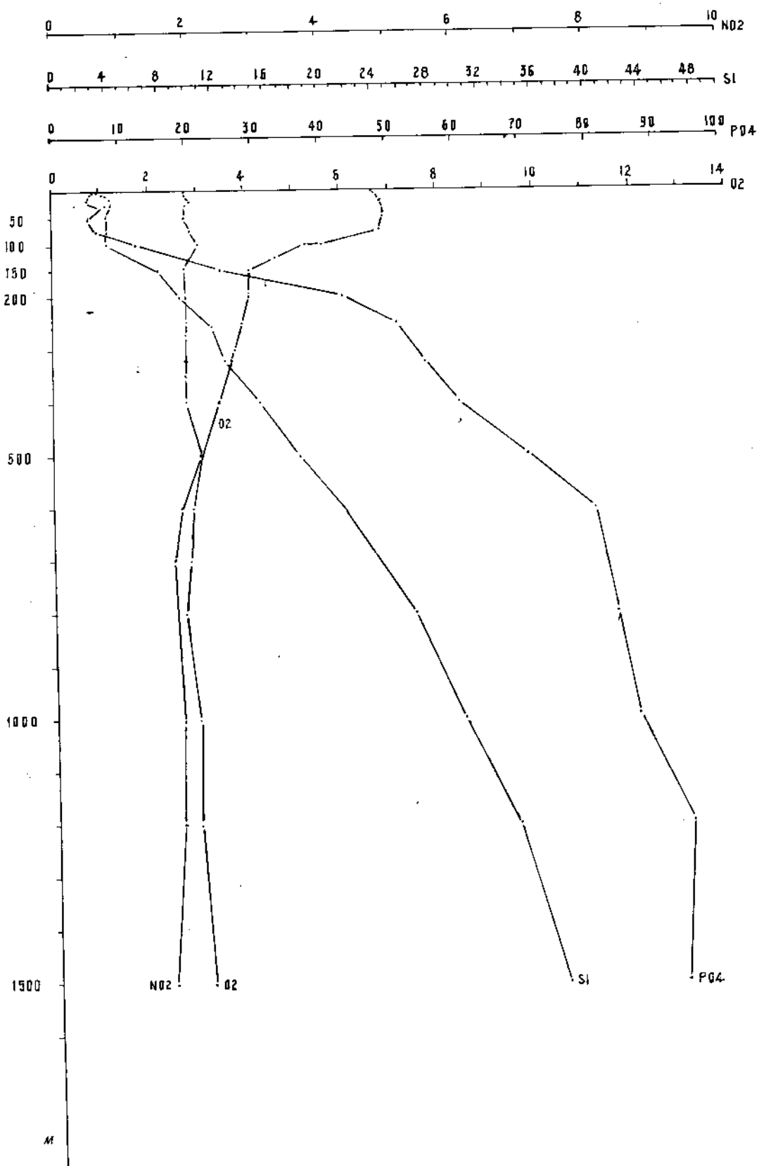
HÌNH VII.13. PHÂN BỐ CÁC YẾU TỐ THỦY HOÁ THEO ĐỘ SÂU TẠI TRẠM 268 (12°00N, 110°00E) THỜI KỲ MÙA ĐÔNG
