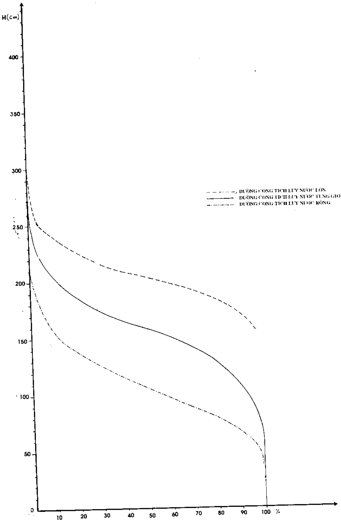
HÌNH III.4. ĐƯỜNG CỘNG TÍCH LŨY MỨC NƯỚC TÙNG GIỎ, NƯỚC LỚN, NƯỚC RÒNG TRẠM : QUI NHƠN
