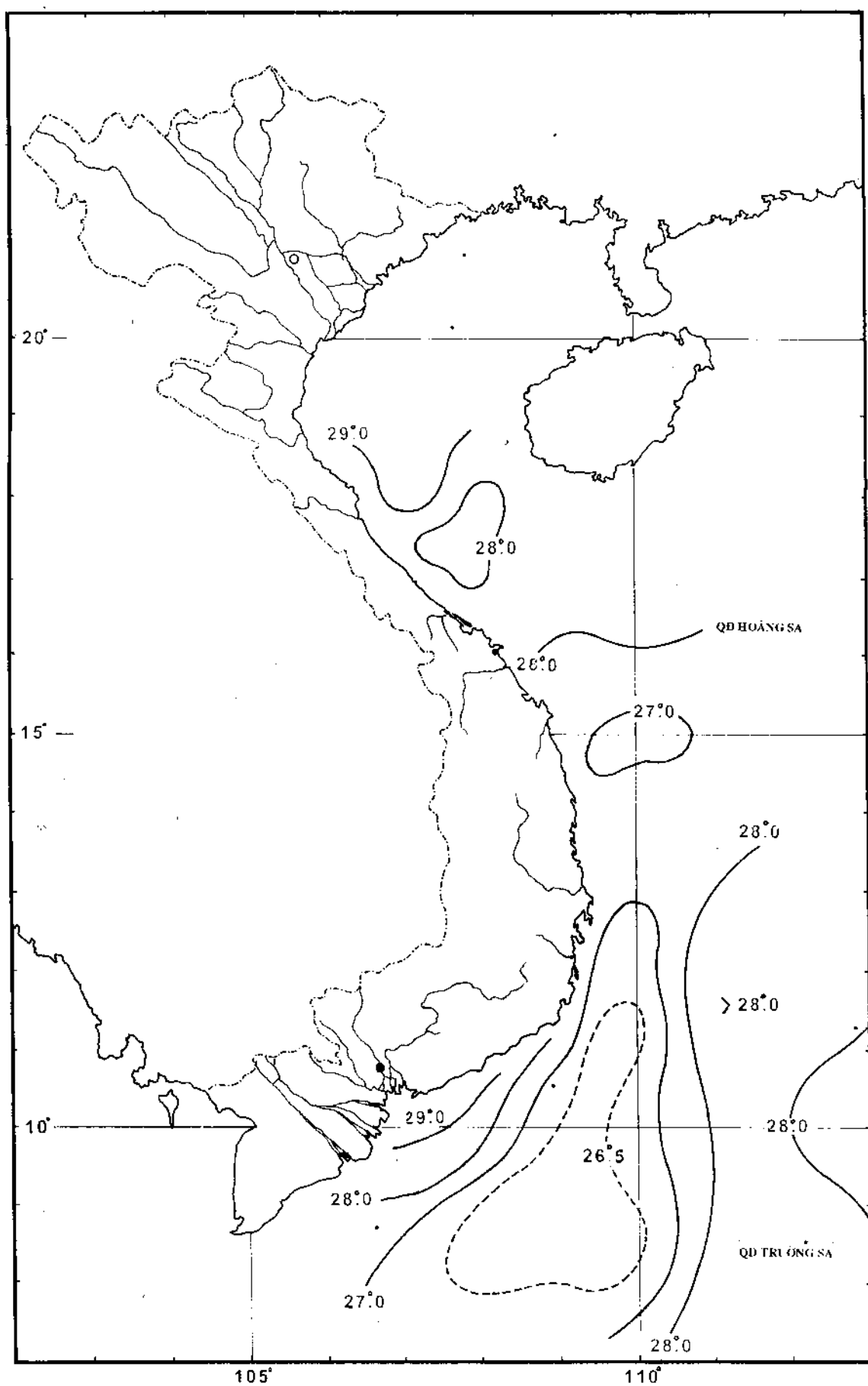
HÌNH VI.9. PHÂN BỐ NHIỆT ĐỘ (°C) NƯỚC BỀ MẶT THÁNG X - XI/1992
