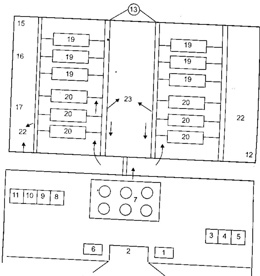
Sơ đồ mặt bằng của một trại lợn
