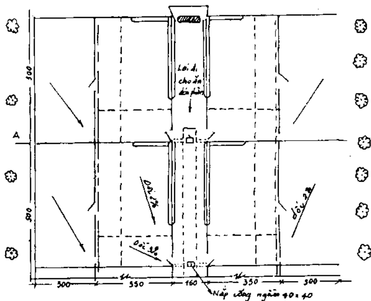
Sơ đồ thiết kế kiểu chuồng nuôi lợn thịt
