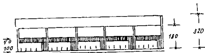
Sơ đồ thiết kế kiểu chuồng lợn đực giống
