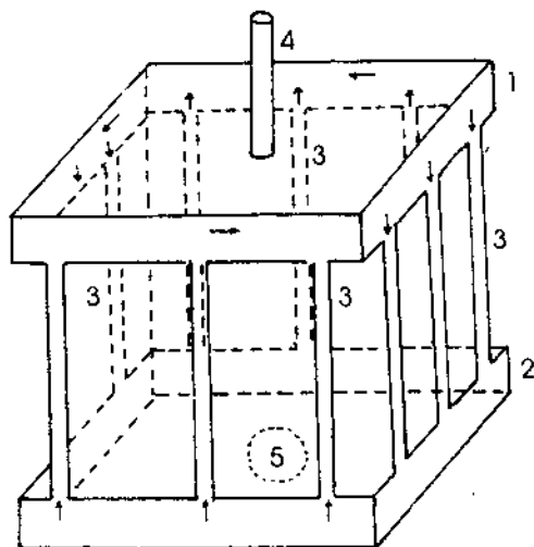
Hình 12. Sơ đồ phần làm bằng kim loại của tủ ấp trứng bằng nước nóng
