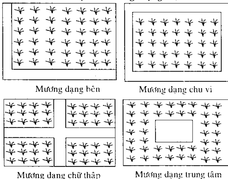
Hình 12. Các dạng mương ở ruộng nuôi tôm
