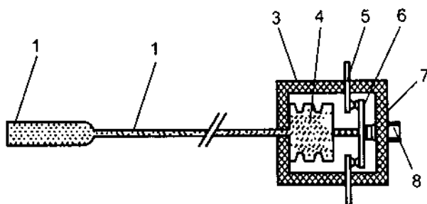
Hình 6.26. Role áp lực
