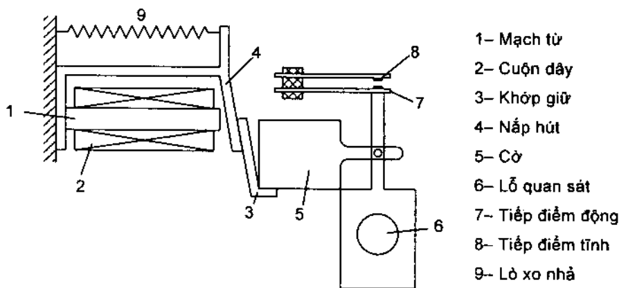
Hình 6.20. Rơle tín hiệu
