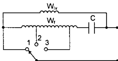
Hình 8.20. Quạt gió ba tốc độ W_{lv} — Cuộn chính; W_f — Cuộn phụ.
