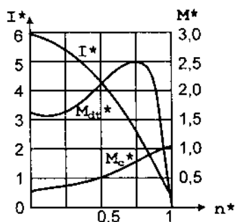
Hình 4.15. Đặc tính mở máy của động cơ không đồng bộ
