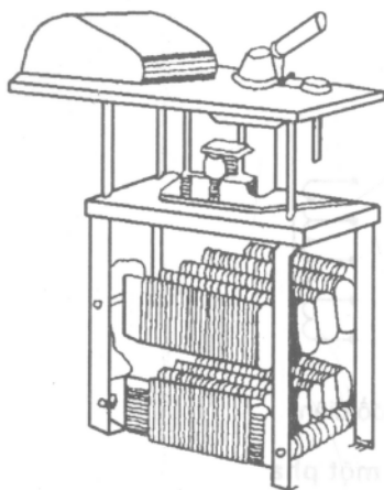
a) Biến trở dầu
