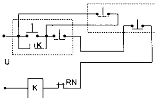
a) Điều khiển hai nơi
