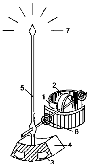
Hình 7.3. Cơ cấu điện động
