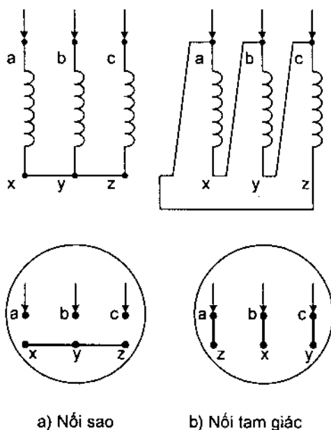
Hình 4.9. Cách đấu động cơ ba pha
