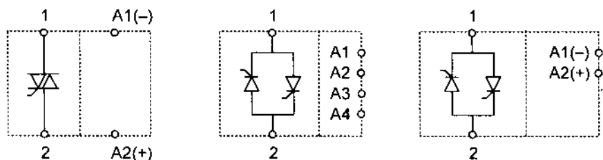
a) Một cực, dùng triac, nguồn điều khiển một chiều
