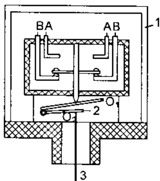
Hình 6.28. Công tắc phao
