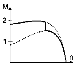
e) Động cơ có tụ khởi động và làm việc
