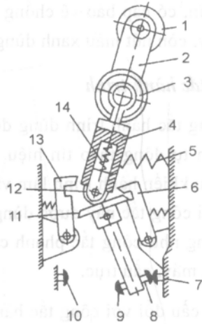
Hình 6.7. Công tắc hành trình kiểu đòn
