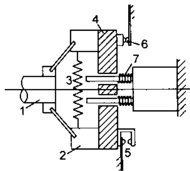
Hình 6.27. Role tốc độ kiểu ly tâm
