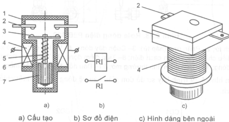
Hình 5.30. Role dòng điện khởi động động cơ một pha
