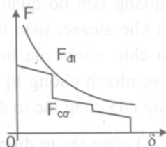
Hình 6.32. Đặc tính lực của công tắc tơ
