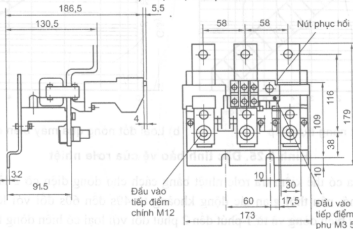
b) Loại có biến dòng
