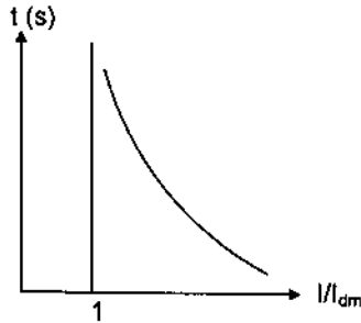
Hình 5.20. Đặc tính bảo vệ của role nhiệt
