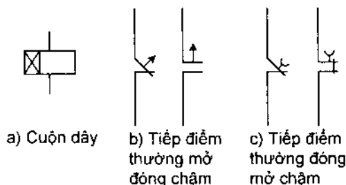
Hình 6.21. Sơ đồ điện rơle thời gian
