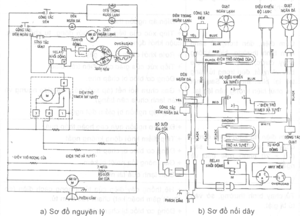
Hình 8.11. Mạch điện của tủ lạnh hai ngăn
