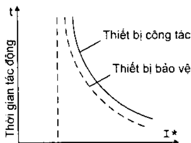
Hình 5.1. Đặc tính bảo vệ theo dòng điện
