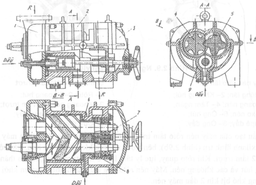
Hình 2.8. Máy nén trục vít (có hai vít) kiểu tràn dầu
