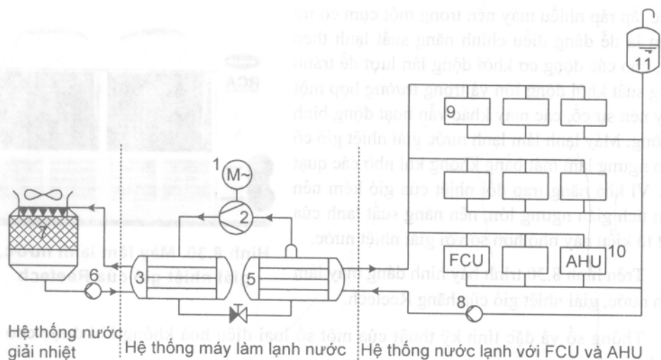
Hình 8.28. Nguyên lý điều hoà trung tâm nước
