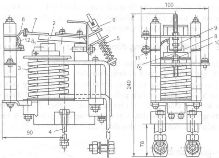
Hình 5.28. Rơle dòng điện PEB.300
