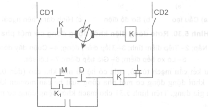
Hình 5.29. Bảo vệ động cơ một chiều khi ngắn mạch
