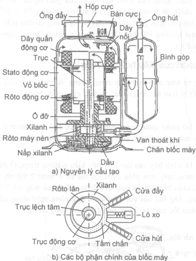
Hình 8.17. Máy nén kiểu rôto lăn
