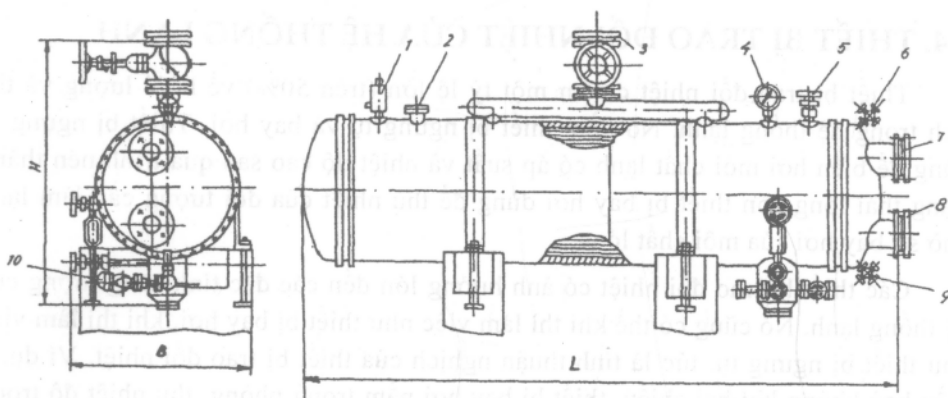
Hình 2.11a. Bình ngưng ống vỏ nằm ngang cho \text{NH}_3
