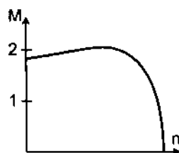
f) Động cơ ba pha
