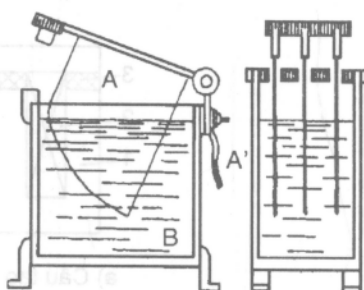
b) Biến trở dung dịch
