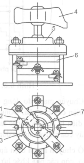
Hình 6.1. Chuyển mạch ba pha
