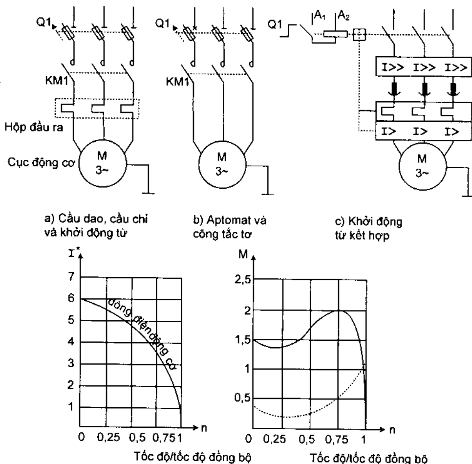
Hình 6.43. Mở máy trực tiếp động cơ rôto lồng sóc
