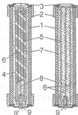
Hình 5.4. Cầu chì cao áp có chất nhồi
