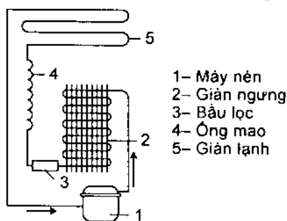
Hình 8.1. Nguyên lý tủ lạnh
