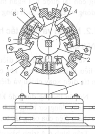
Hình 6.2. Chuyển mạch kiểu cam
