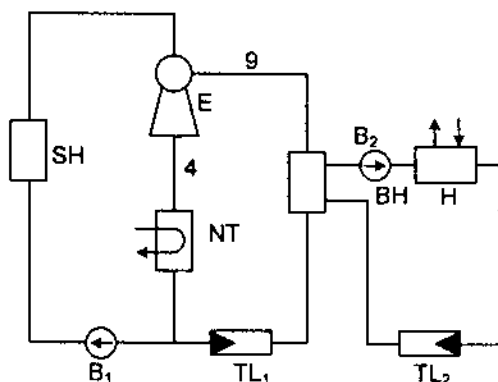
Hình 3.12. Sơ đồ nguyên lý máy lạnh ejector
