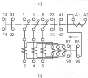
Hình 6.40. Khởi động từ đơn có I_{dm} = 300A
