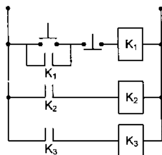
d) Điều khiển lần lượt
