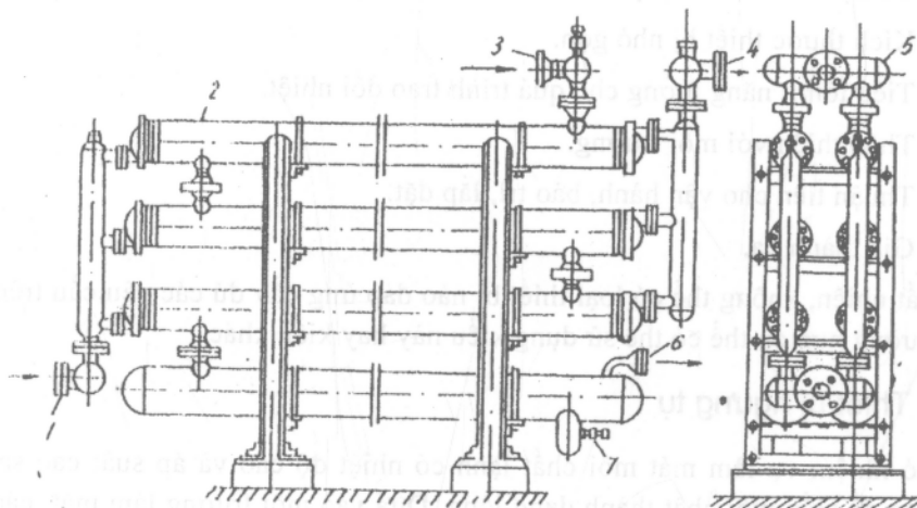
Hình 2.11b. Thiết bị ngưng tụ kiểu phân tử
