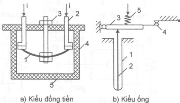
Hình 5.26. Role điều chỉnh nhiệt độ
