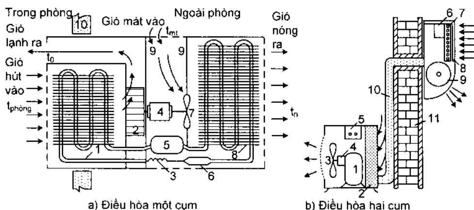
Hình 8.13. Nguyên lý điều hoà gia dụng
