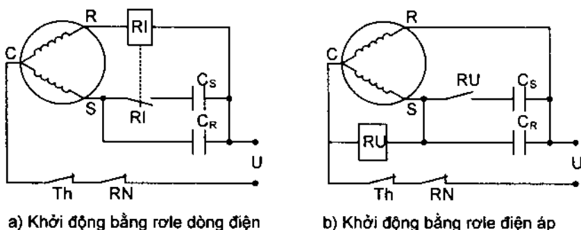
Hình 8.19. Sơ đồ khởi động động cơ máy nén
