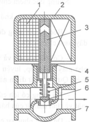
Hình 6.52. Van điện từ
