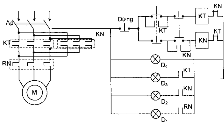
b) Trực tiếp có đảo chiều
