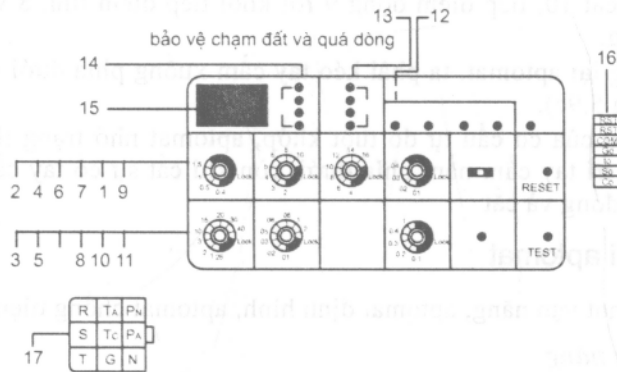
Hình 5.11. Bảng các thông số đặt trị số tác động, các núm thao tác
