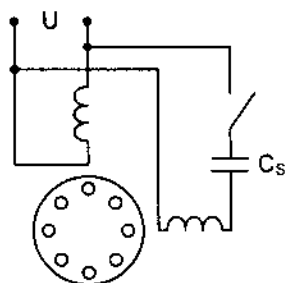
a) Động cơ vành chập b) Động cơ có cuộn khởi động c) Động cơ có tụ làm việc
