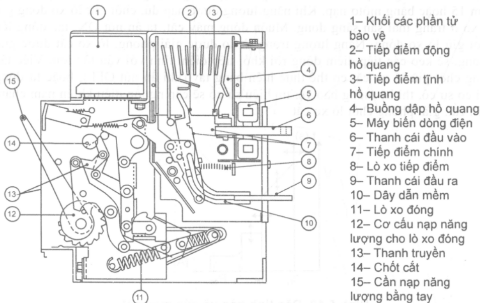
Hình 5.10. Các bộ phận của aptomat vạn năng
