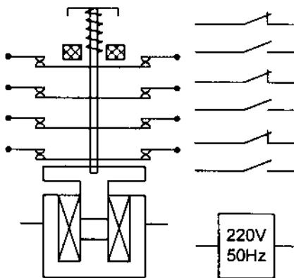
Hình 6.19. Rơle trung gian
