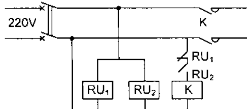
Hình 5.33. Bảo vệ điện áp cao và thấp
