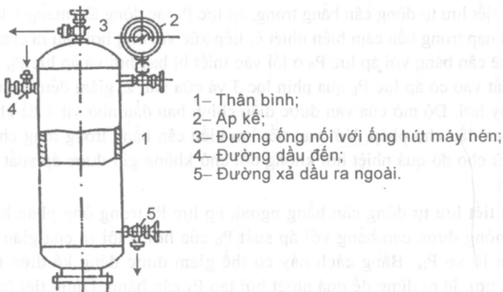
Hình 2.17. Bình chứa dầu
