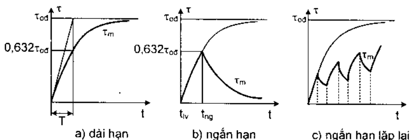
Hình 4.14. Các chế độ làm việc của thiết bị điện
