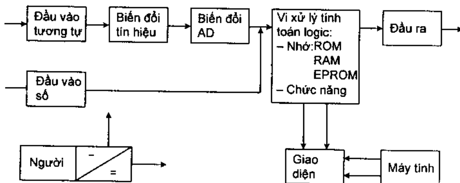
Hình 6.25. Sơ đồ khối của role số
