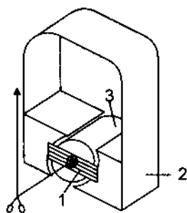
Hình 7.2. Cơ cấu điện từ
