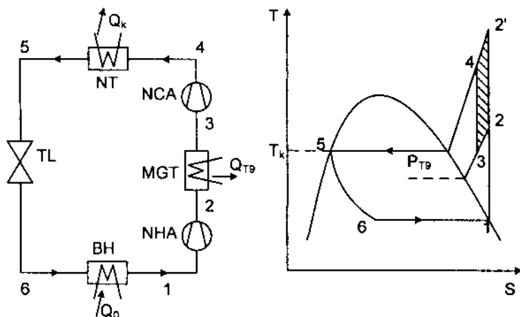
Hình 3.8. Chu trình 2 cấp nén, một tiết lưu làm mát trung gian không hoàn toàn
