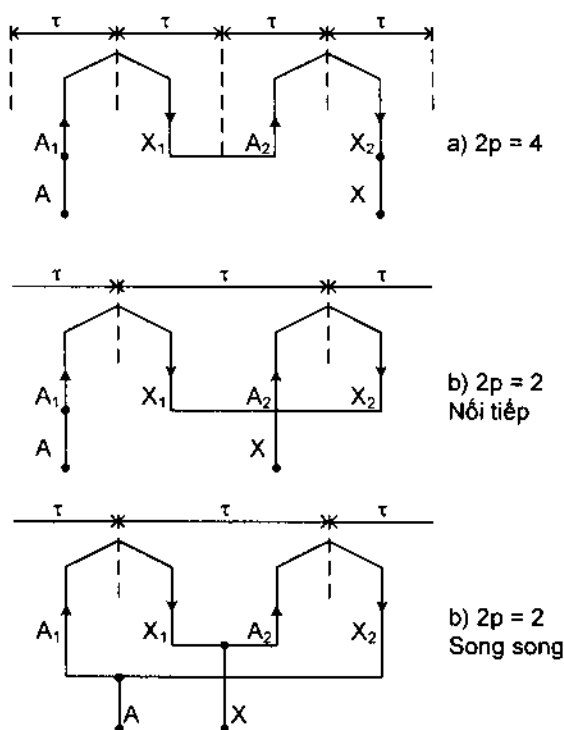
Hình 4.11. Thay đổi số đôi cực
