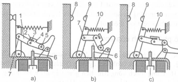
Hình 5.9. Cơ cấu tự do trượt khớp
