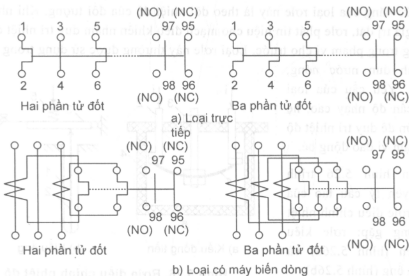
Hình 5.24. Sơ đồ điện của role nhiệt
