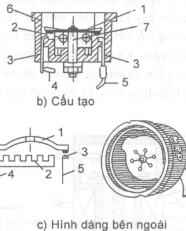
Hình 8.7. Role nhiệt bảo vệ quá dòng điện kiểu tròn, lắp trực tiếp trên vỏ lốc
