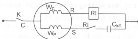
Hình 5.31. Sơ đồ khởi động động cơ một pha bằng role dòng và tụ điện
