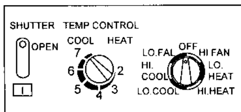
Công tắc quay cánh hướng gió Núm khống chế nhiệt độ Núm chức năng
