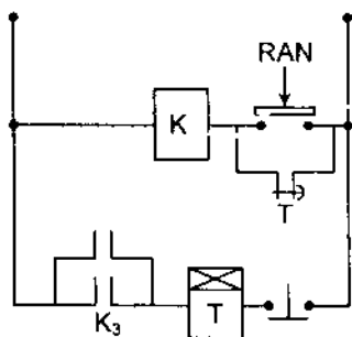
c) Điều khiển có trễ
