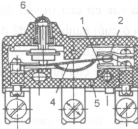
Hình 6.6. Công tắc hành trình tế vi
