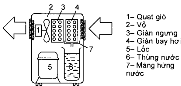
Hình 8.12. Cấu tạo máy hút ẩm dân dụng
