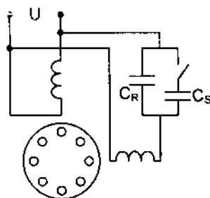
a) Động cơ vành chập b) Động cơ có cuộn khởi động c) Động cơ có tụ làm việc
