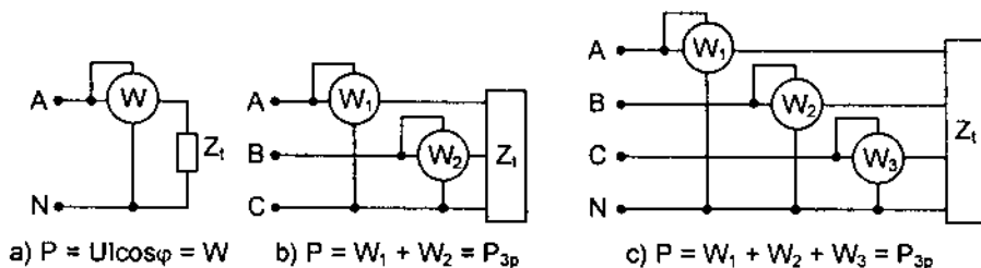
Hình 7.8. Đo công suất
