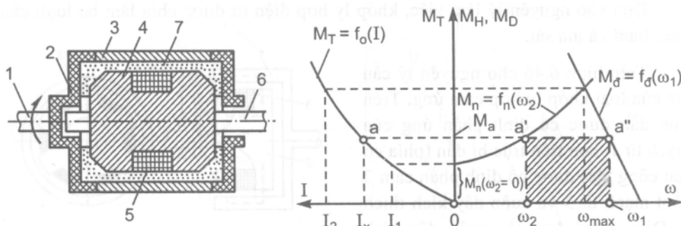
Hình 6.48. Khớp ly hợp điện từ kiểu bám
