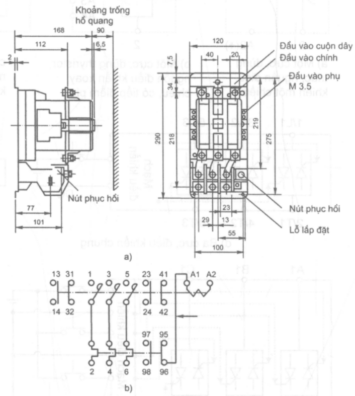
Hình 6.39. Khởi động từ đơn 150A
