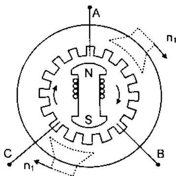
Hình 4.2. Động cơ đồng bộ
