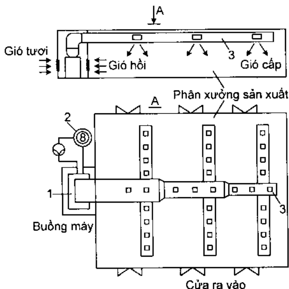
Hình 8.27. Vi dụ ứng dụng của máy điều hoà nguyên cụm giải nhiệt nước
