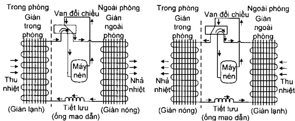
Hình 8.14. Điều hoà hai chiều
