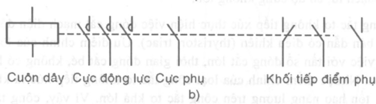
Hình 6.37. Công tắc tơ điện xoay chiều
