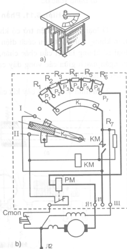
Hình 6.13. Biến trở khô
