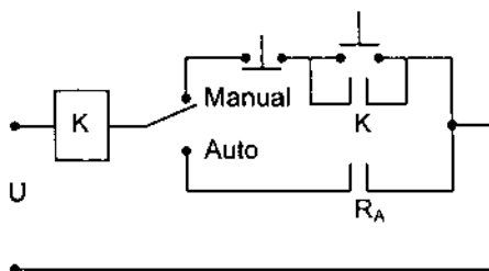
b) Điều khiển hai chế độ
