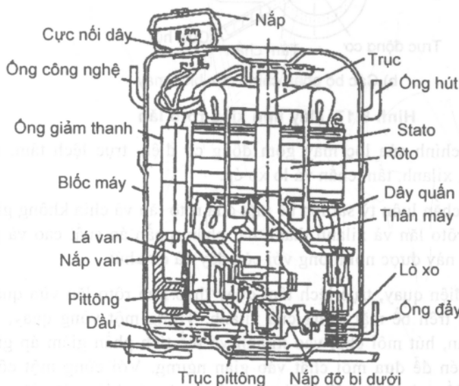
Hình 8.16. Máy nén kiểu pittông
