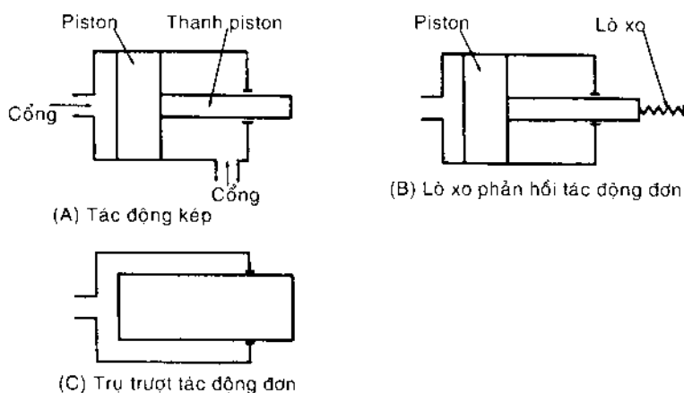
Hình 9-3. Sơ đồ của cylinder không quay; (A) Tác động kép; (B) Lò xo phản hồi tác động đơn; (C) Trượt trượt tác động đơn.
