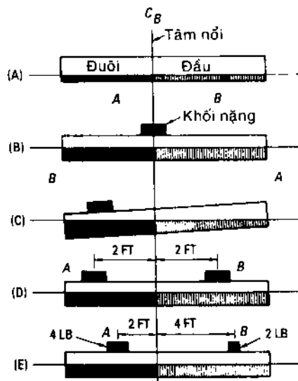
Hình 1-18. Tâm nối và ảnh hưởng của vị trí khối nặng.
