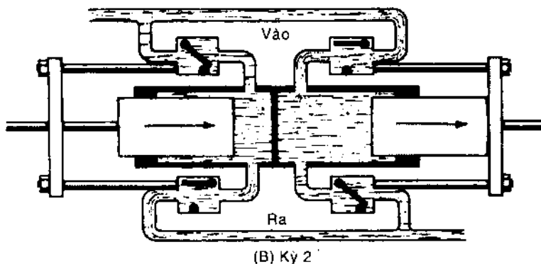
Hình 4-15. Chu trình làm việc hai kỳ của bơm trụ trượt tác động kép, phốt kín bên ngoài.
