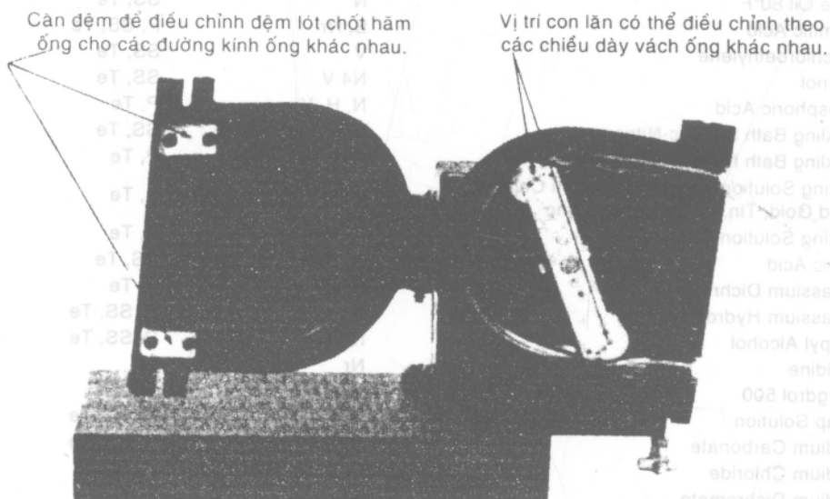
Hình 5-25. Đầu bơm hở để dễ dàng thay kích cỡ ống.
