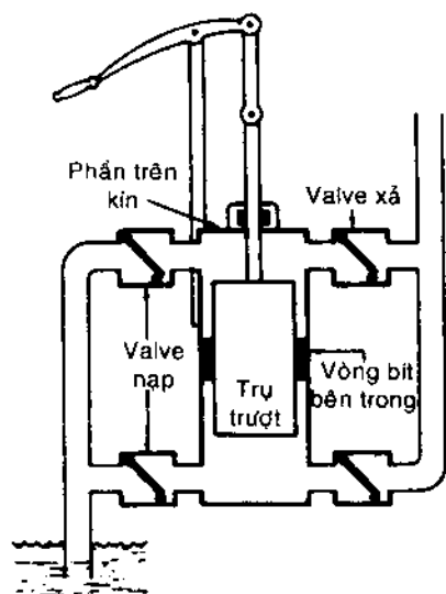
Hình 4-12. Kết cấu cơ bản của bơm đẩy trụ trượt tác động kép với phốt kín bên trong.
