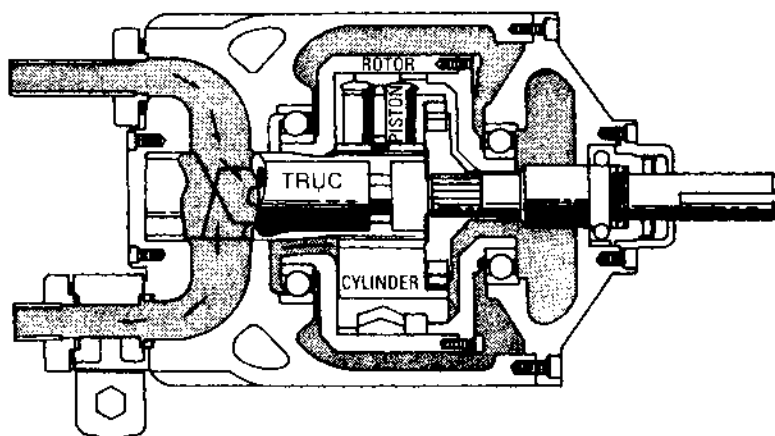
Hình 8-6. Kết cấu động cơ thủy lực loại piston hướng kính có hành trình không đổi.
