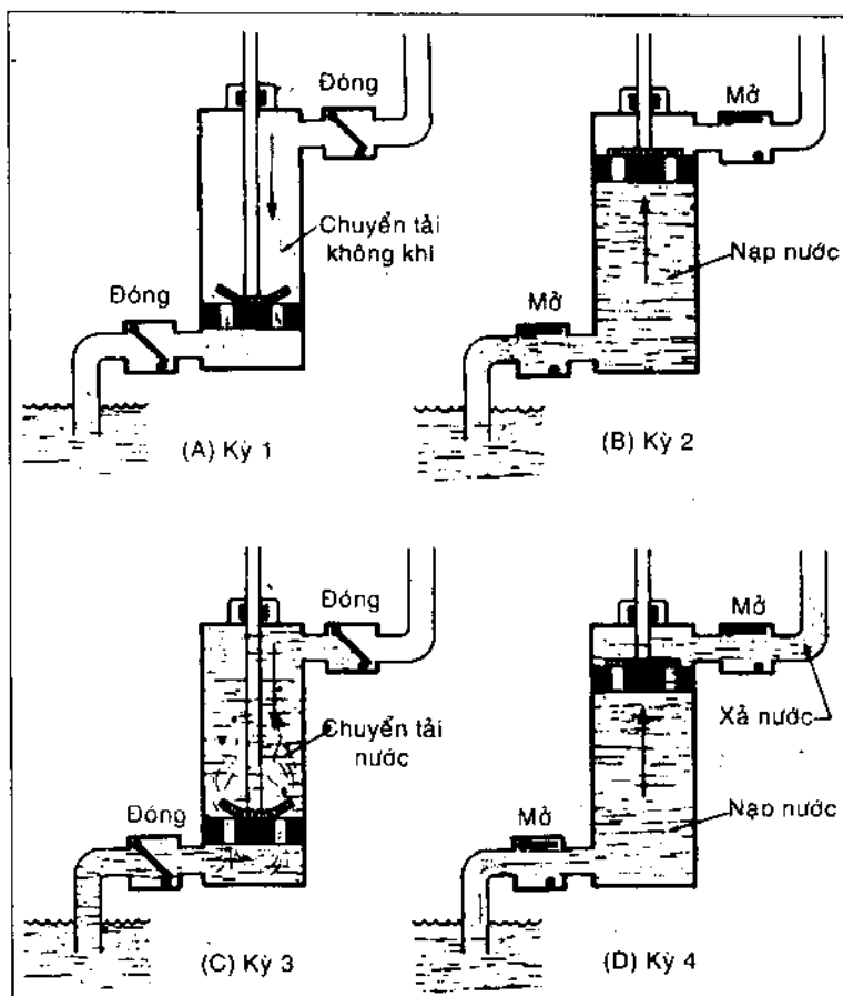
Hình 4-8. Kết cấu cơ bản của bơm đẩy tác động đơn có valve một chiều trong piston.
