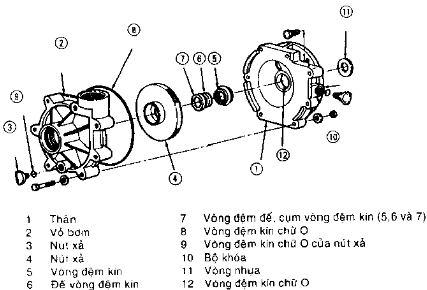
Hình 2-38. Các chi tiết của bơm ly tâm chống ầm mòn
