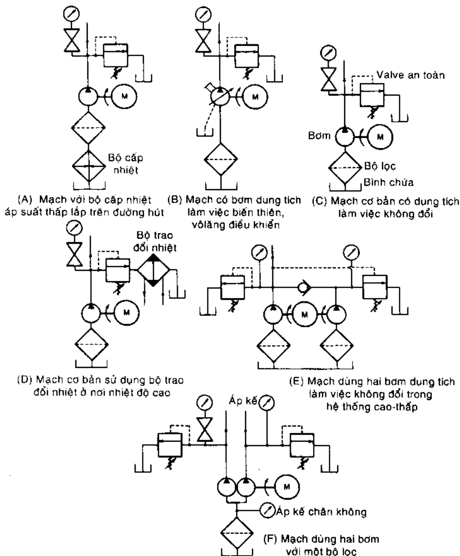
Hình 3-17. Các mạch bơm cơ bản.
