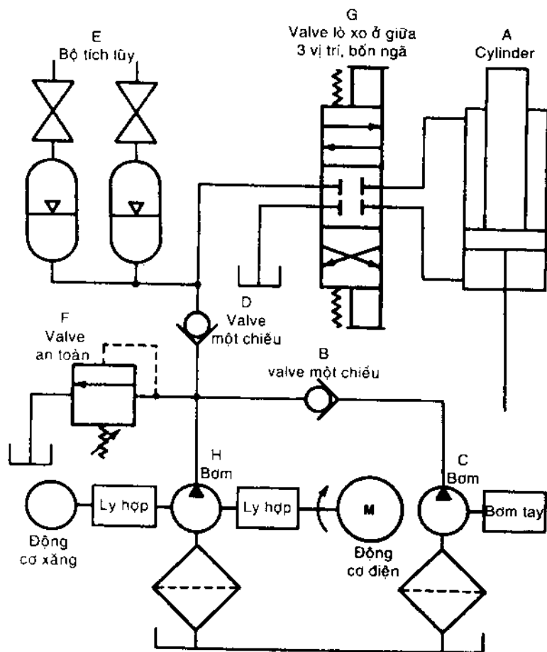
Hình 6-22. Mạch được thiết kế để tạo một công suất dự trữ trong trường hợp nguồn điện hỏng.
