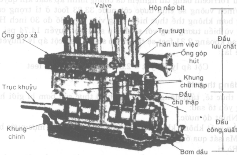
Hình 4-18. Các chi tiết bên trong của bơm piston tịnh tiến.
