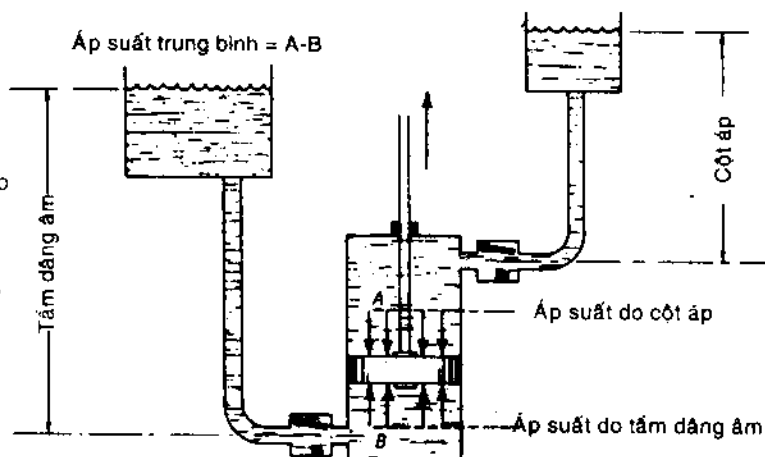
Hình 1-24. Tầm dâng âm, đôi khi được gọi là cột áp hút. Bơm là loại tác động kép, nhưng để đơn giản bộ valve thứ hai không được minh họa.
