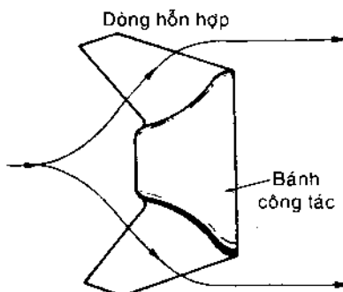
Hình 2-11. Loại bánh công tác dòng hỗn hợp.
