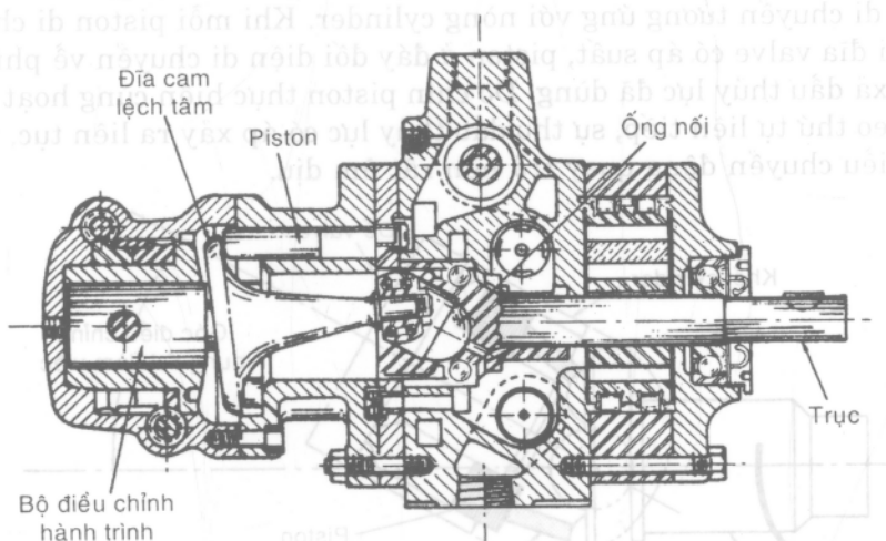
Hình 8-9. Kết cấu cơ bản của động cơ thủy lực có các valve điều khiển chính trong cùng một vỏ.
