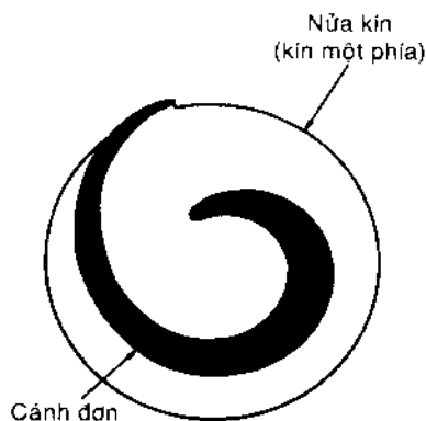
Hình 2-8. Bánh công tác nửa kín, cánh gạt đơn.
