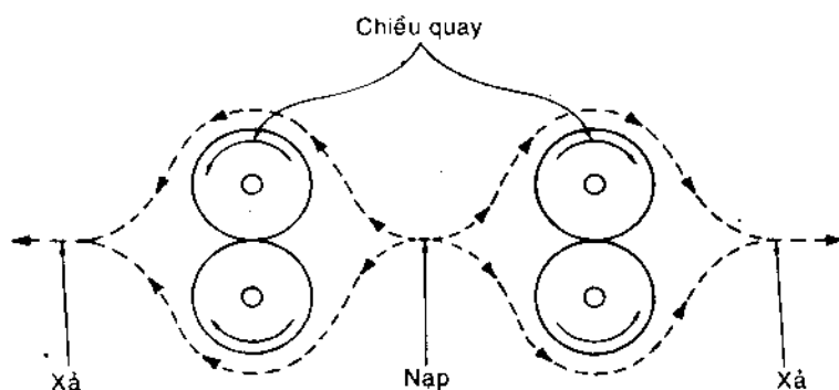
Hình 3-13. Dòng chất lỏng và chiều quay của bơm bánh răng.
