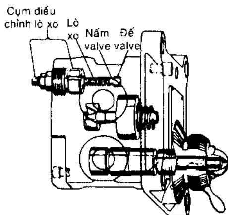
Hình 10-11. Valve điều khiển lưu lượng và bảo vệ quá tải.
