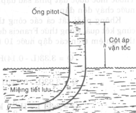
Hình 1-30. Nguyên lý cơ bản của ống pitot dùng để đo lưu lượng nước.
