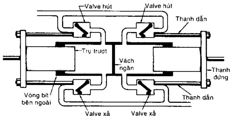
Hình 4-14. Kết cấu cơ bản của bơm đẩy trụ trượt tác động kép với phốt kín bên ngoài.
