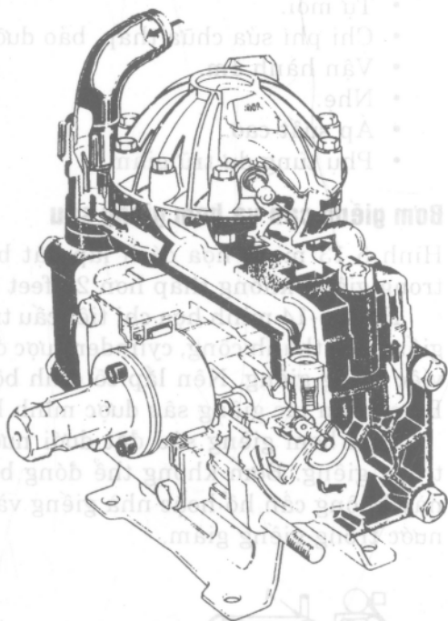
Hình 5-12. Bơm màng chắn, minh họa quỹ đạo lưu động.
