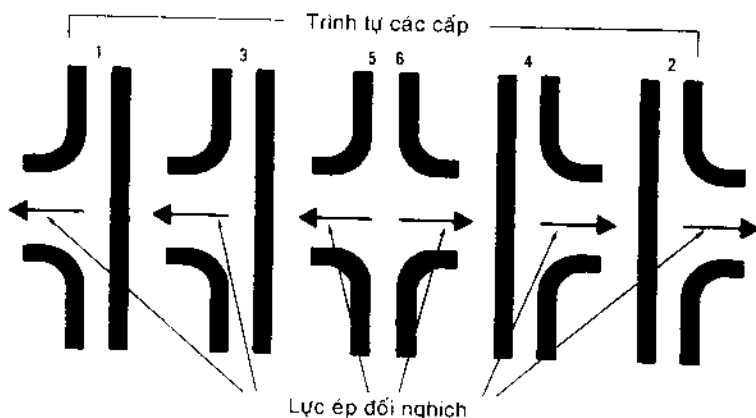
Hình 2-15. Cân bằng tự nhiên trong bơm ly tâm sáu cấp nhờ một bộ bốn bánh công tác hòng hút đơn (trái và phải) và một bánh công tác hòng hút kép (chính giữa).
