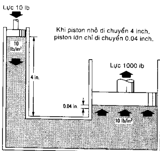
Hình 7-27. Áp suất thủy lực thay đổi. Lực 20 pound có thể nâng 1000 pound, nhưng chú ý khoảng cách di chuyển của cả hai lực và đối tượng chuyển động.
