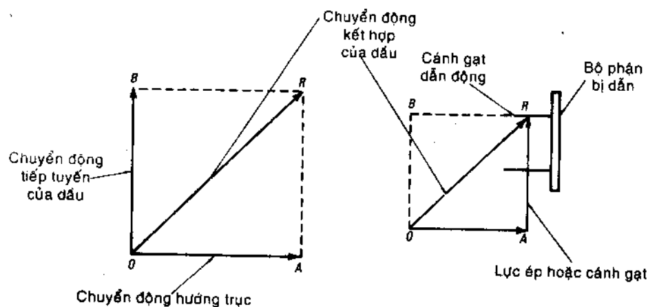
Hình 7-9. Động dầu thủy lực tổng hợp từ chuyển động tiếp tuyến và hướng trục (trái); gia tốc tiếp tuyến tạo moment có khuynh hướng quay cánh gạt bộ phận bị dẫn (phải).
