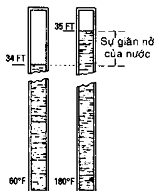
Hình 1-25. Sự gia tăng tầm dâng lý thuyết cực đại theo sự gia tăng nhiệt độ nước.
