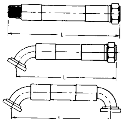
Hình 13-3. Phương pháp đo chiều dài cụm ống.
