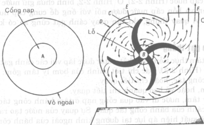
Hình 2-4. Các chi tiết cơ bản của bơm ly tâm gồm vỏ ngoài (trái) và mặt cắt bơm ly tâm, thường được gọi là bơm xoắn ốc do hình dạng vỏ bơm.
