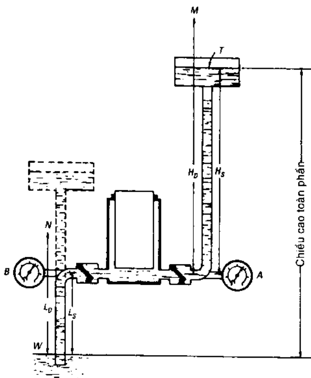
Hình 3-16. Cột động hoặc cột tổng đối với máy bơm.
