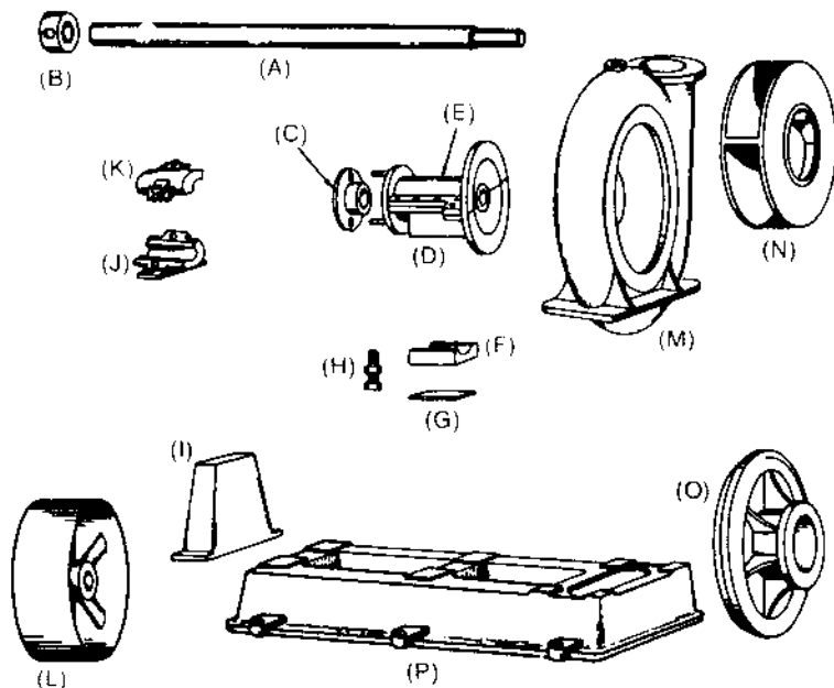
Hình 2-23. Các chi tiết của bơm ly tâm một cấp truyền động đai. Các chi tiết được minh họa là: (A) trục; (B) vành ti trục; (C) mặt xích ổ trục; (D) ổ trục (nửa dưới); (E) ổ trục (nửa trên); (F) ổ trục, đồng; (G) ổ trục, miếng chêm đồng; (H) ổ trục, vít chỉnh đồng; (I) giá đỡ ổ trục; (J) ổ đỡ; (K) nắp ổ đỡ; (L) bánh đai; (M) vỏ bơm; (N) bánh công tác; (O) đĩa bơm và (P) tâm đế.
