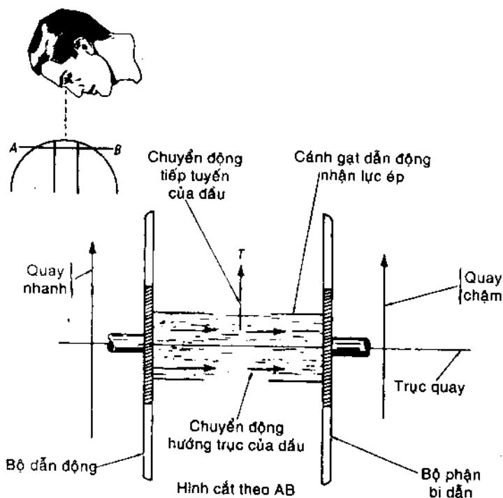
Hình 7-8. Sơ đồ mặt cắt có một phần vành cánh gạt liên kế bị cắt bỏ (trên đường AB ở bên trái phía trên), minh họa chuyển động hướng trục A và chuyển động tiếp tuyến T của dầu thủy lực.
