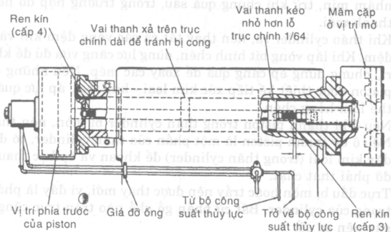
Hình 9-18. Lắp đặt thiết bị măm cặp trên máy.
