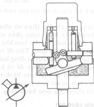
Hình 3-10. Bơm piston hướng trục dung tích biến thiên với cam hoặc vấu nghiêng để điều khiển lưu lượng phân phối của bơm.
