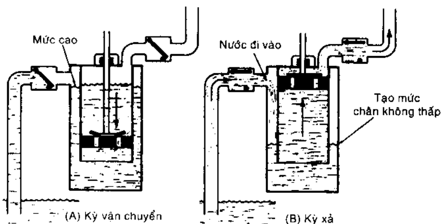
Hình 4-17. Chu trình làm việc hai kỳ của bơm xiphông (tự mồi).
