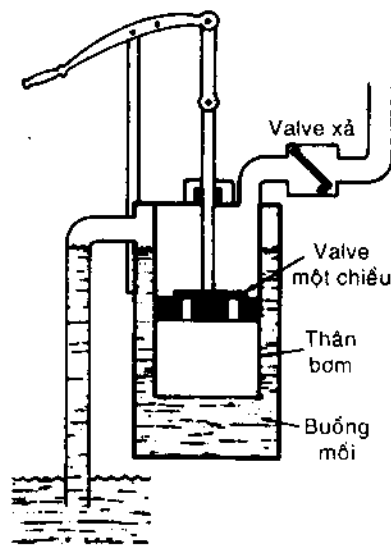
Hình 4-16. Kết cấu cơ bản của bơm xiphông (tự mồi).
