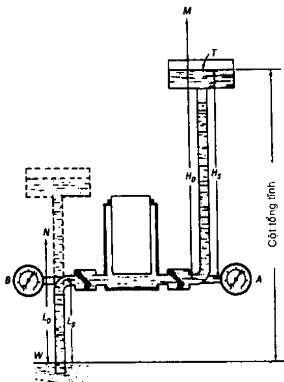
Hình 4-20. Phương pháp đo cột nước tĩnh và cột nước động, cột áp tĩnh và cột áp động, cột tổng tĩnh và cột tổng động.
