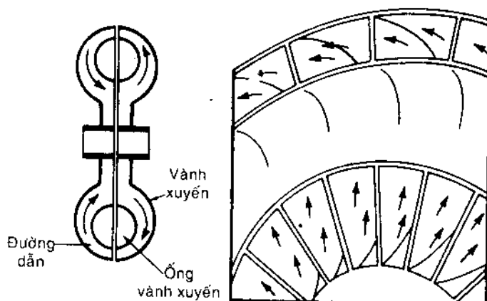
Hình 7-15. Sơ đồ minh họa sự tuần hoàn dầu thủy lực trong bộ dẫn động và bộ phận bị dẫn (trái); Sự tuần hoàn dầu trong rotor được minh họa thêm (phải).
