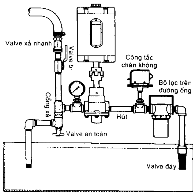
Hình 3-14. Lắp đặt bơm bánh răng.
