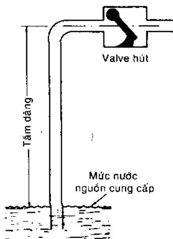
Hình 1-12. Điểm đo chính xác cột áp và tầm dâng.
