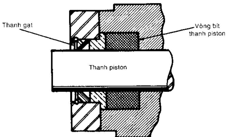
Hình 9-6. Thanh gạt bằng kim loại dùng để gạt các căn cứng trên thanh piston.
