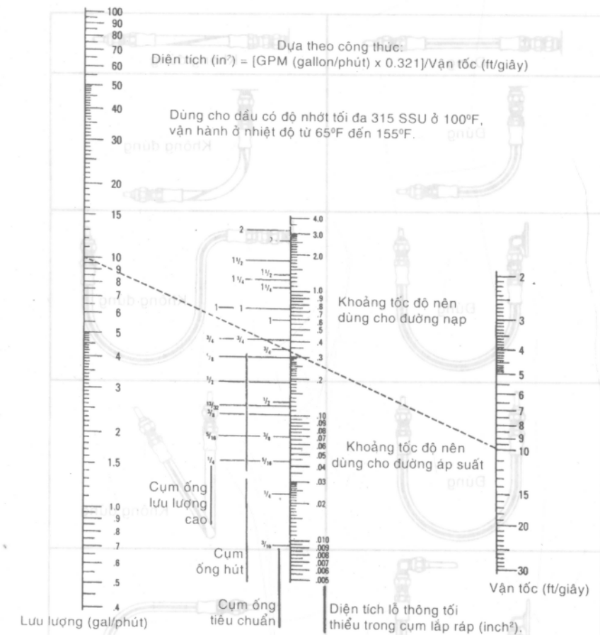
Hình 13-5. Phương pháp xác định kích cỡ ống chính xác.
