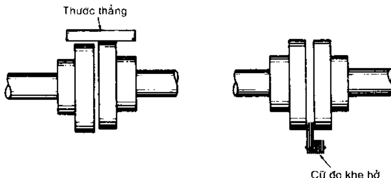
Hình 2-25. Dùng thước thẳng và bộ cử đo khe hở kiểm tra sự thẳng hàng giữa bơm và trục dẫn động.
