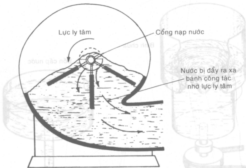
Hình 2-3. Bơm ly tâm minh họa nguyên lý lực ly tâm.
