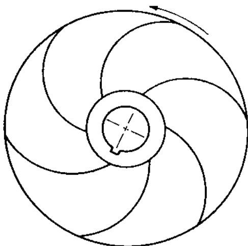
Hình 2-26. Chiều quay của bánh công tác trên bơm ly tâm.
