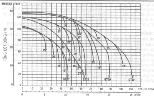
Hình B-11. Bơm ly tâm tự mỗi Irri-Gator, mẫu GT (đặc tính hiệu suất).
