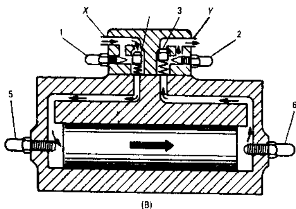
Hình 11-10. Hai nêm điều chỉnh được dùng trên valve thủy lực vận hành dẫn hướng.
