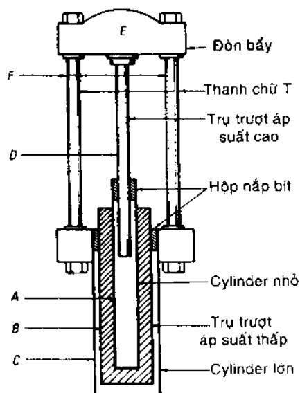
Hình 6-6. Kết cấu cơ bản của thiết bị tăng áp suất hoặc bộ tăng cường là loại bộ tích lũy vi sai. Bộ tăng cường là thiết bị thủy lực được dùng để chuyển đổi chất lỏng áp suất thấp thành áp suất cao.
