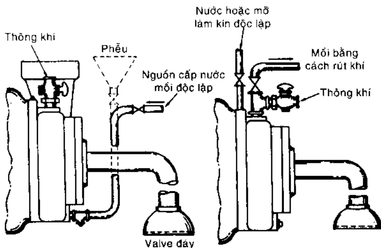
Hình 2-30. Ống cho hệ thống môi sử dụng nguồn nước môi độc lập (trái) và môi bằng rút khí (phải).
