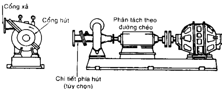
Hình 2-17. Bơm ly tâm thông dụng. Vỏ ngoài phân chia theo đường chéo cho phép dễ tháo các chi tiết bên trong mà không làm xáo trộn phần xả của ống hút.
