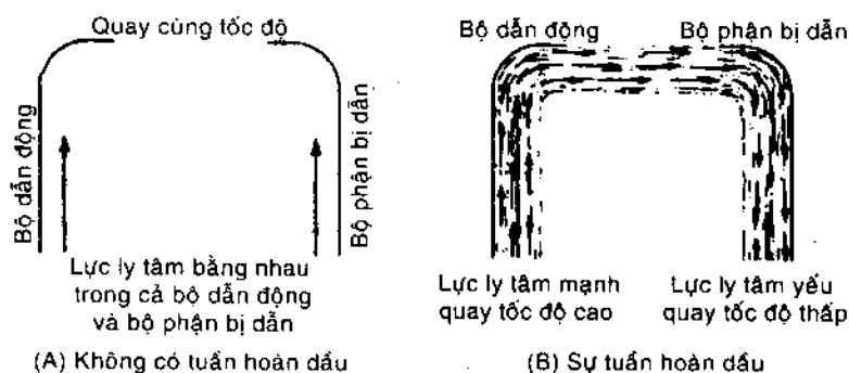
Hình 7-4. Nguyên nhân cơ bản của sự tuần hoàn dầu trong bộ dẫn động thủy lực. Lực ly tâm trong bộ dẫn động và bộ phận bị dẫn ngược nhau, dầu thủy lực không tuần hoàn trừ khi lực ly tâm của một trong các bộ phận này lớn hơn, do tăng tốc độ quay.
