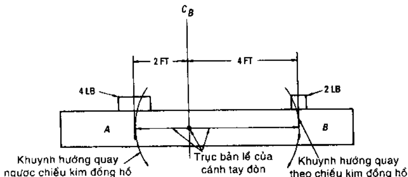
Hình 1-19. Sự cân bằng quy chiếu theo tâm nối ( C_B ) và sự phân bố các khối nặng.
