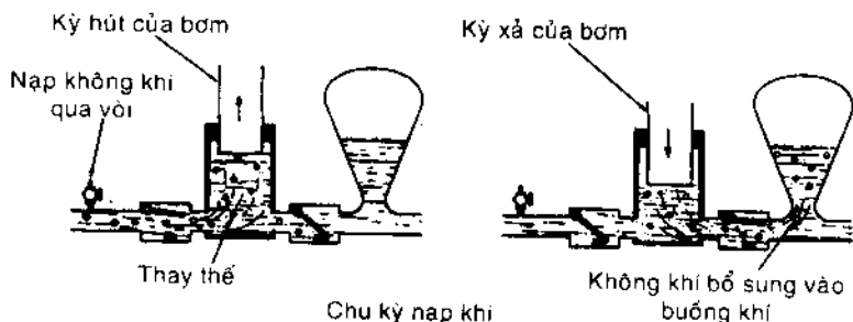
Hình 6-17. Phương pháp cung cấp thêm không khí để bù cho phần khí bị nước hấp thu.
