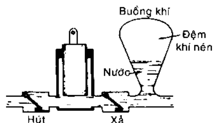
Hình 6-15. Tương quan vị trí giữa buồng không khí và bơm trong hệ thống nước.
