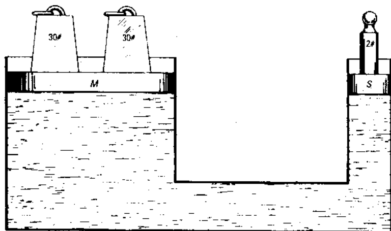
Hình 1-6. Áp lực do chất lỏng tác dụng trên bề mặt tỷ lệ với diện tích bề mặt.
