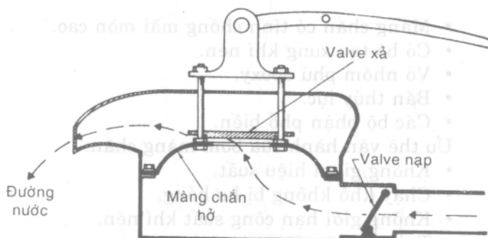
Hình 5-11. Những chi tiết cơ bản trong bơm màng chắn hở.
