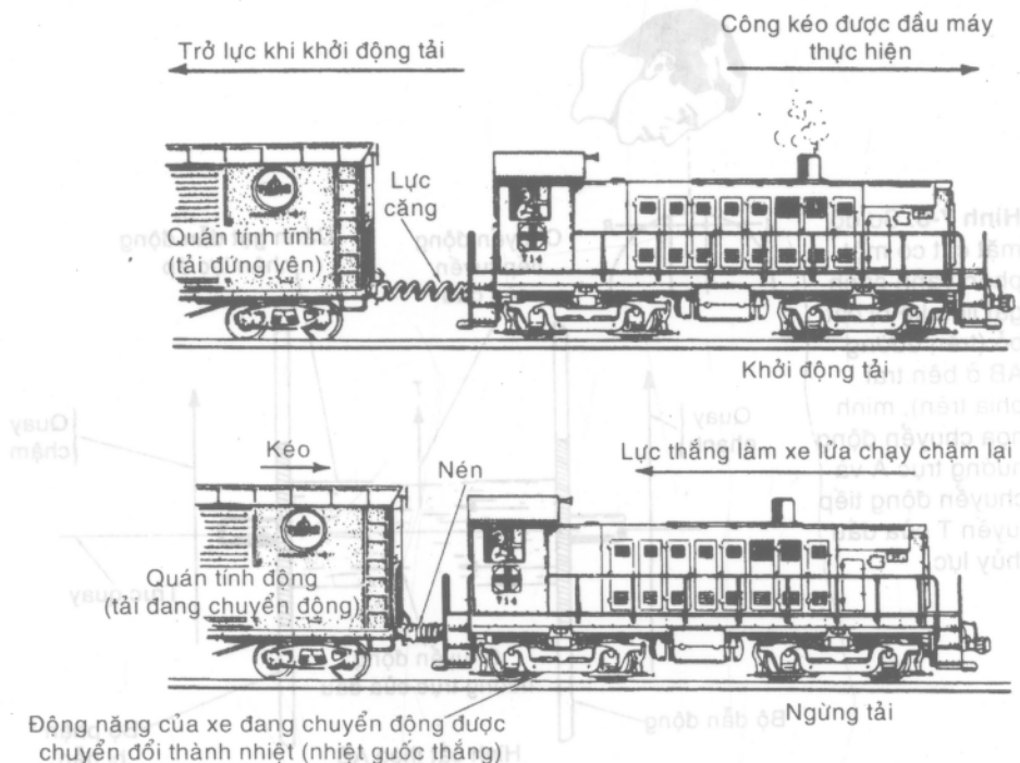
Hình 7-10. Động năng. Đầu máy cần công để bắt đầu kéo tải (trên) và công cần thiết để xe đang di chuyển dừng tải, có khuynh hướng duy trì chuyển động (dưới). Chú ý, công cần để dừng tải được biến đổi thành nhiệt quoc thẳng.
