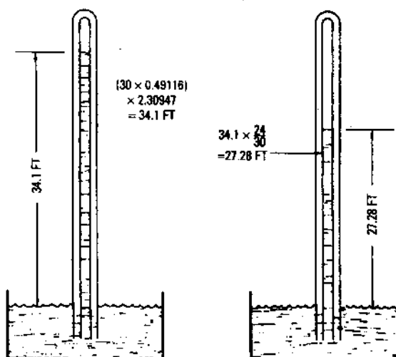
Hình 1-15. Tấm dăng cực đại của nước ở nhiệt độ chuẩn (62°F) khi áp suất phong vũ biểu là 30 inch (trái) và 24 inch (phải).
