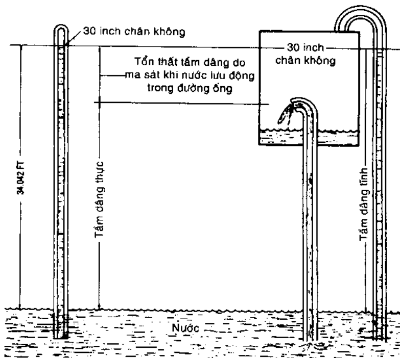
Hình 1-22. Tầm dâng lý thuyết (trái) đối với bơm, tương ứng với tầm dâng tính ở số đo phong vũ biểu đã cho, nhưng không đạt được trong thực tế; tầm dâng động (phải) là tầm dâng thực tế, cộng thêm trở lực ma sát.
