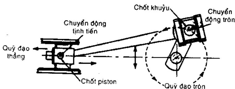
Hình 4-1. Sự khác nhau cơ bản giữa chuyển động tịnh tiến (trái) và chuyển động tròn (phải).
