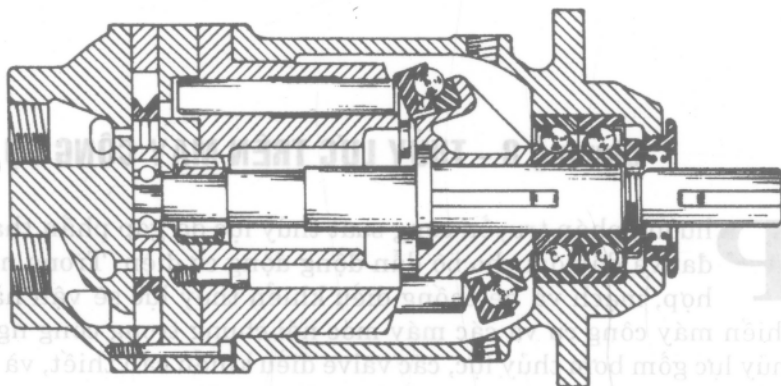
Hình 8-2. Kết cấu chi tiết của piston và thanh truyền trong động cơ thủy lực.
