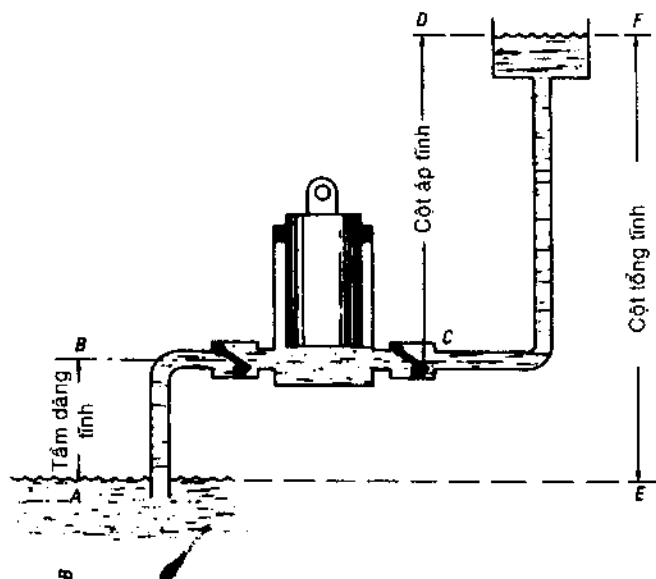
Hình 1-26. Cột tổng tĩnh (EF) là tầm dâng tĩnh (AB) cộng với cột áp tĩnh (CD), thẳng đứng từ mức nước nguồn đến điểm xả hoặc mặt thoáng của nước trong bồn chứa.
