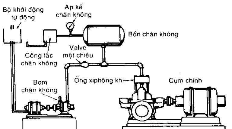
Hình 2-29. Hệ thống môi tự động, sử dụng bơm chân không làm bình dự trữ để duy trì việc môi bơm chính.
