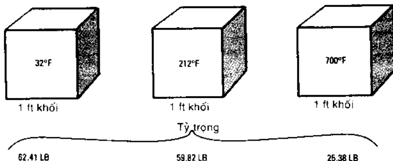
Hình 1-40. Tỷ trọng nước ở các nhiệt độ khác nhau. Tỷ trọng giảm khi nhiệt độ tăng.
