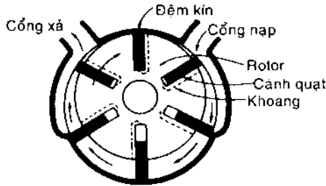
Hình 3-3. Chi tiết bơm cánh gạt quay.
