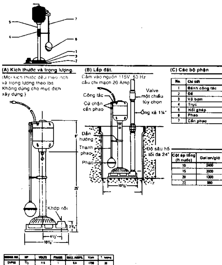
Hình 5-6. Đặc tính kỹ thuật chung đối với các bơm nước thải.
