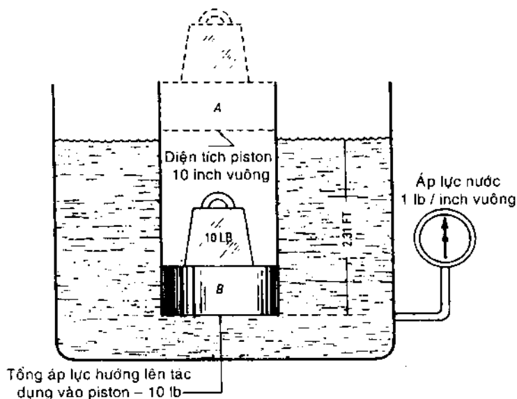
Hình 1-17. Sự minh họa độ nổi bằng cách nhúng cylinder chứa piston không ma sát vào nước.
