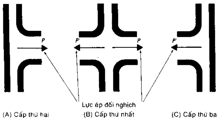
Hình 2-13. Cân bằng tự nhiên đạt được ở bơm ba cấp nhờ hai bánh công tác hống hút đơn đối nhau (trái và phải) và một bánh công tác hống hút kép (ở giữa).
