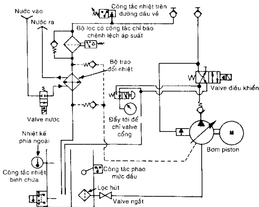
Hình 7-31. Mạch Quietpak do Hydrex sản xuất.
