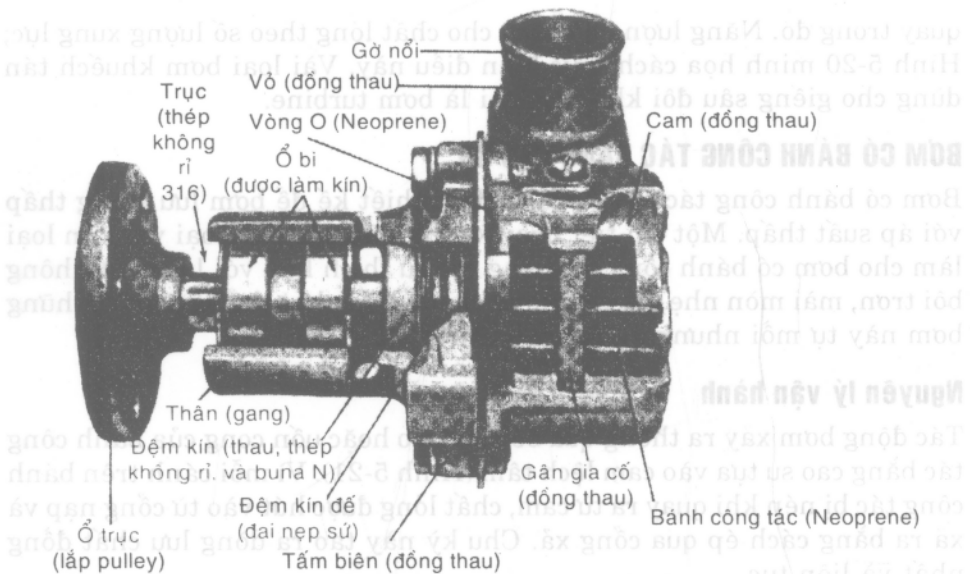
Hình 5-22. Bơm làm mát động cơ tàu thủy, vật liệu đồng thau. Minh họa các đặc điểm thiết kế và vật liệu chi tiết.
