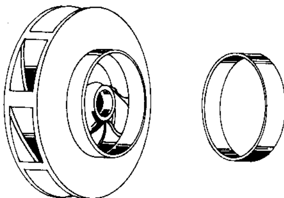
Hình 2-18. Bánh công tác hòng hút kép loại kín và vòng bù độ mòn. Vải chất lỏng cần bánh công tác được làm bằng các hợp kim đặc biệt như crôm, monel, nickel,...
