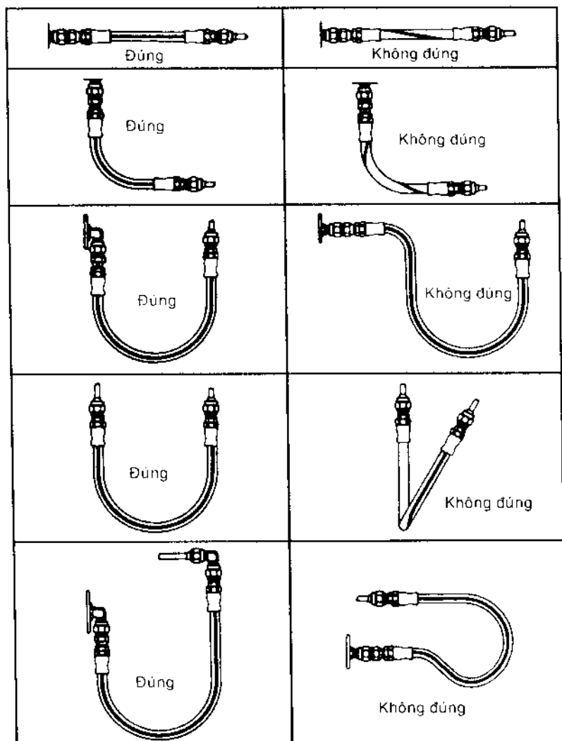
Hình 13-6. Lắp đặt cụm ống mềm.
