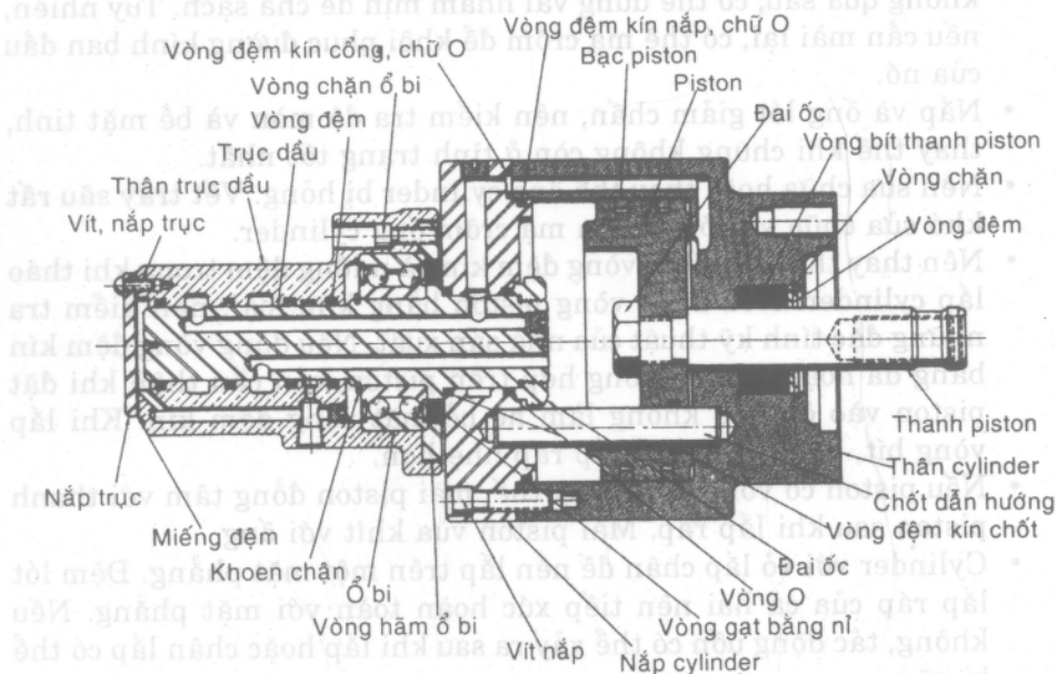
Hình 9-16. Các chi tiết của cylinder thủy lực quay.
