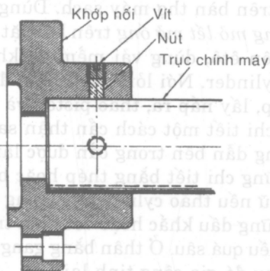
Hình 9-17. Khớp nối cho cylinder quay.
