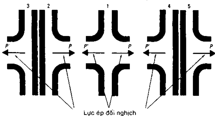
Hình 2-14. Cân bằng tự nhiên đạt được ở bơm năm cấp nhờ một bộ gồm hai cặp bánh công tác lưng đối lưng hống hút đơn đối nhau (trái và phải) và một bánh công tác hống hút kép (chính giữa).
