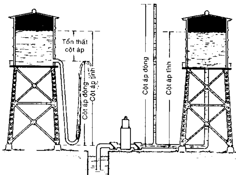
Hình 1-11. Cột áp tĩnh và cột áp động
