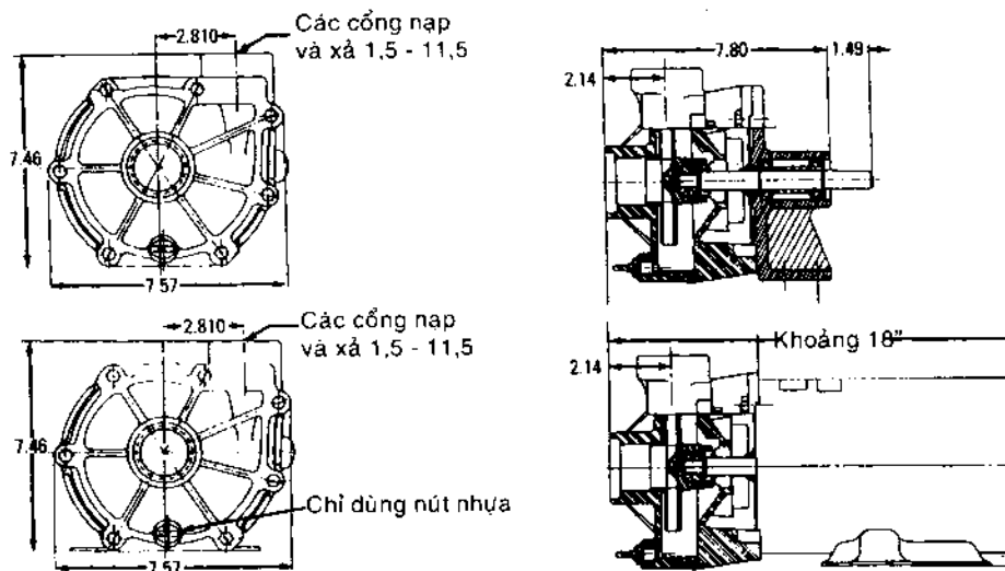
Hình 2-37. (a) Hình chiếu bơm kiểu có đế; (b) Hình chiếu bơm kiểu lắp ở đầu.
