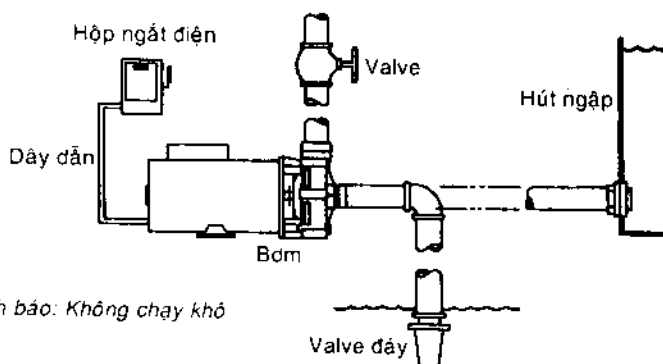
Hình 2-35. Nối điện cho bơm ly tâm.
