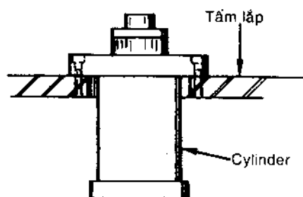
Hình 9-10. Lắp mặt bích đảo ngược của cylinder thủy lực cho những ứng dụng ép.
