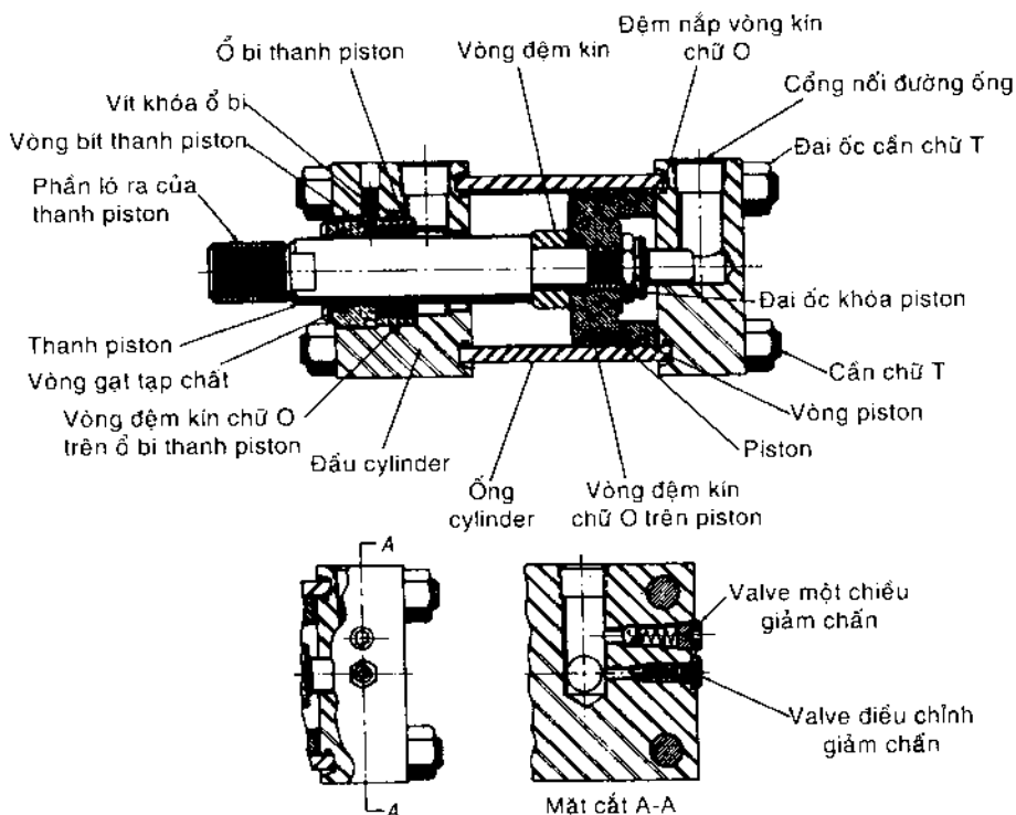
Hình 9-5. Các chi tiết của cylinder thủy lực chịu tải nặng.
