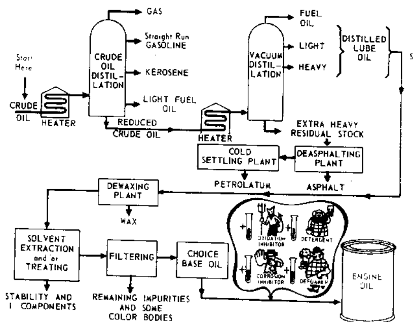
Hình 26: Quá trình lọc dầu bôi trơn
