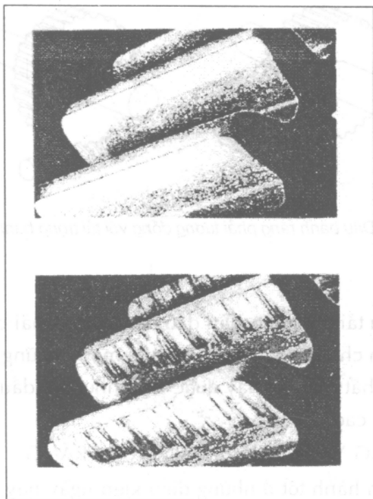
Hình 54: Mài mòn bánh răng bình thường và mài mòn trầy xước
