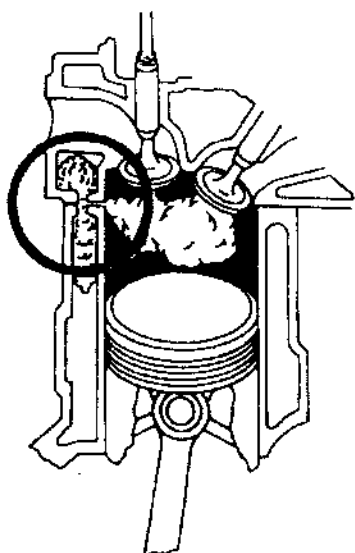
Hình 65: Gas cháy rò vào trong hệ thống làm mát có thể làm nếu chất tải nhiệt và cũng gây ra nổi bọt, quá nóng và chảy tràn.
