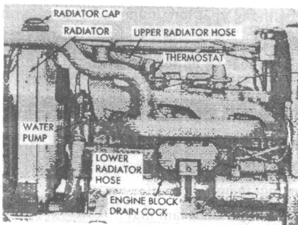
Hình 62: Hệ thống làm nguội động cơ.
