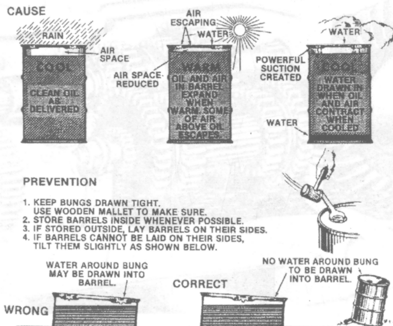
Hình 52: Các quy trình kỹ thuật cất giữ giúp ngăn ngừa nhiễm bẩn ở dầu
