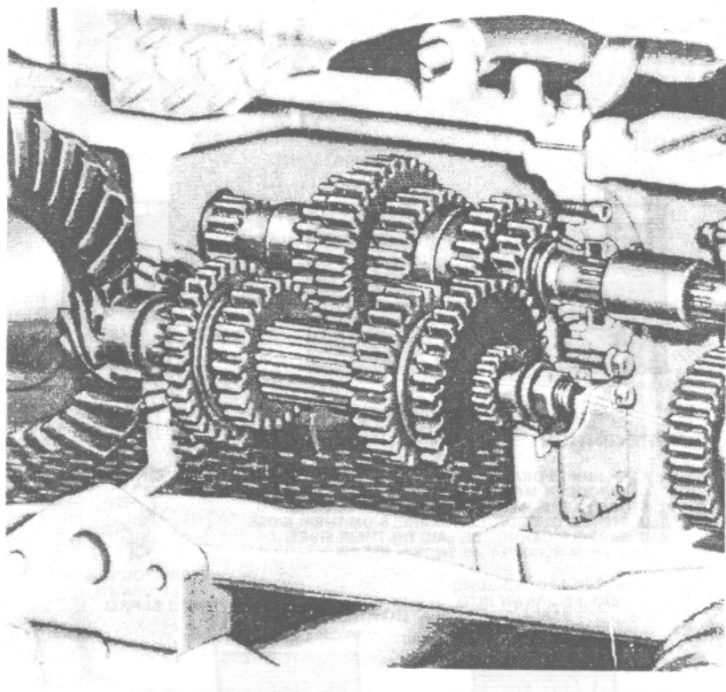
Hình 53: Bộ vi sai truyền động hoạt động trong dung dịch dầu
