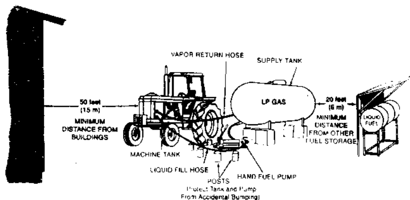
Hình 22: Vị trí an toàn để thùng chứa Gaz LP liên quan đến nhà ở và nơi chứa nhiên liệu khác
