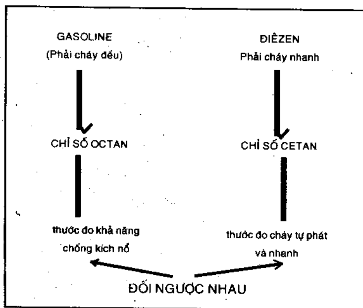
Hình 12: Sự khác nhau giữa chỉ số octan (xăng) và cetan (điêzen)
