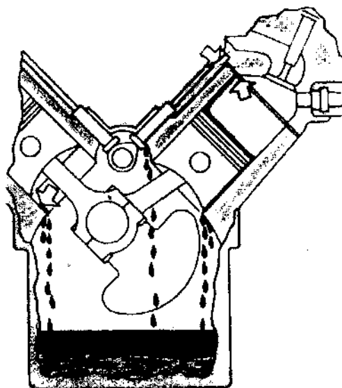
Hình 72: Chất tải nhiệt rò vào trong hộp cacte có thể làm hỏng việc bôi trơn.
