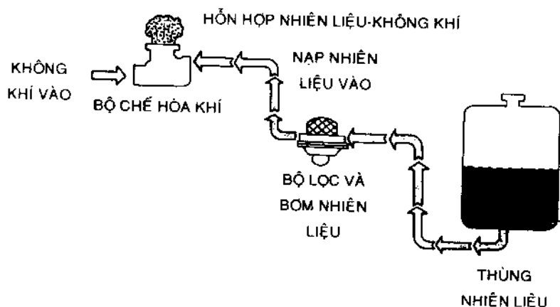
Hình 6: Hệ thống nhiên liệu xăng
