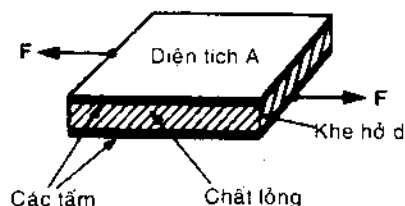
Hình 6-9 Định nghĩa khoa học về độ nhớt dưới dạng lực trượt.
