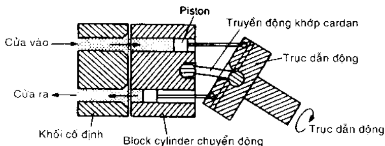
Hình 2-15 Bơm piston trục lệch
