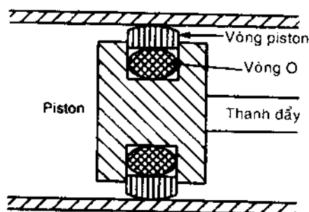
Hình 5-21 Kết hợp vòng piston và vòng đệm kín O (không theo tỉ lệ).
