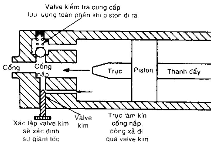
Hình 5-10 Giảm chấn cylinder
