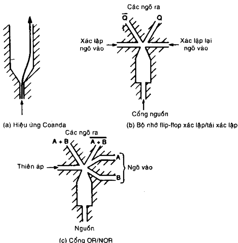
Hình 7-32 Logic học chất lỏng.
