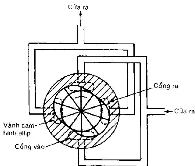
(b) Bơm cánh gạt cân bằng
