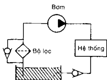
(d) Bảo vệ bộ lọc bị nghẹt và khóa sự hút
