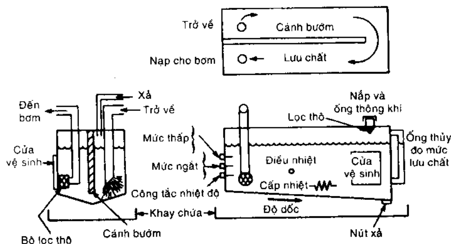
Hình 6-1 Kết cấu bình chứa dầu thủy lực.
