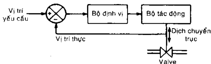
Hình 7-21 Bộ định vị valve.
