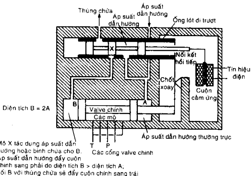
Hình 4-40 Valve trợ động hai cấp
