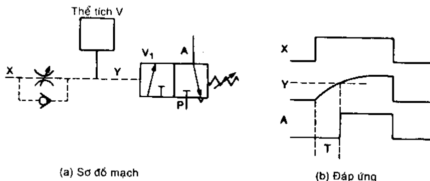
Hình 7-28 Trì hoãn thời gian (xem kết cấu trên Hình 4-28)
