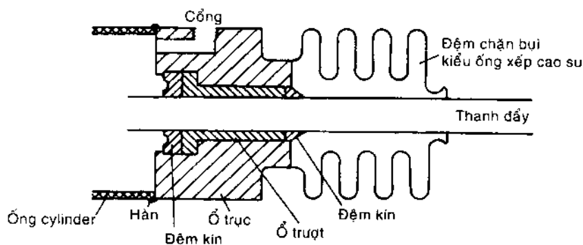
(a) Mặt cắt nắp ổ trục
