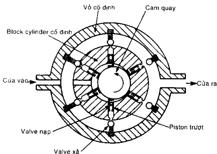
Hình 2-12 Bơm piston hướng kính
