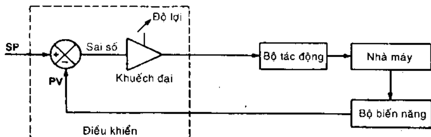
Hình 7-7 Bộ điều khiển tỷ lệ
