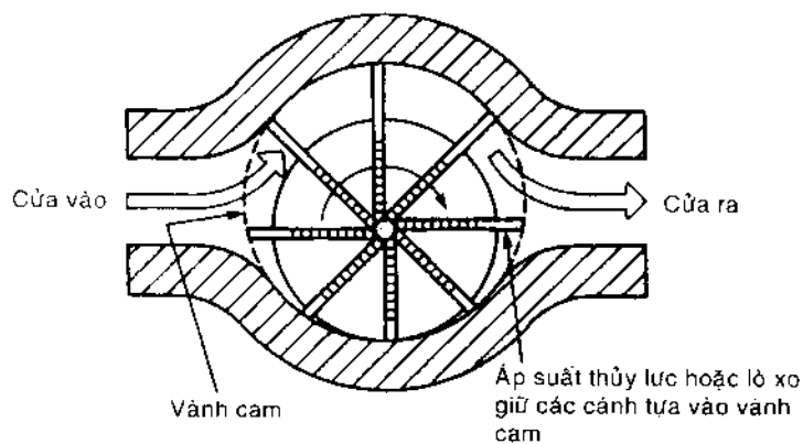
(a) Bơm cánh gạt lệch tâm
