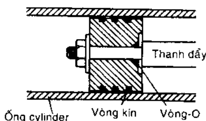
(c) Vòng đệm kín và vòng-O
