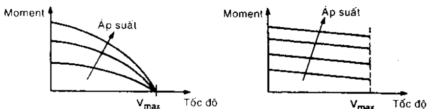
Hình 5-23 Đường cong moment/tốc độ của bộ tác động quay.
