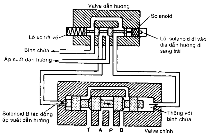
(a) Kết cấu: Điện năng tác động vào solenoid đẩy cuộn dẫn hướng về bên trái. Điều này tác dụng áp suất dẫn hướng lên đầu bên trái của ống cuộn chính, đẩy ống cuộn sang phải để nối các cổng P và B
