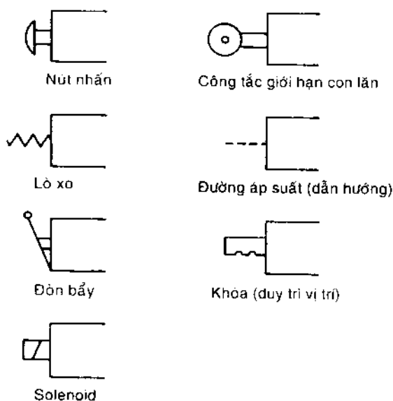
(a) Các ký hiệu tác động
