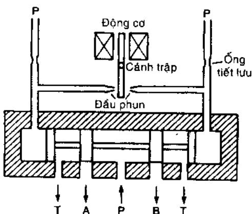
Hình 4-42 Valve trợ động cánh trập
