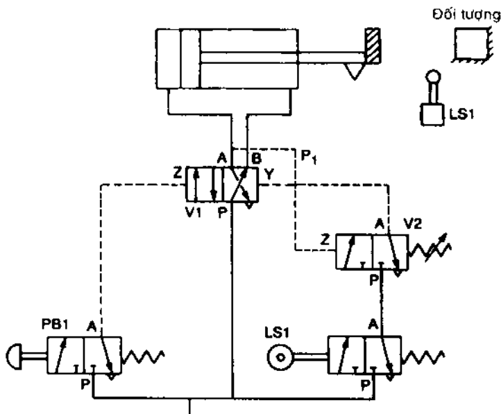
Hình 7-29 Ứng dụng valve chuỗi thứ tự.
