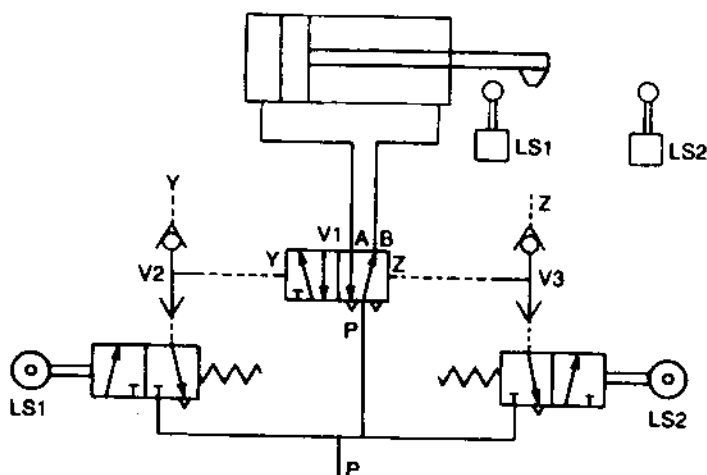
Hình 7-27 Ví dụ về chuỗi thứ tự; thanh piston đảo động giữa LS 1 và LS 2 .
