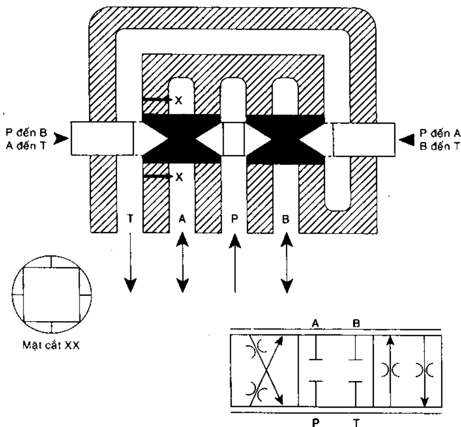
Hình 4-30 Cấu trúc và ký hiệu valve cân bằng. Khi được dùng với cylinder có tỷ số giữa đường kính trong của cylinder và phần vành khuyên là 2:1, một nửa số khía định lượng V sẽ ở trên một trong các mô P.
