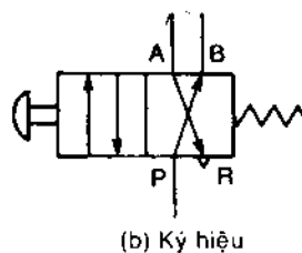
Hình 4-11 Valve đĩa 4/2
