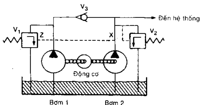
(a) Bơm tổ hợp
