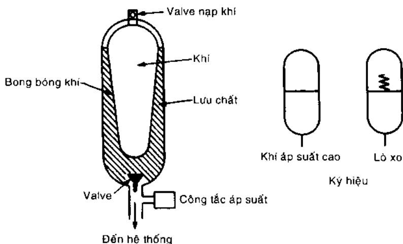
Hình 6-4 Bộ tích lũy.
