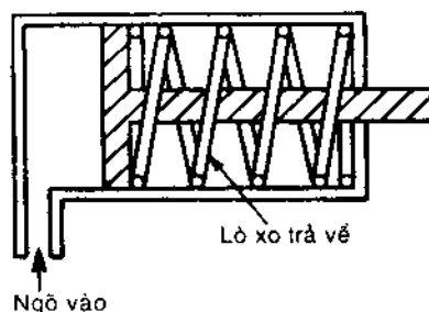
Hình 5-5 Cylinder tác động đơn
