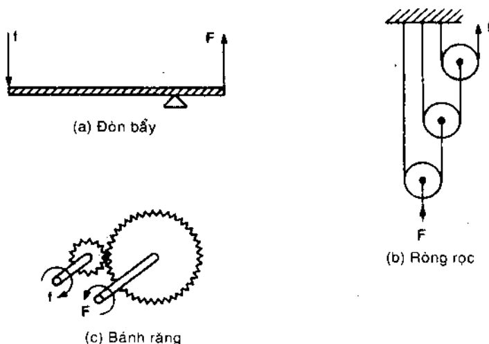
Hình 1-11 Đồ lợi công cơ học, lực f nhỏ ở đầu vào tạo ra lực F lớn ở đầu ra.
