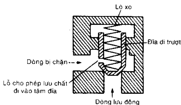
(b) Van điều khiển thẳng góc
