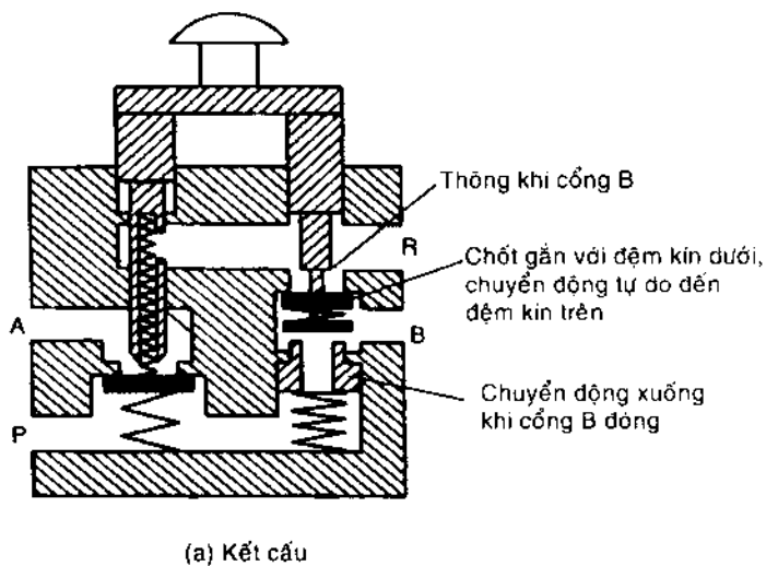
Hình 4-10 Valve đĩa 3/2
