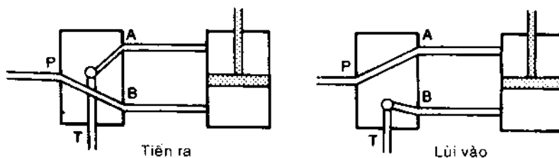
Hình 4-2 Vận hành bên trong valve.
