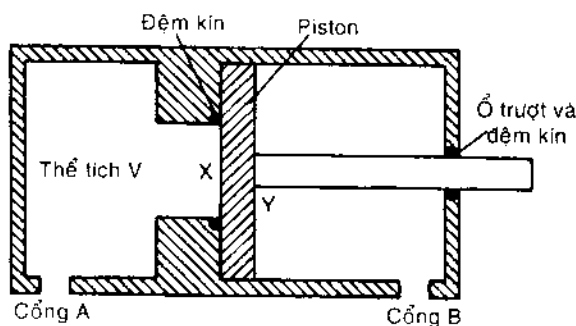
Hình 5-13 Cylinder dập
