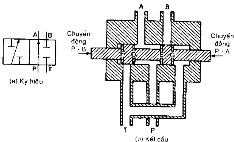
Hình 4-12 Valve ống cuộn hai ngã
