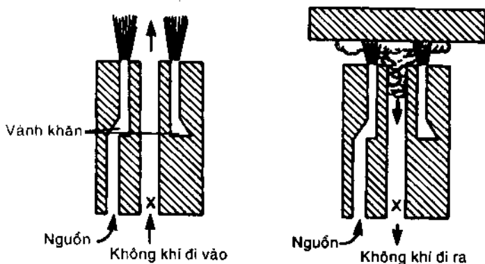
Hình 7-30 Công tác phản xạ gần.
