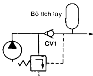
(b) Bộ tích lũy
