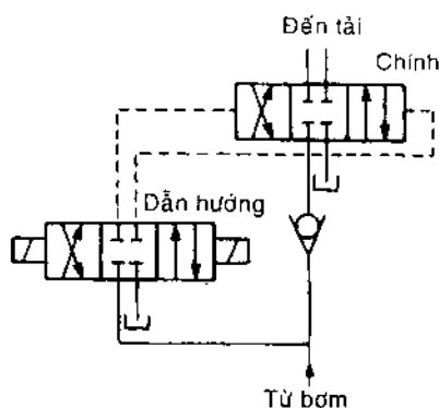
(c) Cung cấp áp suất dẫn hướng
