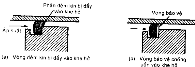
Hình 5-20 Vòng bảo vệ đệm kín
