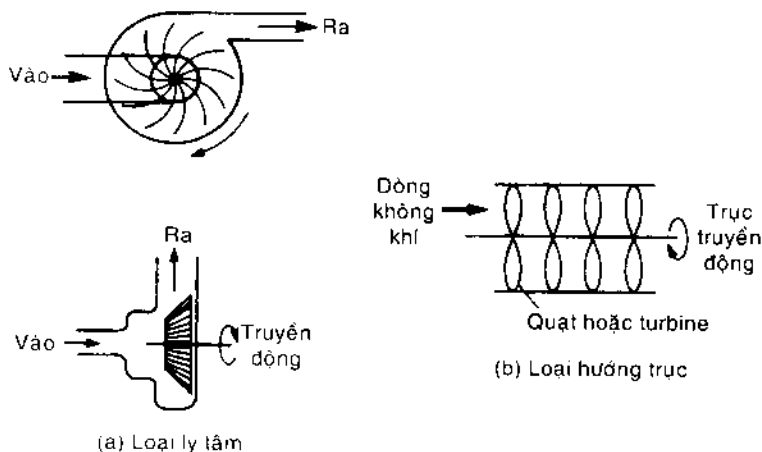
Hình 3-12 Loại máy nén không tịnh tiến (quạt thổi)
