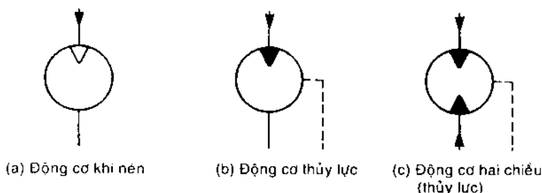
Hình 5-25 Ký hiệu bộ tác động quay
