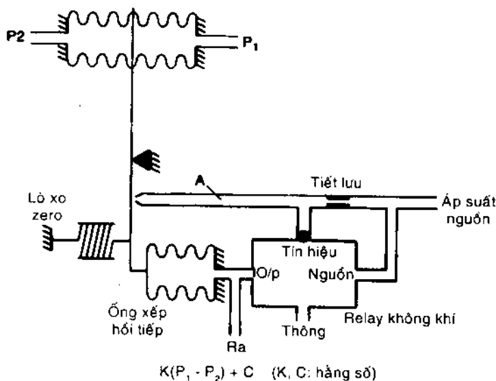
Hình 7-6 Nguyên lý cân bằng lực.
