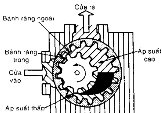
(a) Bơm bánh răng trong
