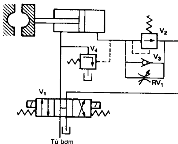
Hình 5-47 Mạch giải nén có điều khiển
