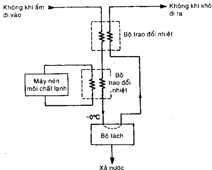
Hình 3-20 Bộ sấy kiểu làm lạnh.
