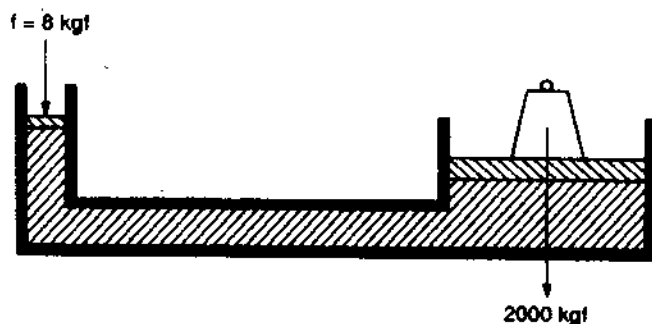
Hình 1-10 Lợi về công
