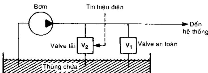
Hình 2-18 Valve tải.
