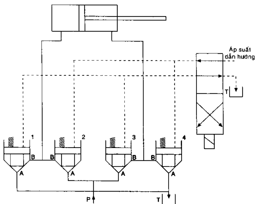
Hình 4-48 Điều khiển hướng với bốn valve hộp. Cylinder sẽ kéo dài hoặc thu lại hoàn toàn. Nếu dùng hai valve solenoid, một để mở và một để đóng, cylinder có thể duy trì vị trí trung gian.
