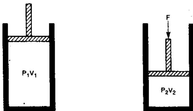
Hình 1-24 Định luật Boyle
