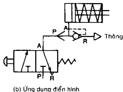
Hình 4-26 Valve xả nhanh
