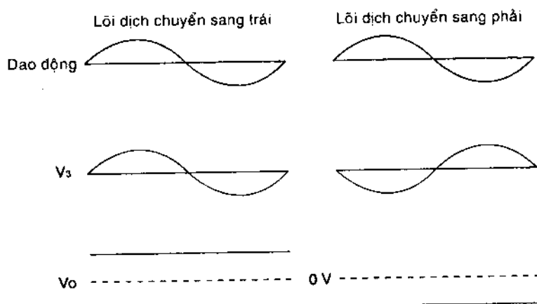
Hình 4-32 Công dụng của LVDT là điều khiển vị trí của valve ống cuộn. LVDT có thể nối với ống cuộn dẫn hướng hoặc ống cuộn chính. (a) Mạch LVDT và chỉnh lưu nhảy pha. (b) Tín hiệu ngõ ra khi lõi dịch chuyển qua trái và phải.
