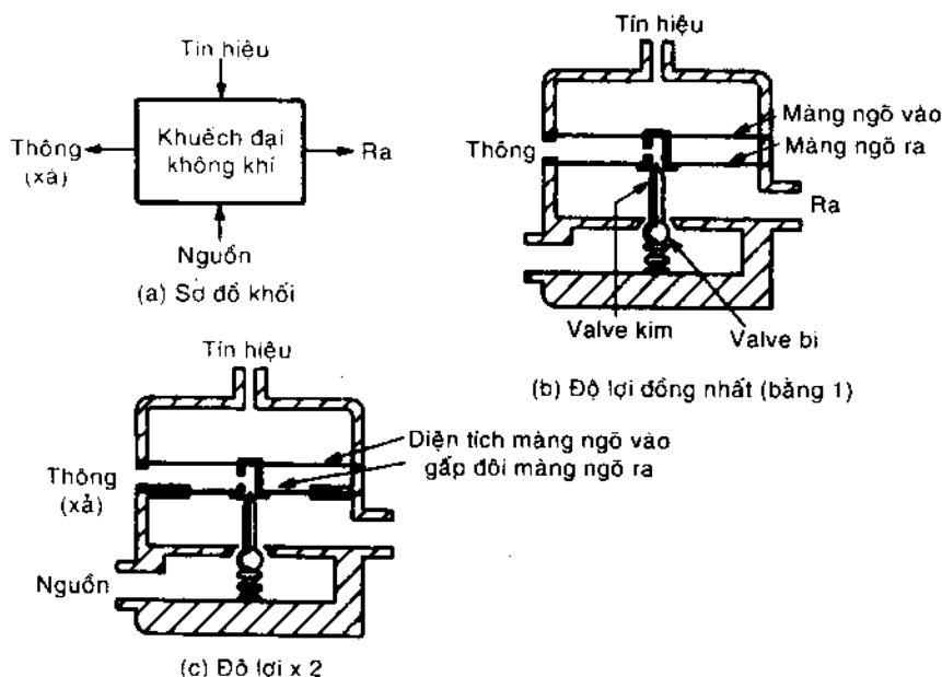
Hình 7-4 Bộ tăng lưu lượng hoặc bộ khuếch đại khí.
