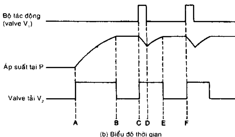
Hình 6-3 Hệ thống với bộ tích lũy
