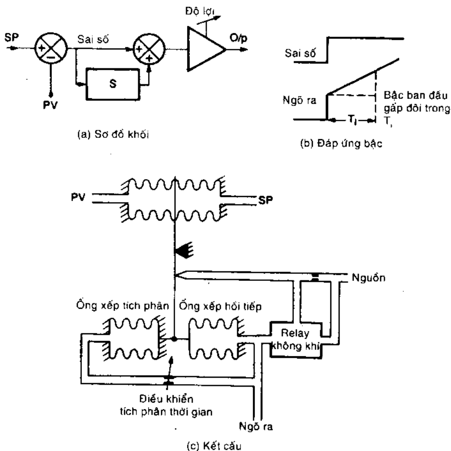
Hình 7-8 Bộ điều khiển tỉ lệ tích phân (P+I).
