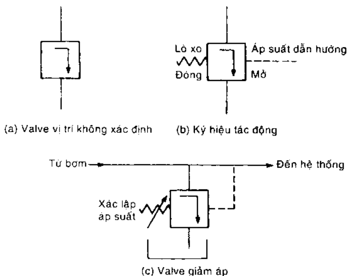
Hình 4-8 Ký hiệu valve vị trí không xác định
