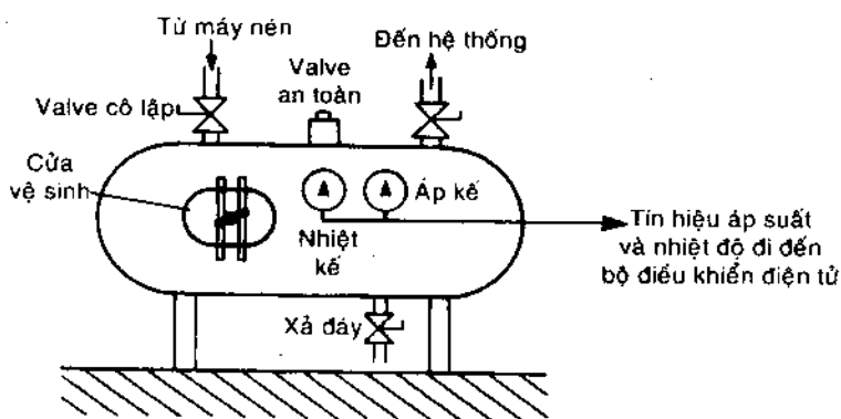
Hình 3-13 Bình chứa khí nén.
