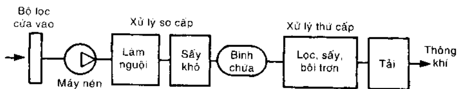
Hình 3-18 Ba giai đoạn xử lý không khí.
