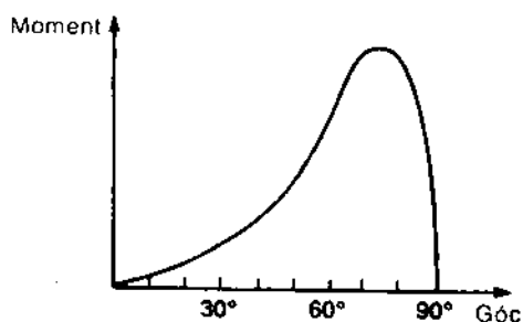
Hình 7-16 Moment trên valve bướm.
