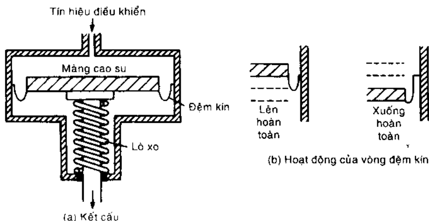
Hình 7-18 Bộ tác động sự cố hướng lên.
