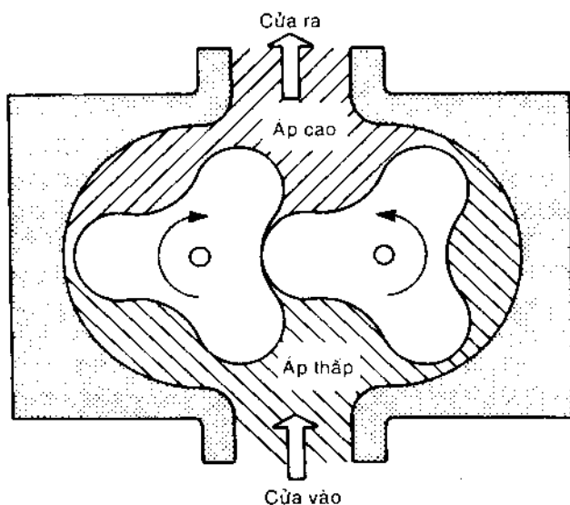
Hình 2-8 Bơm rotor (ba thủy)
