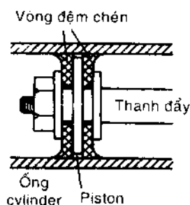
(b) Vòng đệm chén
