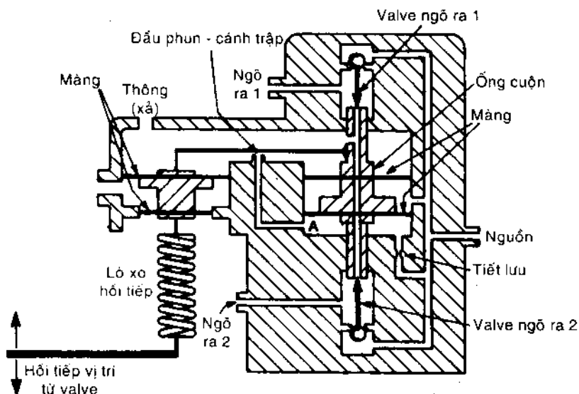
Hình 7-22 Bộ định vị valve cân bằng lực.
