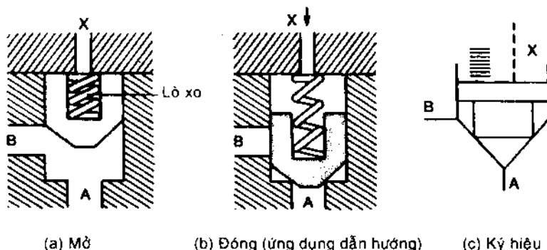
Hình 4-46 Valve logic kiểu hộp.
