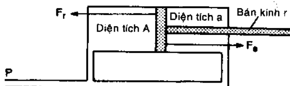
Hình 5-3 Áp suất tác dụng vào cả hai phía piston
