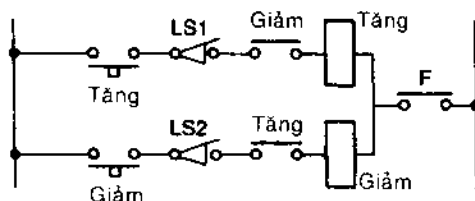
(a) Mạch điện
