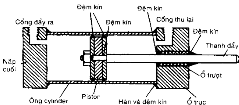
Hình 5-8 Kết cấu cylinder.
