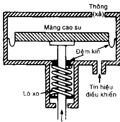
Hình 7-19 Bộ tác động sự cố hướng xuống
