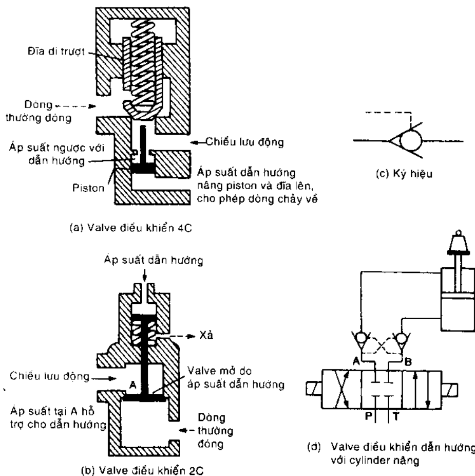
Hình 4-23 Valve điều khiển vận hành nhờ valve dẫn hướng
