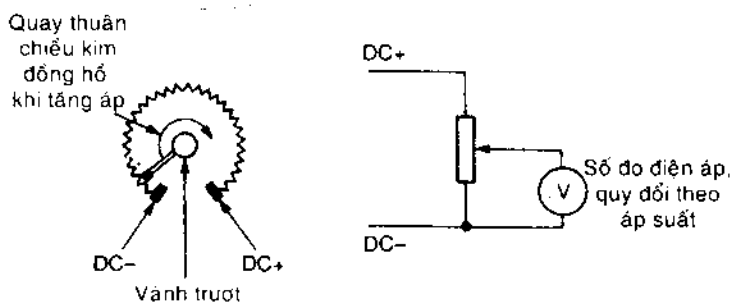
(b) Tín hiệu điện từ áp kế Bourdon
