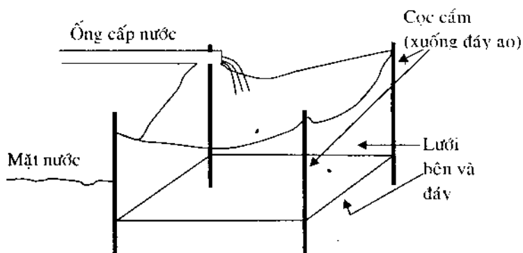
Hình 5b. – Bộng cấp nước và lưới lọc cá tạp
