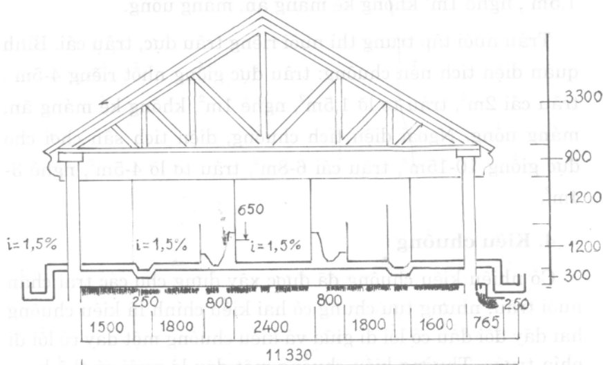
Kiểu chuồng hai dãy đối đầu có lối đi giữa (mặt cắt)
