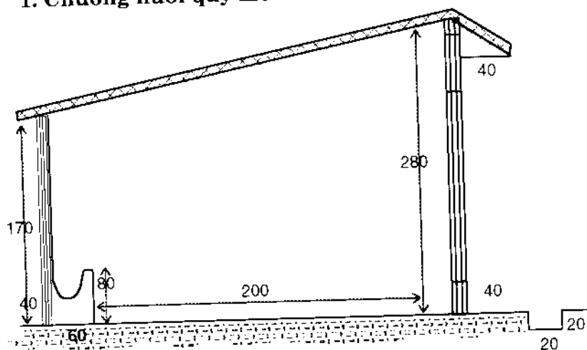
Chuồng 1 dây - Mặt cắt ngang Tiêu chuẩn 1 con bò: 3,5m 2 .
