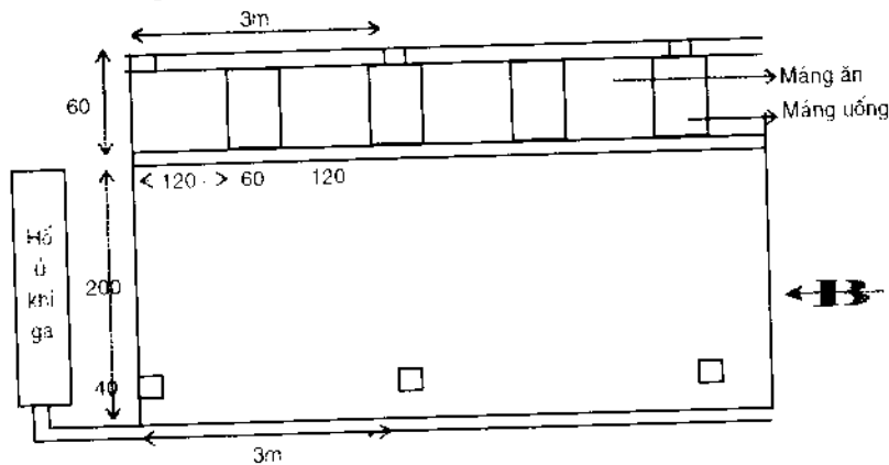
Chuồng 1 dây: Mặt bằng
