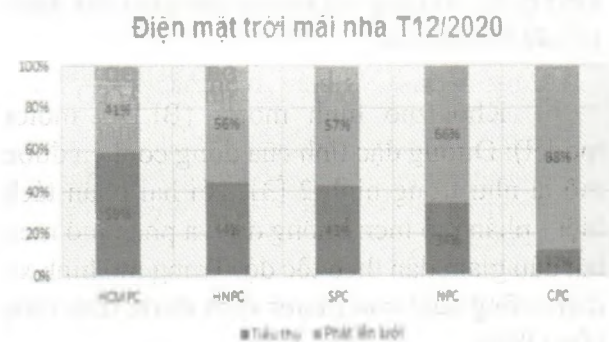
Hình 4. Tỷ lệ sản lượng ĐMTAM tiêu thụ và phát lên lưới tháng 12/2020 theo từng Tổng công ty
