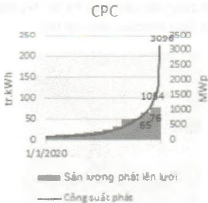
Hình 1. Sản lượng và công suất phát của các hệ thống ĐMTAP tại CPC trong năm 2020
