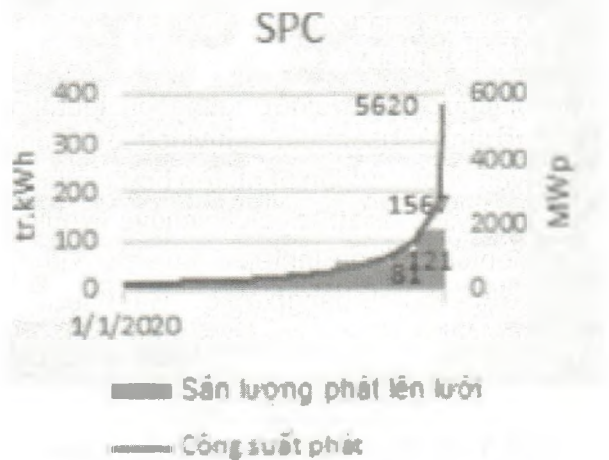
Hình 2. Sản lượng và công suất phát của các hệ thống ĐMTAP tại SPC trong năm 2020
