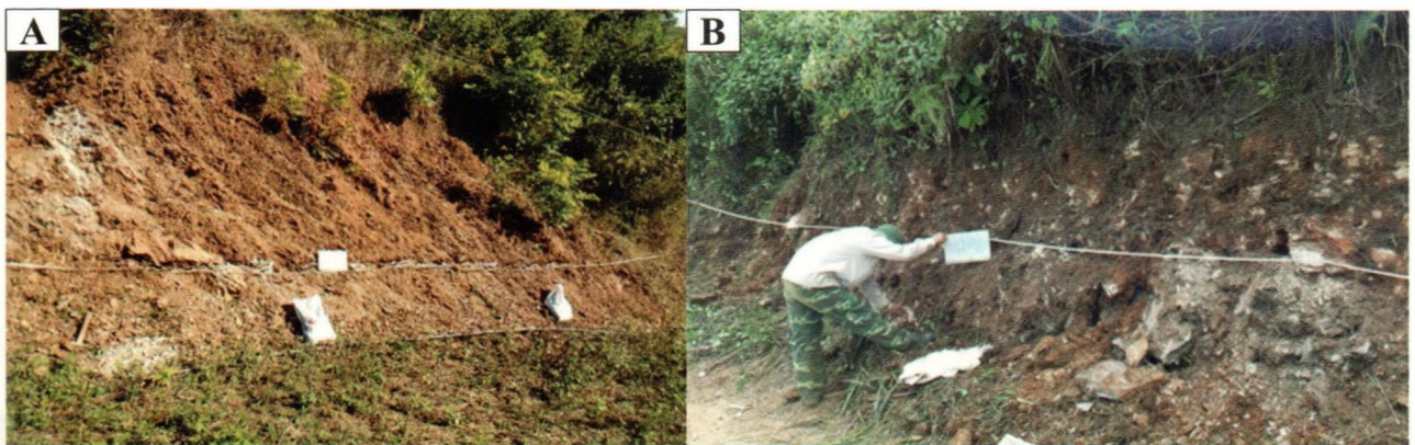
H.2. A-Điểm lộ quặng talc tại vết lộ VLN.370 (TQ.7) khu Bản Ngày; B-Điểm lộ quặng talc tại vết lộ VLH.236 (TQ.1) khu Bản Hua Ngáy [4]
