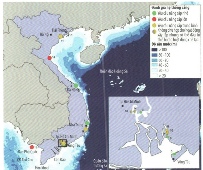
Hình 5. Hệ thống cảng hậu cần, bãi chế tạo, lắp ráp. Nguồn BVG, 2020.
