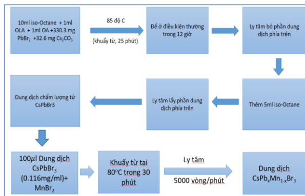
Hình 1. Sơ đồ quy trình chế tạo chấm lượng tử bán dẫn CsPbBr_3 pha tạp ion Mn^{2+}
