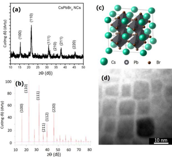
Hình 2. (a) phổ nhiễu xạ tia X, và (b) phổ chuẩn XRD, (c) mô hình cấu trúc tinh thể lập phương và (d) ảnh TEM của mẫu của mẫu CsPbBr 3 không pha tạp
