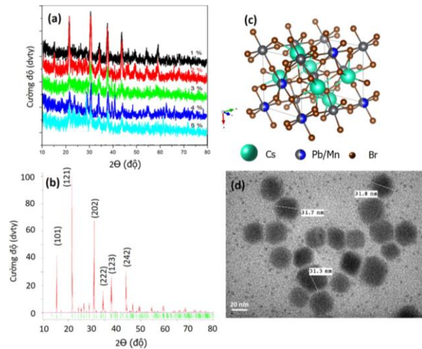
Hình 3. (a) phổ nhiễu xạ tia X, và (b) phổ chuẩn XRD, (c) mô hình cấu trúc tinh thể lập phương và (d) ảnh TEM của mẫu của mẫu CsPbBr 3 pha tạp Mn 2+
