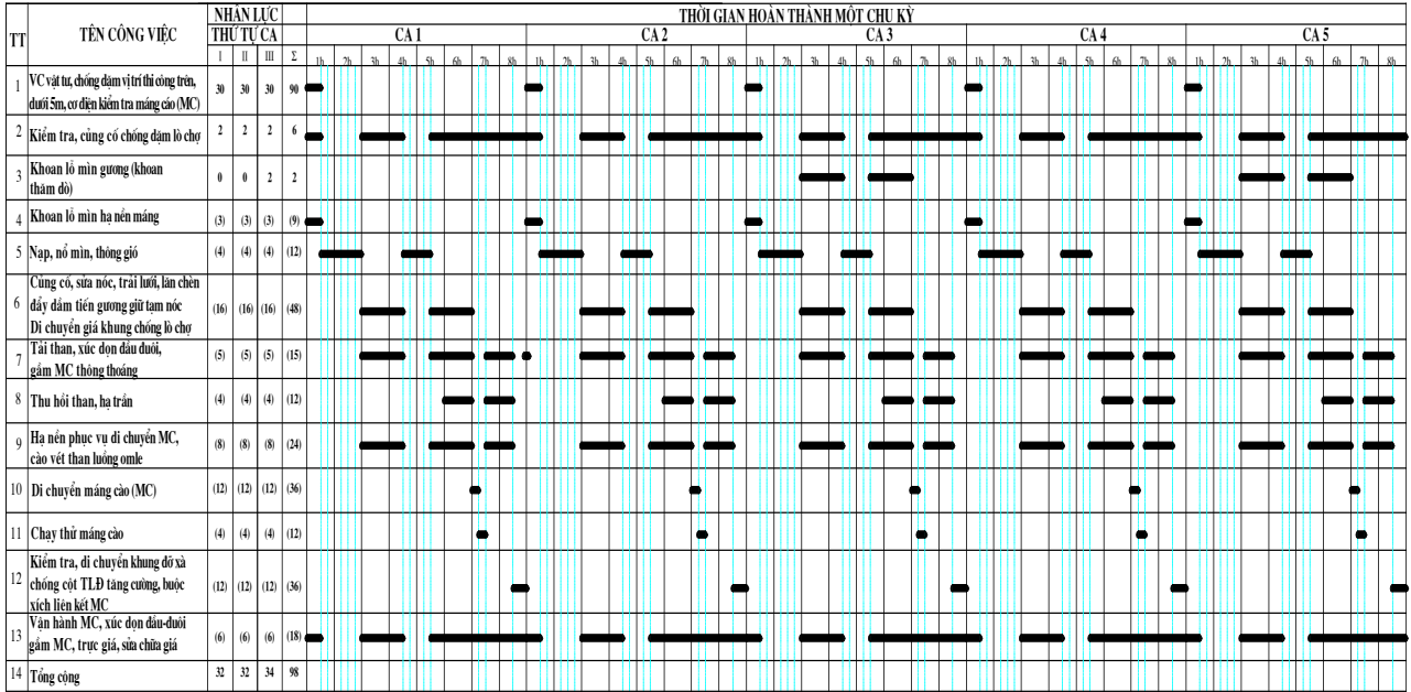
H.5. Biểu đồ bố trí nhân lực để xuất áp dụng cho lò chợ vỉa 10, cánh Bắc của giải pháp
