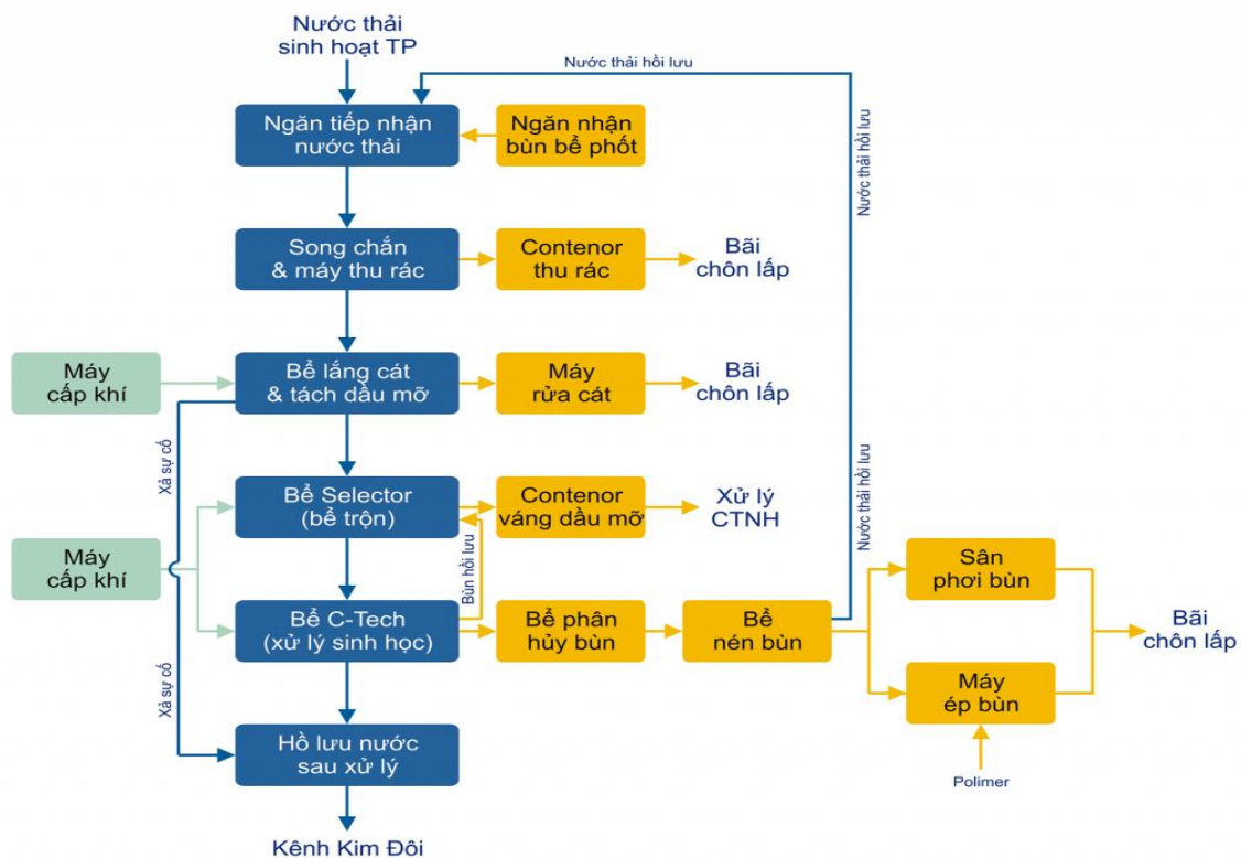
Hình 1. Sơ đồ dây chuyền công nghệ tại NMXLNT thành phố Bắc Ninh ( https://thoatnuocbacninh.vn/ )
