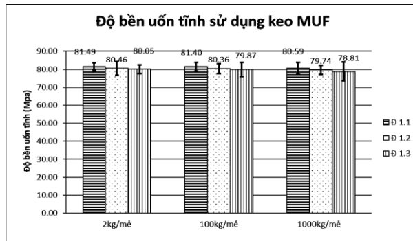
Hình 8. Cường độ uốn tĩnh ván dán gỗ Keo tai tượng sử dụng keo MUF tổng hợp ở 3 quy mô 2 kg/m 2 , 100 kg/m 2 , 1.000 kg/m 2 .
