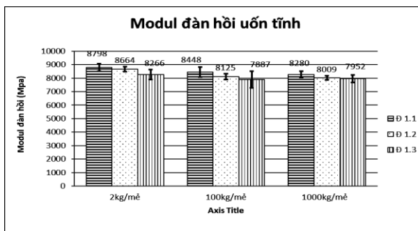
Hình 9. Modul đàn hồi uốn tĩnh ván dán gỗ Keo tai tượng sử dụng keo MUF tổng hợp ở 3 quy mô 2 kg/m 2 , 100 kg/m 2 , 1.000 kg/m 2 .
