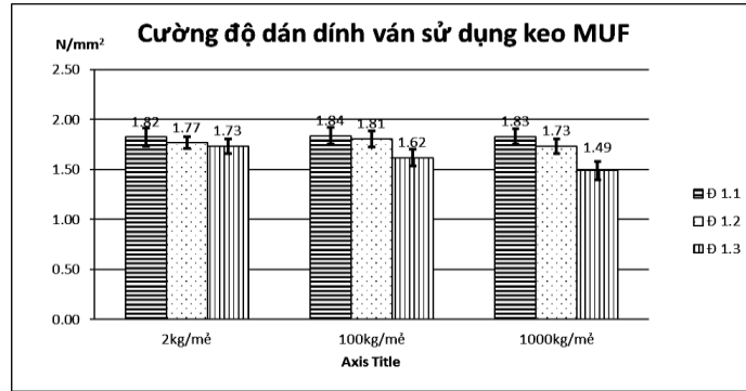
Hình 7. Cường độ kéo trượt Class 2 ván dán gỗ Keo tai tượng sử dụng keo MUF tổng hợp ở 3 quy mô 2 kg/m 2 , 100 kg/m 2 , 1.000 kg/m 2 .
