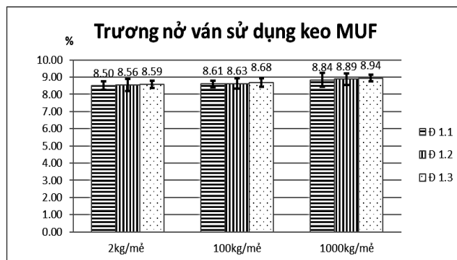
Hình 6. Độ trương nở ván dán gỗ Keo tại tương với 3 đơn keo MUF tổng hợp ở 3 quy mô 2 kg/m 3 , 100 kg/m 3 , 1000 kg/m 3 .
