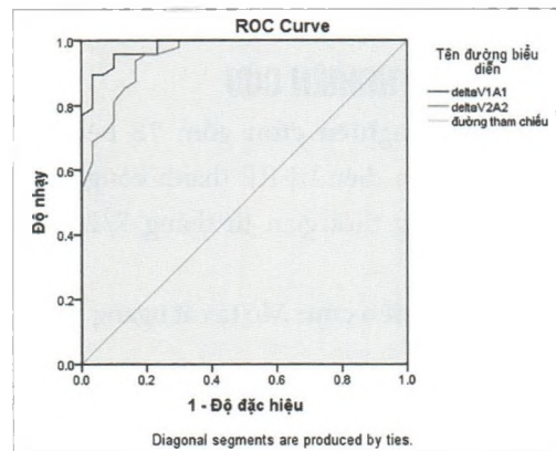
Biểu đồ 1. Đường cong (ROC) của các chỉ số ΔV1A1 và ΔV2A2
