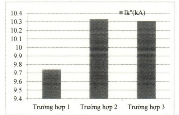
Hình 9. Dòng điện ngắn mạch trong 3 trường hợp
