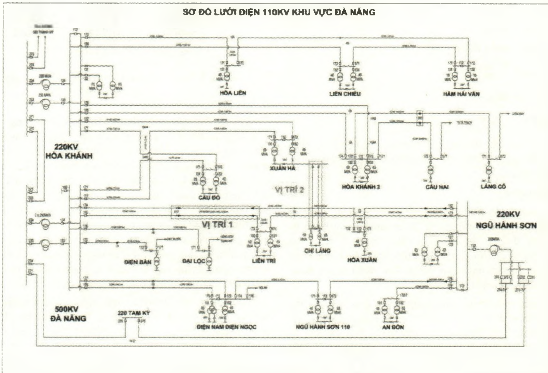
Hình 6. Sơ đồ lưới điện 110kV Đà Nẵng
