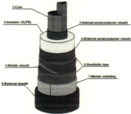
Hình 2. Cấu trúc cáp
