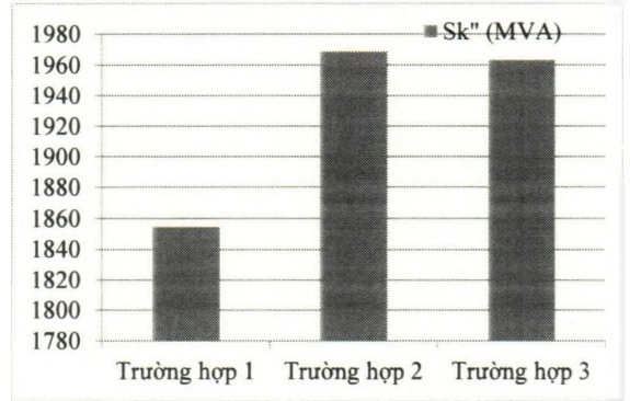
Hình 8. Công suất ngắn mạch trong 3 trường hợp
