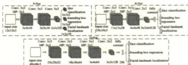
Hình 2. Sơ đồ hoạt động của MTCNN [5]
