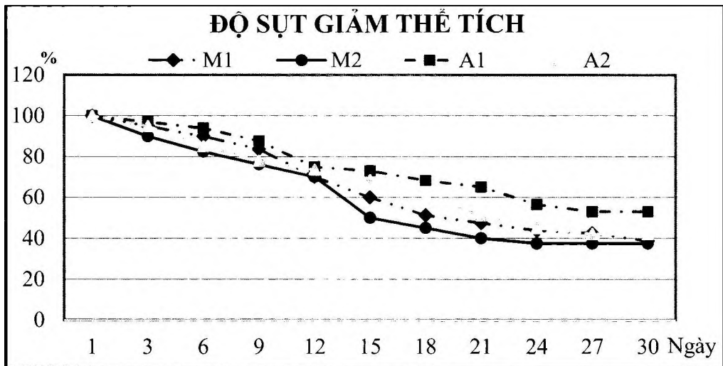
Hình 6. Độ sụt giảm thể tích
