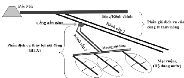
Hình 1. Sơ đồ hệ thống thủy lợi cung cấp dịch vụ cấp nước tưới cho lúa
