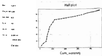
Hình 7. Đồ thị Hall cho 1 giếng bơm ép trên thượng trình
