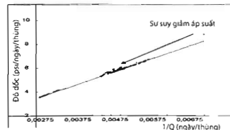
Hình 5. Kết quả khớp lịch sử và dự báo cho giếng bơm ép bằng đá thi Hall
