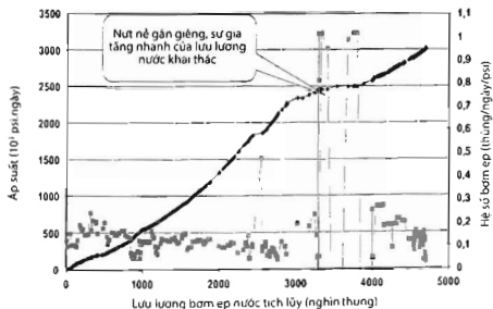
Hình 3. Đồ thị Hall cho giếng bơm ép W-3
