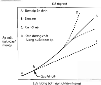
Hình 1. Đồ thị Hall
