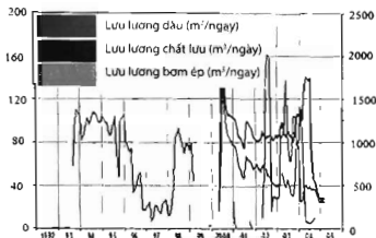
Hình 4. Hiện trạng khai thác giếng 7
