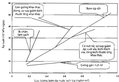
Hình 2. Đồ thị Hall
