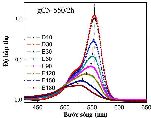
Hình 7. Sự suy giảm nồng độ RhB trong phổ hấp thụ UV-Vis theo thời gian của mẫu g-C_3N_4 nung ở 550 °C trong 2h (Dx nghĩa là khuấy trong bóng tối x phút, Ex nghĩa là chiếu xạ dưới ánh sáng đèn Xenon trong x phút)
