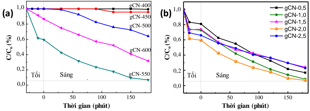
Hình 6. Khả năng quang xúc tác của các mẫu g-C_3N_4 : (a) nhiệt độ nung khác nhau, (b) thời gian nung khác nhau
