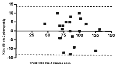
Hình 1. Biểu đồ Bland-Altman.
