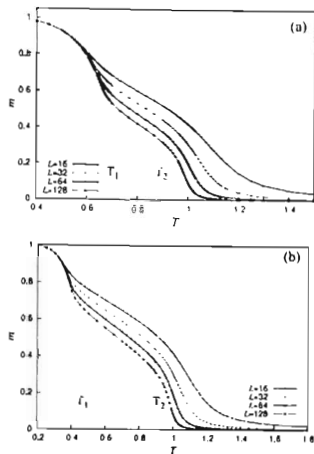
Hình 2. Sự phụ thuộc nhiệt độ của độ từ hoá:
