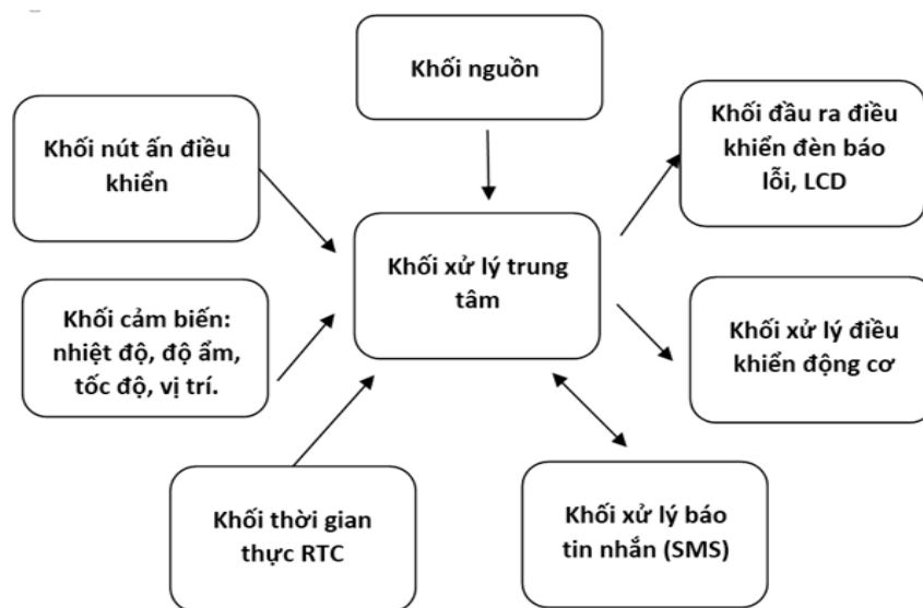
Hình 3. Sơ đồ khối mạch điều khiển.
