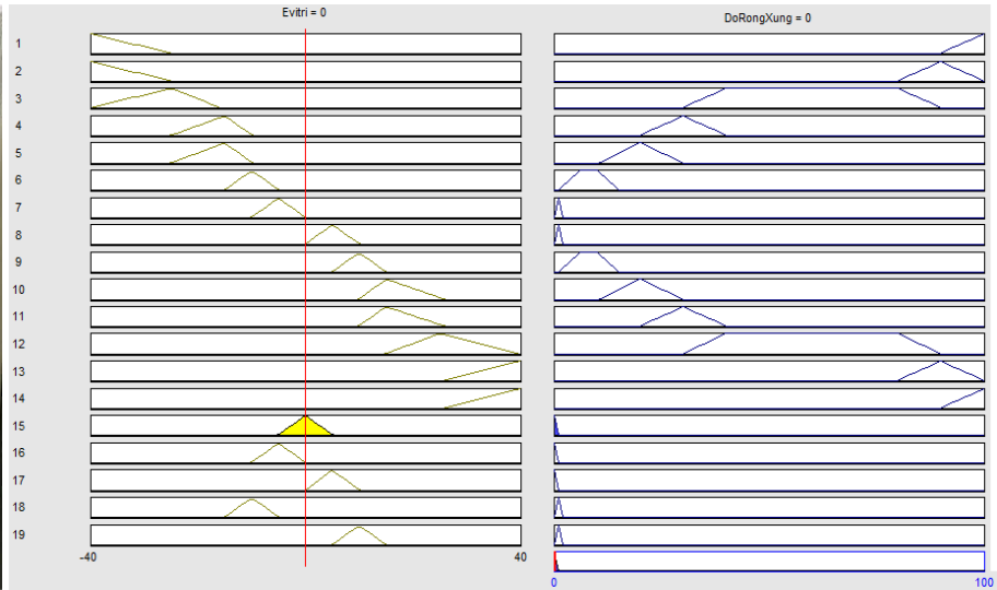
Hình 15. Kết quả mô phỏng bộ điều khiển logic mờ trên phần mềm Matlab.
