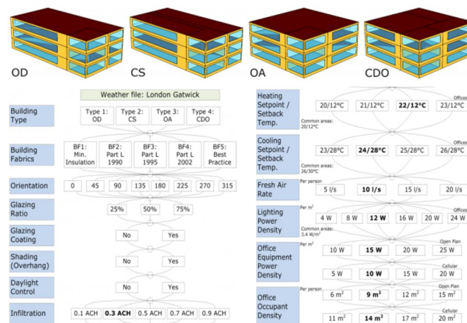
Hình 3. Mô hình công trình và các tham số thiết kế [6]
