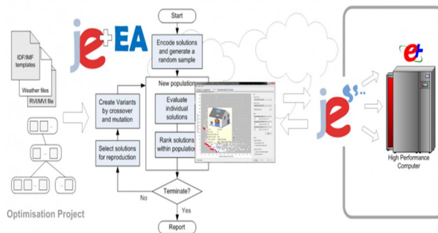
Hình 2. Nguyên lý hoạt động của phần mềm jEPlus+EA (jeplus.org)
