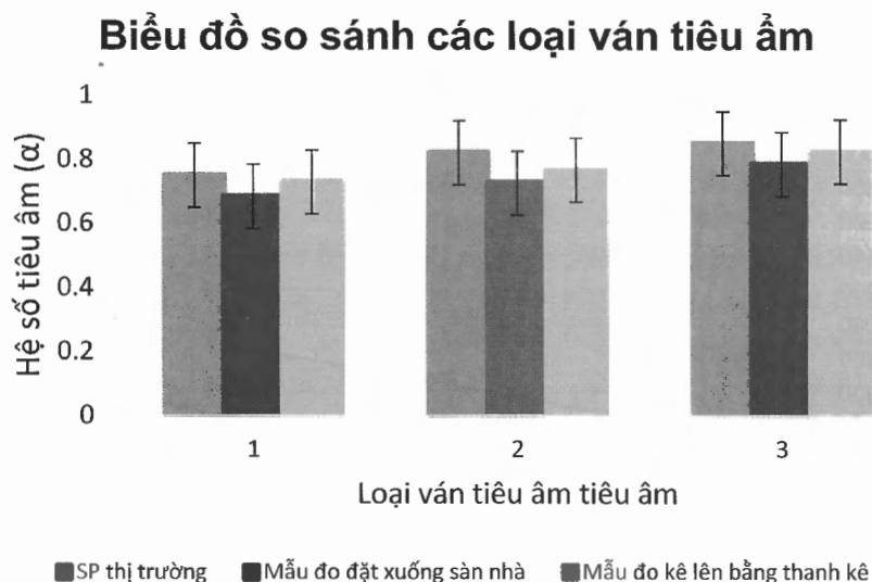
Hình 6. So sánh hệ số tiêu âm của mẫu ván tiêu âm được công bố bởi nhà cung cấp trên thị trường Việt Nam, mẫu ván khi đặt xuống sàn và mẫu ván kê lên thanh kê
