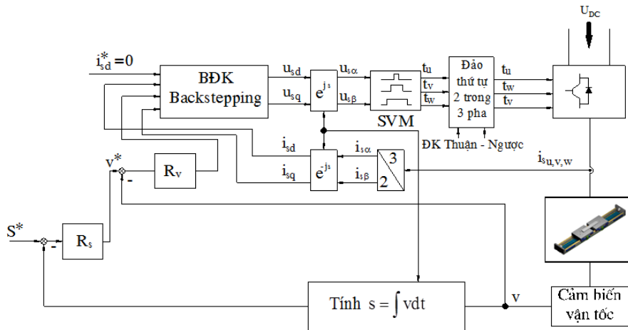
Hình 2. Cấu trúc điều khiển ĐKTĐ-DB-KTVC theo phương pháp Backstepping
