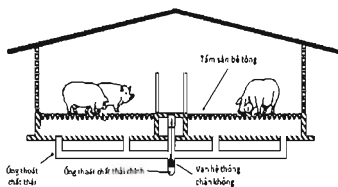
Hình 2. Hệ thống chăn không với nền chuồng hoàn toàn bằng tấm đan
