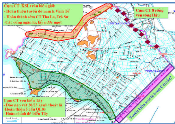
Hình 9: Hệ thống công trình kiểm soát lũ vòng ngoài vùng Tứ Giác Long Xuyên cần điều chỉnh nâng cấp
