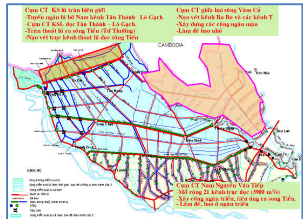
Hình 10: Hệ thống công trình kiểm soát lũ vòng ngoài vùng Đồng Tháp Mười cần điều chỉnh nâng cấp
