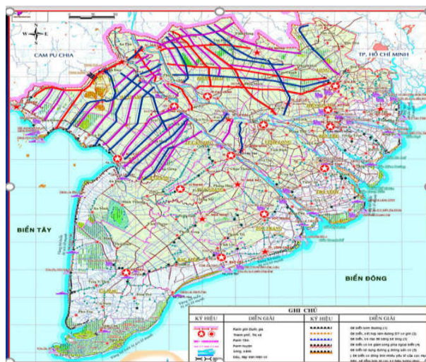
Hình 2: Một số hạng mục công trình chính kiểm soát lũ tràn biên giới, hệ thống kênh trục vùng lũ ĐBSCL
