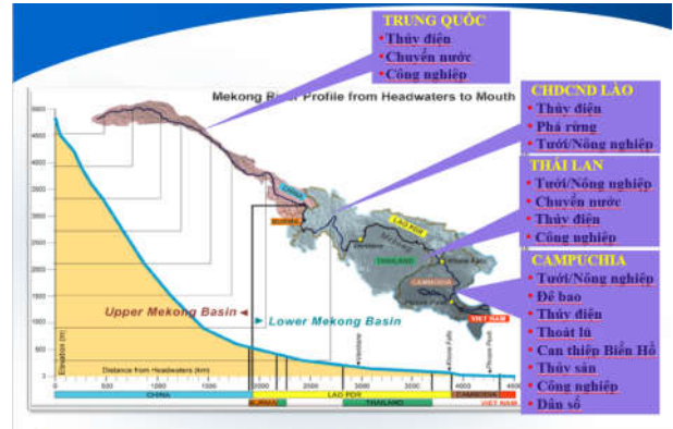
Hình 5: Một số hoạt động của các nước thượng châu thổ sông Mê Công làm thay đổi chế độ động lực, bùn cát vùng ĐBSCL
