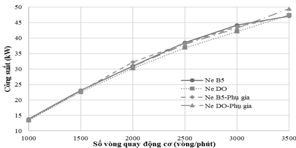
Hình 2. Kết quả đo công suất động cơ
