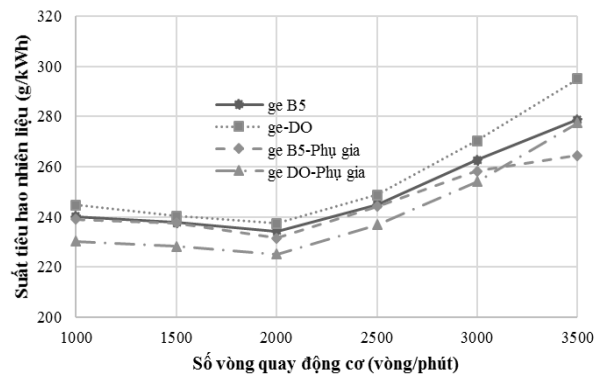
Hình 3. Kết quả đo tiêu hao nhiên liệu
