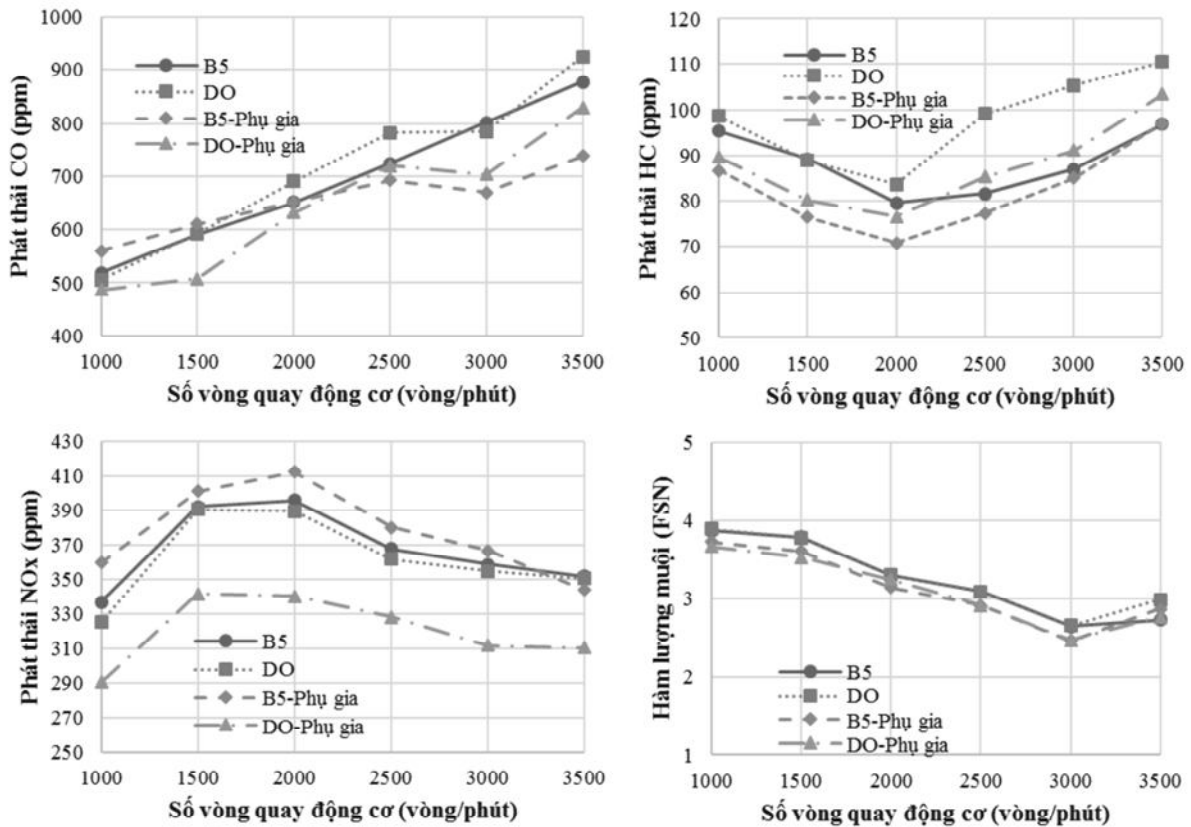
Hình 4. Kết quả đo phát thải CO, HC, NO x và độ khói
