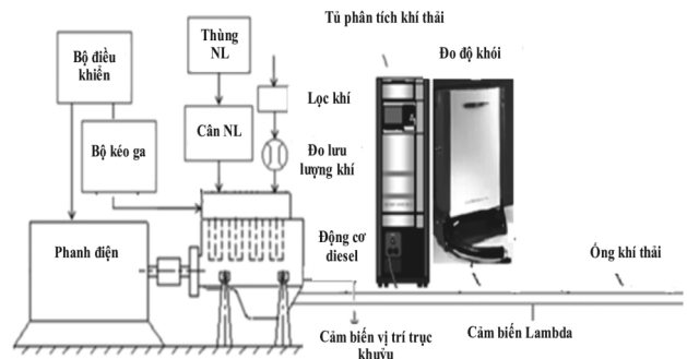
Hình 1. Sơ đồ băng thử động cơ
